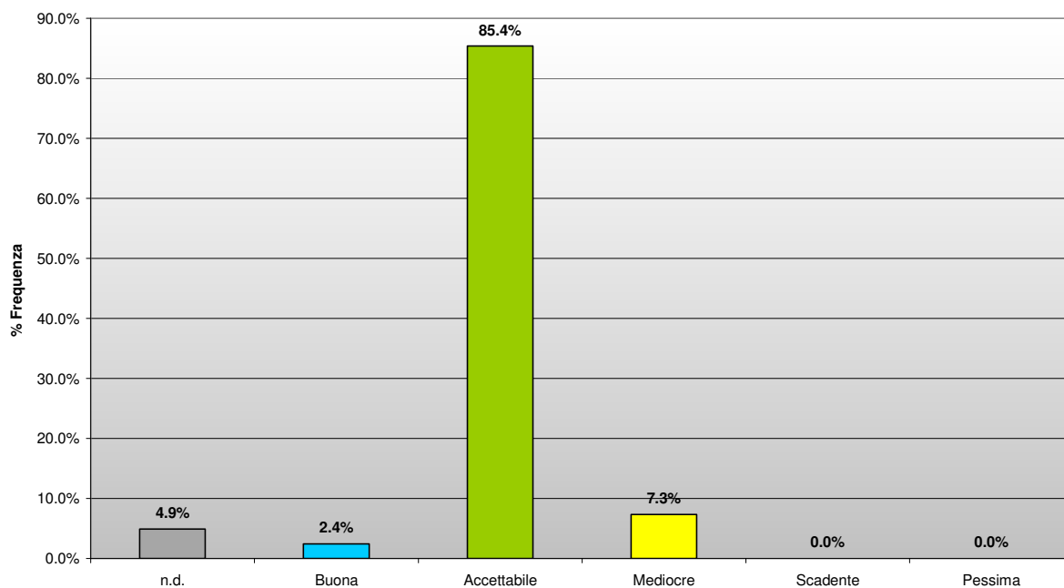
Indice di qualità dell'aria - Campagna di BL-Soverzene
