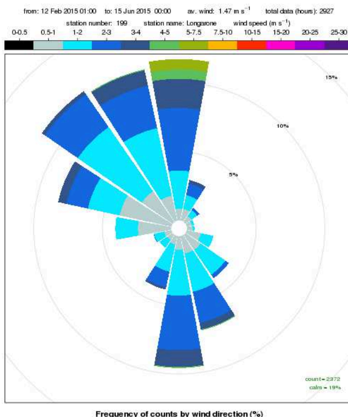
Figura 4: rosa dei venti registrati presso la stazione meteorologica di Longarone nel periodo 12 febbraio – 15 giugno 2015
