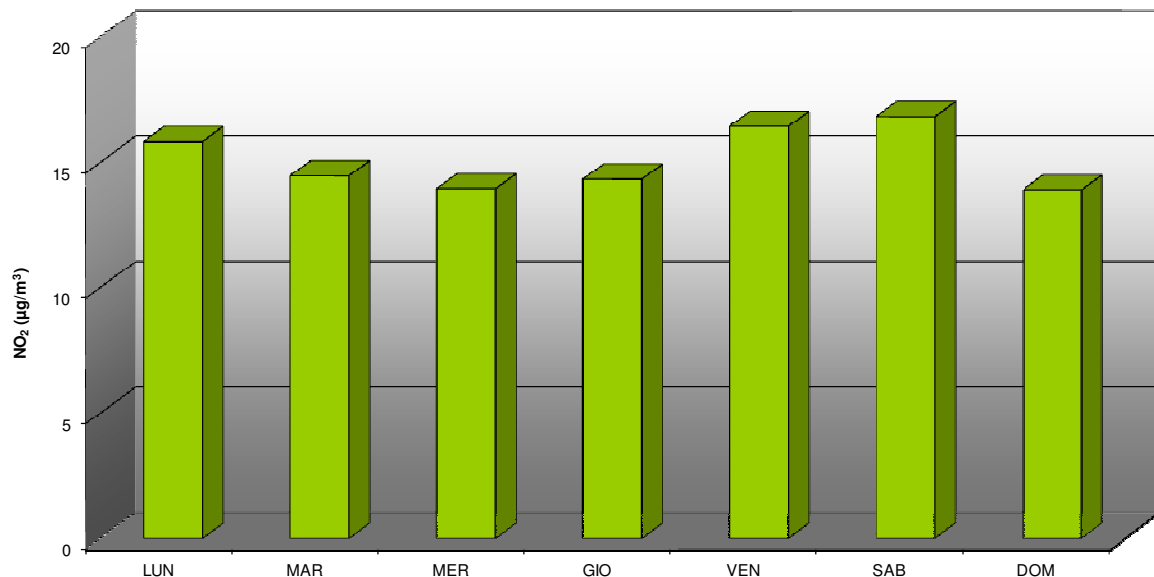
COMUNE DI SOVERZENE: PARAMETRO BISSIDO DI AZOTO (NO 2 ) SETTIMANATIPO DAL 12 FEBBRAIO AL 14 GIUGNO 2015
