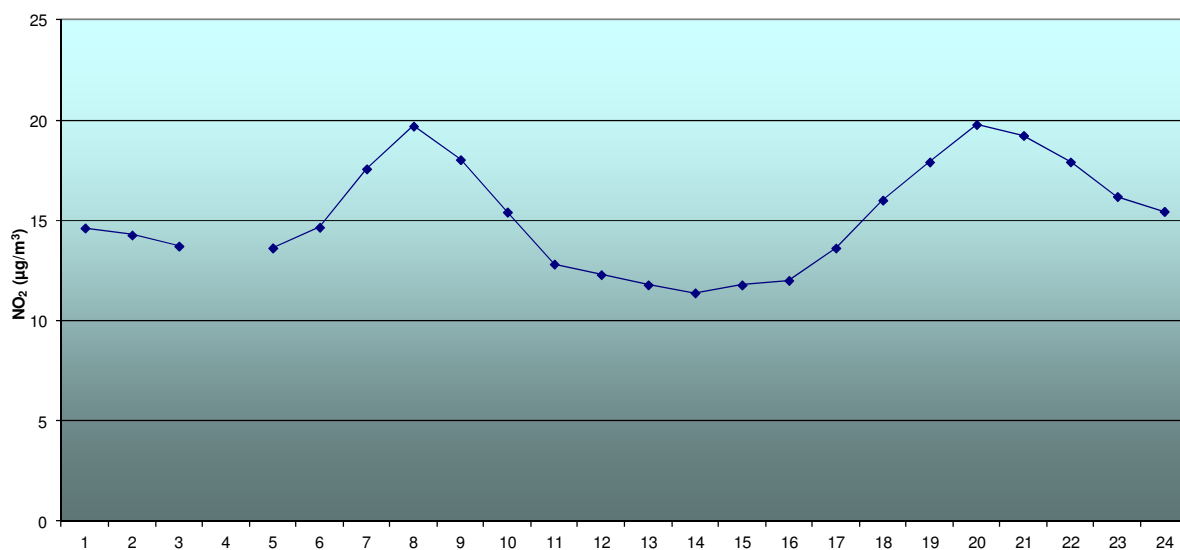
COMUNE DI SOVERZENE: PARAMETRO BLOSSIDO DI AZOTO (NO 2 ) GIORNO TIPO DAL 12 FEBBRAIO AL 14 GIUGNO 2015
