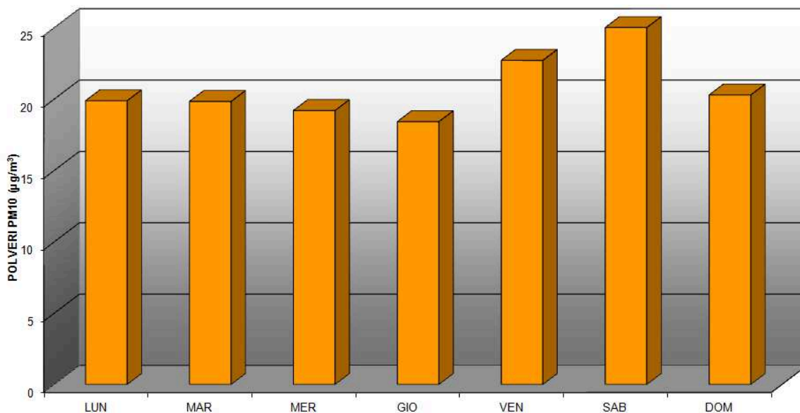
COMUNE DI SOVERZENE: PARAMETRO POLVERI PM10 SETTIMANA TIPO DAL 12 FEBBRAIO AL 14 GIUGNO 2015
