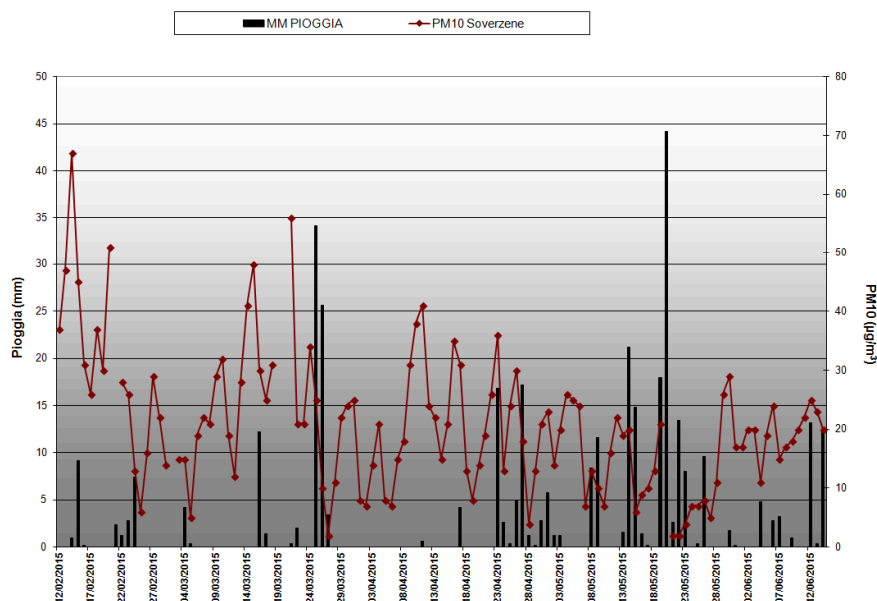
COMUNE DI SOVERZENE ANDAMENTO DELLE POLVERI PM10 DAL 12 FEBBRAIO AL 14 GIUGNO 2015
