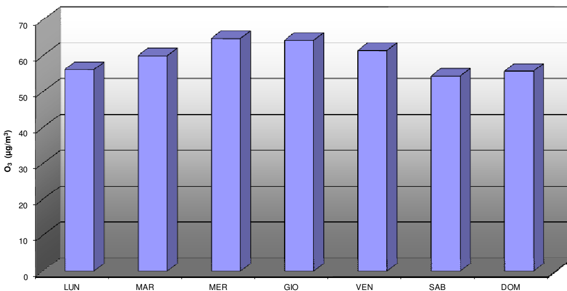
COMUNE DI SOVERZENE: PARAMETRO OZONO (O 3 ) SETTIMANA TIPO DAL 12 FEBBRAIO AL 14 GIUGNO 2015
