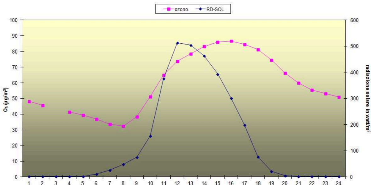
COMUNE DI SOVERZENE: GIORNO TIPO OZONO (O 3 ) E RADIAZIONE SOLARE DAL 12 FEBBRAIO AL 14 GIUGNO 2015
