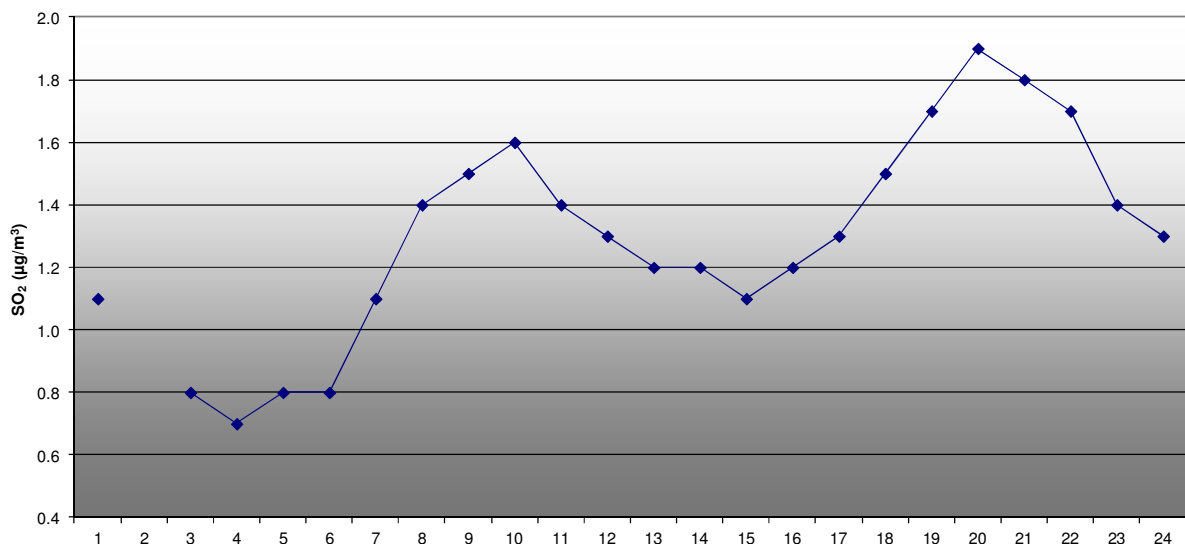
COMUNE DI SOVERZENE: PARAMETRO ANIDRIDE SOLFOROSA (SO 2 ) GIORNO TIPO DAL 12 FEBBRAIO AL 14 GIUGNO 2015
