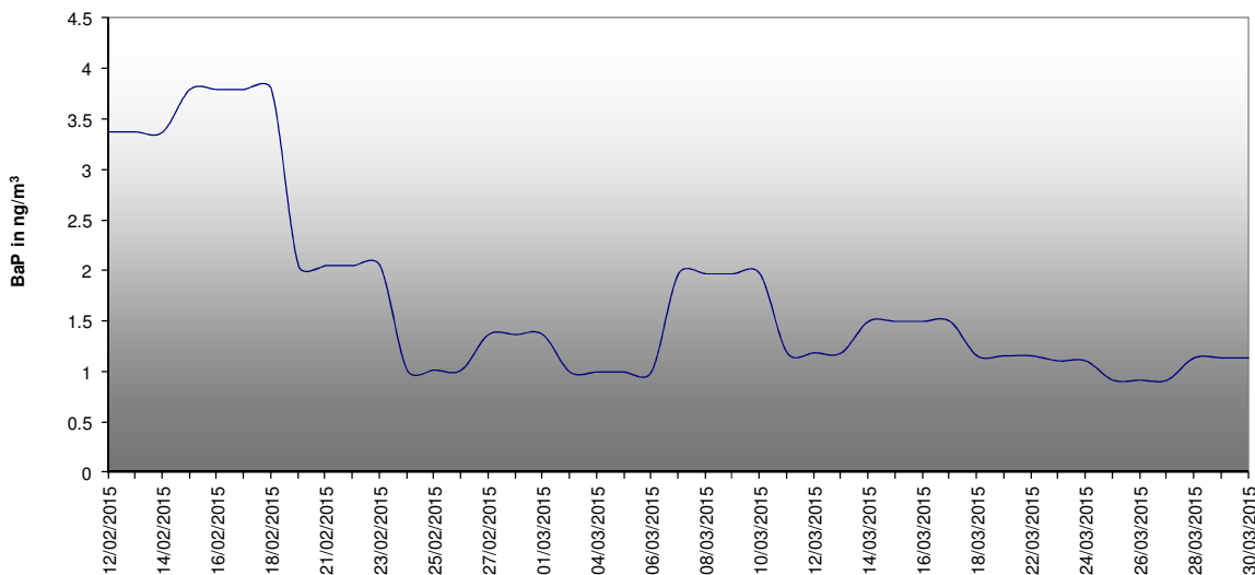
Comune di Soverzene: misure giornaliere di Benzo(a)Pirene dal 12 febbraio al 30 marzo 2015
