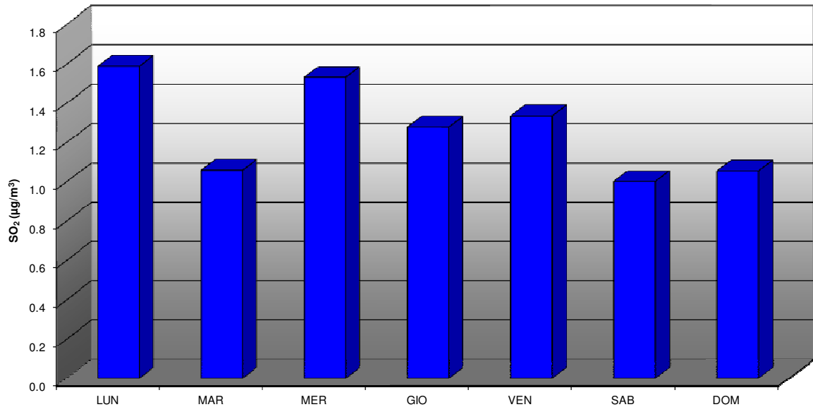
COMUNE DI SOVERZENE: PARAMETRO ANIDRIDE SOLFOROSA (SO 2 ) SETTIMANATIPO DAL 12 FEBBRAIO AL 14 GIUGNO 2015
