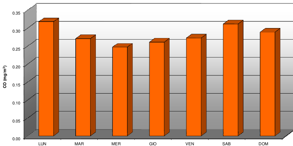
COMUNE DI SOVERZENE: PARAMETRO MONOSSIDO DI CARBONIO (CO) SETTIMANATIPO DAL 12 FEBBRAIO AL 14 GIUGNO 2015
