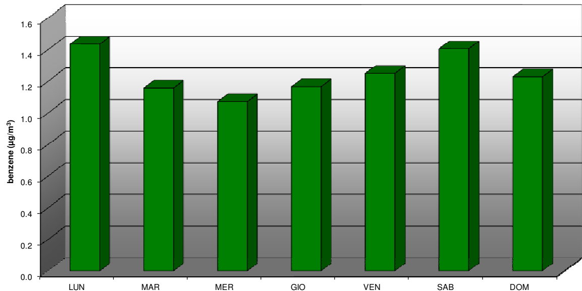
COMUNE DI SOVERZENE: PARAMETRO BENZENE (C 6 H 6 ) SETTIMANATIPO DAL 12 FEBBRAIO AL 14 GIUGNO 2015
