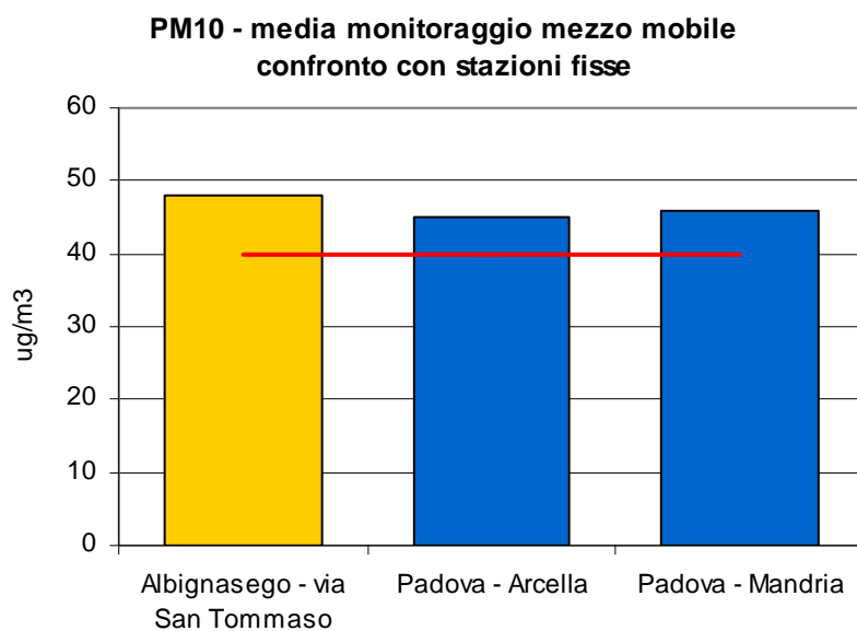
Figura 2.2 Polveri fini ( \text{PM}_{10} ): concentrazione media durante il monitoraggio dal 16/02/12 al 27/03/12 e dal 20/06/12 al 24/07/12 nel Comune di Albignasego.
