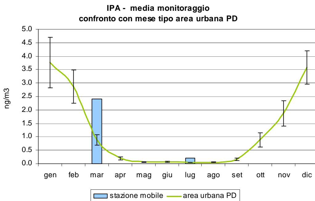
Figura 3.4 Benzo(a)pirene (IPA): confronto delle concentrazioni medie rilevate durante il monitoraggio nel Comune di Albignasego, con l'andamento caratteristico del 'mese tipo' ricavato dalla serie storica nell'area urbana di Padova. Le barre di errore indicano un intervallo \pm 2\sigma intorno alla media del mese tipo.
