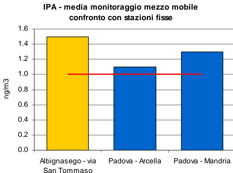
Figura 2.3 Benzo(a)pirene (IPA): concentrazione media rilevata durante il monitoraggio dal 16/02/12 al 27/03/12 e dal 20/06/12 al 24/07/12 nel Comune di Albignasego.
