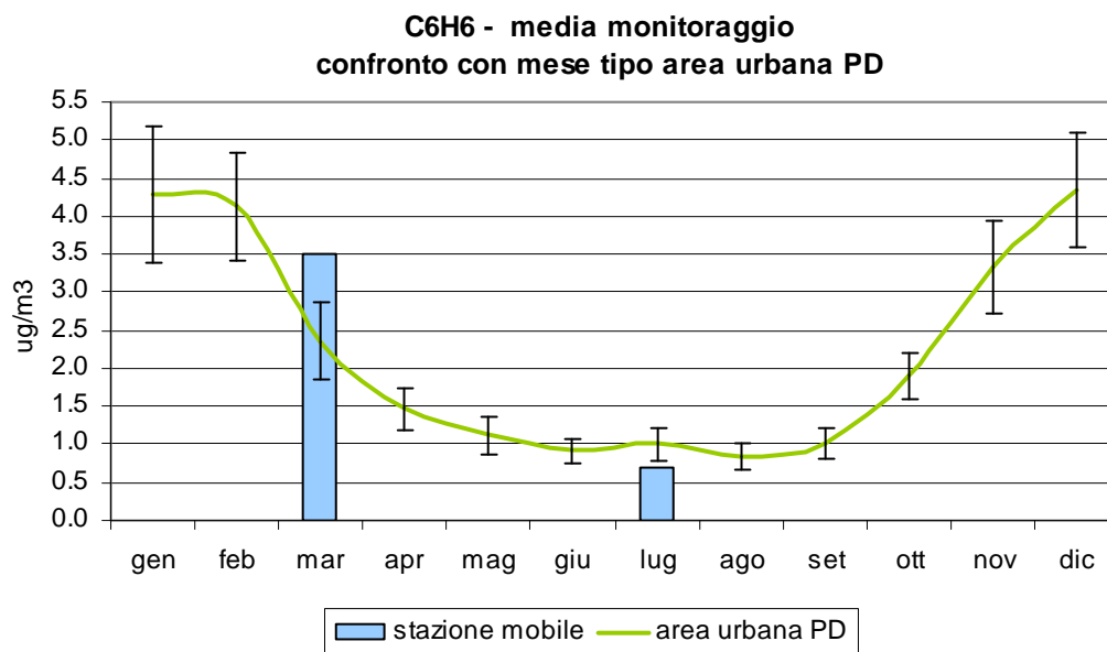
Figura 3.5 Benzene (C 6 H 6 ): confronto delle concentrazioni medie rilevate durante il monitoraggio nel Comune di Albignasego, con l'andamento caratteristico del 'mese tipo' ricavato dalla serie storica nell'area urbana di Padova. Le barre di errore indicano un intervallo \pm 2\sigma intorno alla media del mese tipo.
