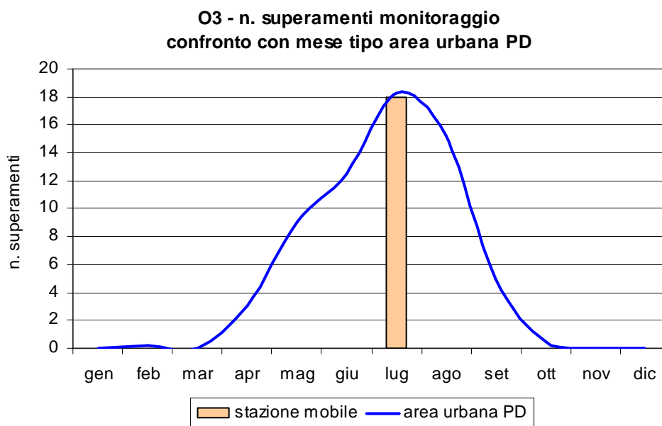
Figura 3.1 Ozono ( O_3 ): confronto del numero di superamenti del valore del limite di protezione della salute ( 120 \mu\text{g}/\text{m}^3 ) rilevati durante il monitoraggio nel Comune di Albignasego, con l'andamento caratteristico del 'mese tipo' ricavato dai dati della serie storica della stazione fissa di Mandria.
