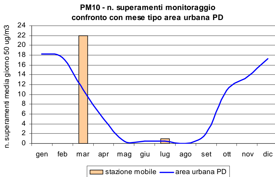
Figura 3.3 Polveri fini (PM 10 ): confronto delle concentrazioni medie e del numero di superamenti del valore limite di protezione della salute (50 µg/m 3 ) rilevati durante il monitoraggio nel Comune di Albignasego, con l'andamento caratteristico del 'mese tipo' ricavato dalla serie storica nell'area urbana di Padova.
