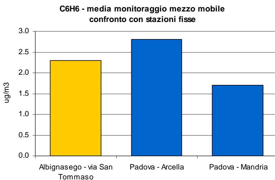
Figura 2.4 Benzene ( \text{C}_6\text{H}_6 ): concentrazione media rilevata durante il monitoraggio in Via Don Schiavon nel Comune di Albignasego.
