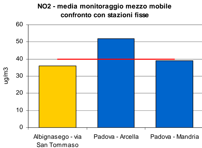
Figura 2.1 Biossido di azoto (NO 2 ): concentrazione media rilevata durante il monitoraggio nel Comune di Albignasego.
