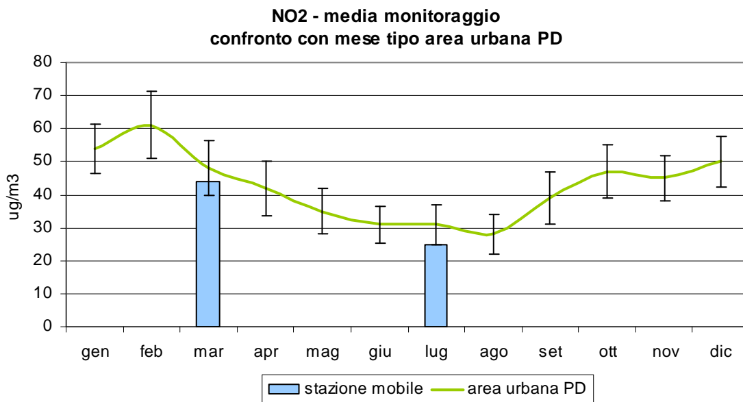
Figura 3.2 Biossido di azoto (NO 2 ): confronto delle concentrazioni medie rilevate durante il monitoraggio nel Comune di Albignasego, con l'andamento caratteristico del 'mese tipo' ricavato dalla serie storica nell'area urbana di Padova. Le barre di errore indicano un intervallo \pm 2\sigma intorno alla media del mese tipo.
