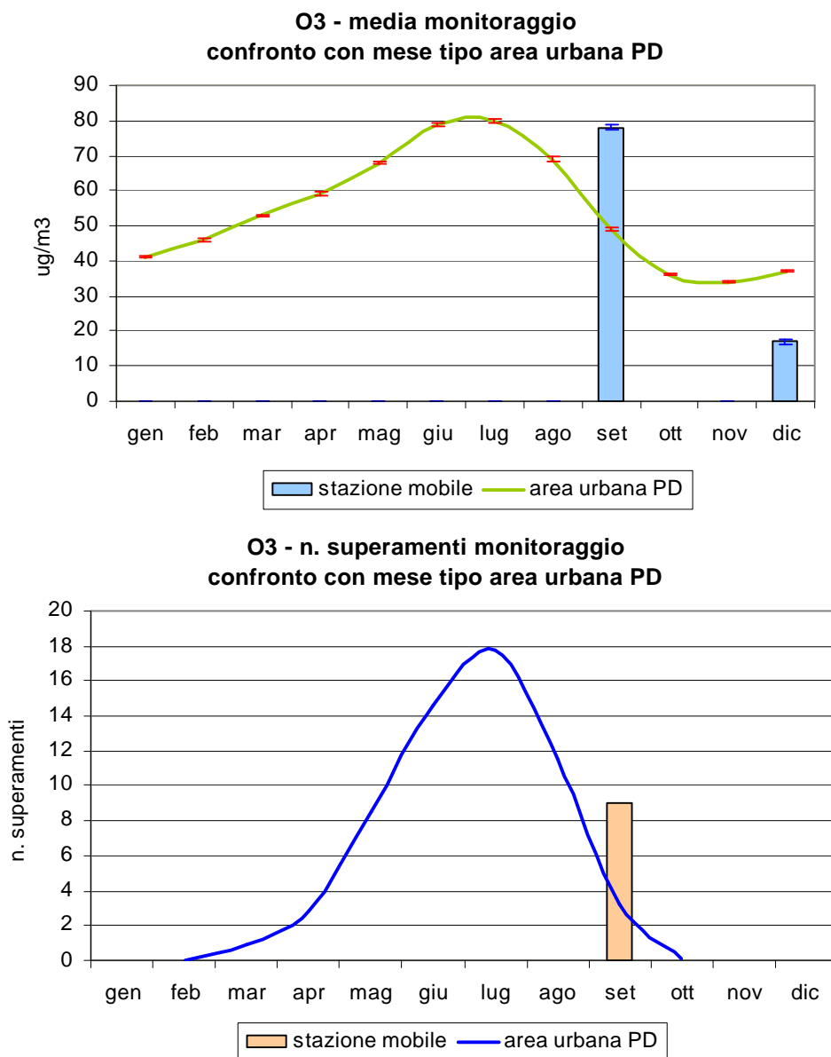
Figura 3.4 Ozono (O 3 ): confronto delle concentrazioni medie e del numero di superamenti del valore del limite di protezione della salute (120 \mu\text{g}/\text{m}^3 ) rilevati durante il monitoraggio in Via Ulivi nel Comune di Arquà Petrarca, con l'andamento caratteristico del 'mese tipo' ricavato dalla serie storica nell'area urbana di Padova (dai dati della serie storica della sola stazione fissa di Mandria); per i valori di concentrazione mensile le barre indicano l'errore standard della media.
