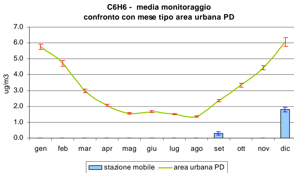
Figura 3.7 Benzene ( C_6H_6 ): confronto delle concentrazioni medie rilevate durante il monitoraggio in Via Ulivi nel Comune di Arquà Petrarca, con l'andamento caratteristico del 'mese tipo' ricavato dalla serie storica nell'area urbana di Padova; le barre indicano l'errore standard della media.
