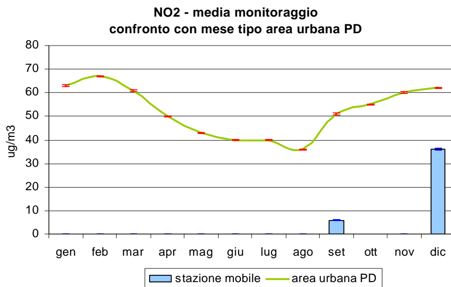
Figura 3.3 Biossido di azoto (NO 2 ): confronto delle concentrazioni medie rilevate durante il monitoraggio in Via Ulivi nel Comune di Arquà Petrarca, con l'andamento caratteristico del 'mese tipo' ricavato dalla serie storica nell'area urbana di Padova; le barre indicano l'errore standard della media.
