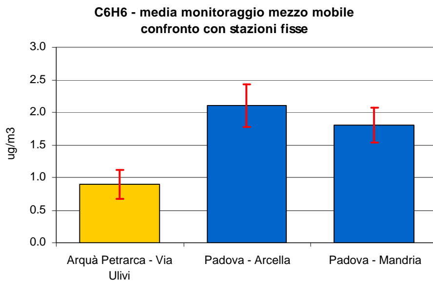
Figura 2.7 Benzene (C 6 H 6 ): concentrazione media rilevata durante il monitoraggio in Via Ulivi nel Comune di Arquà Petrarca; le barre indicano l'errore standard della media.
