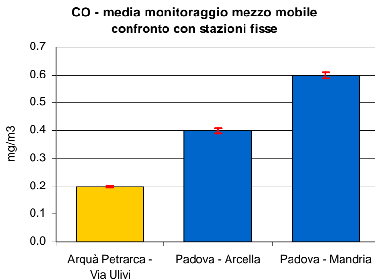
Figura 2.2 Monossido di carbonio (CO): concentrazione media rilevata durante il monitoraggio in Via Ulivi nel Comune di Arquà Petrarca; le barre indicano l'errore standard della media.
