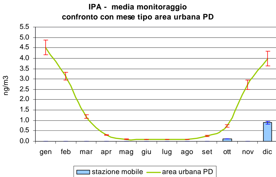
Figura 3.6 Benzo(a)pirene (IPA): confronto delle concentrazioni medie rilevate durante il monitoraggio in Via Ulivi nel Comune di Arquà Petrarca, con l'andamento caratteristico del 'mese tipo' ricavato dalla serie storica nell'area urbana di Padova; le barre indicano l'errore standard della media.
