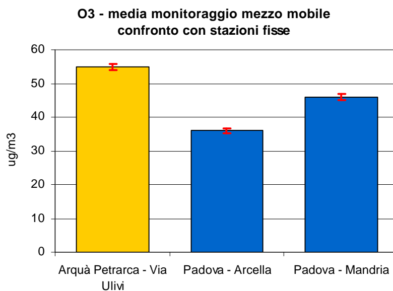
Figura 2.3 Ozono ( O_3 ): concentrazione media rilevata durante il monitoraggio in Via Ulivi nel Comune di Arquà Petrarca; le barre indicano l'errore standard della media.
