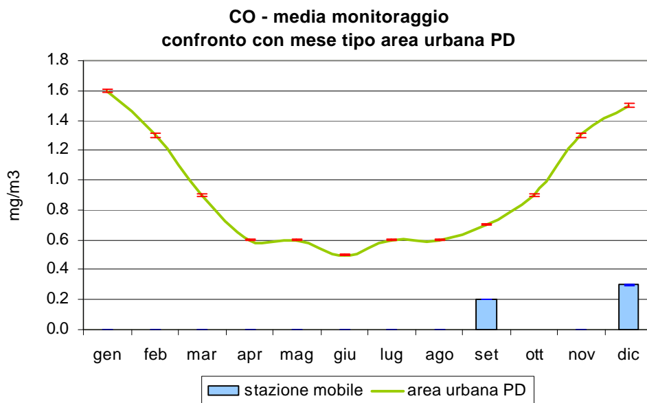
Figura 3.2 Monossido di carbonio (CO): confronto delle concentrazioni medie rilevate durante il monitoraggio in Via Ulivi nel Comune di Arquà Petrarca, con l'andamento caratteristico del 'mese tipo' ricavato dalla serie storica nell'area urbana di Padova; le barre indicano l'errore standard della media.
