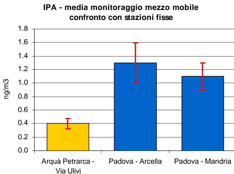
Figura 2.6 Benzo(a)pirene (IPA): concentrazione media rilevata durante il monitoraggio dal 21/08/09 al 12/10/09 e dal 18/11/09 al 20/12/09 in Via Ulivi nel Comune di Arquà Petrarca; le barre indicano l'errore standard della media.
