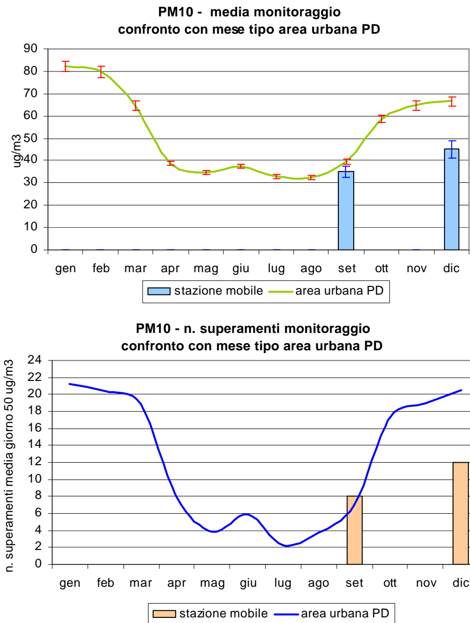
Figura 3.5 Polveri fini (PM 10 ): confronto delle concentrazioni medie e del numero di superamenti del valore limite di protezione della salute (50 \mu\text{g}/\text{m}^3 ) rilevati durante il monitoraggio in Via Ulivi nel Comune di Arquà Petrarca, con l'andamento caratteristico del 'mese tipo' ricavato dalla serie storica nell'area urbana di Padova; per i valori di concentrazione mensile le barre indicano l'errore standard della media.
