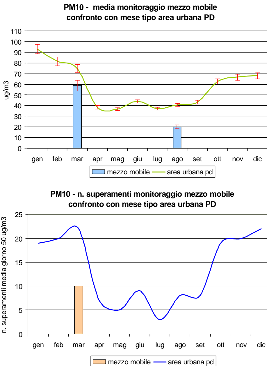
Figura 2.5 Polveri fini ( PM_{10} ): concentrazione media e numero di superamenti rilevati durante il monitoraggio dal 10/03/05 al 30/03/05 e dal 03/08/05 al 31/08/05 in Via Matteotti nel Comune di Bagnoli di Sopra; confronto con i periodi corrispondenti presso le stazioni fisse di Arcella e Mandria nel Comune di Padova e con l'andamento caratteristico del 'mese tipo' ricavato dalla serie storica nell'area urbana di Padova; per i valori di concentrazione mensile le barre indicano l'errore standard della media.
