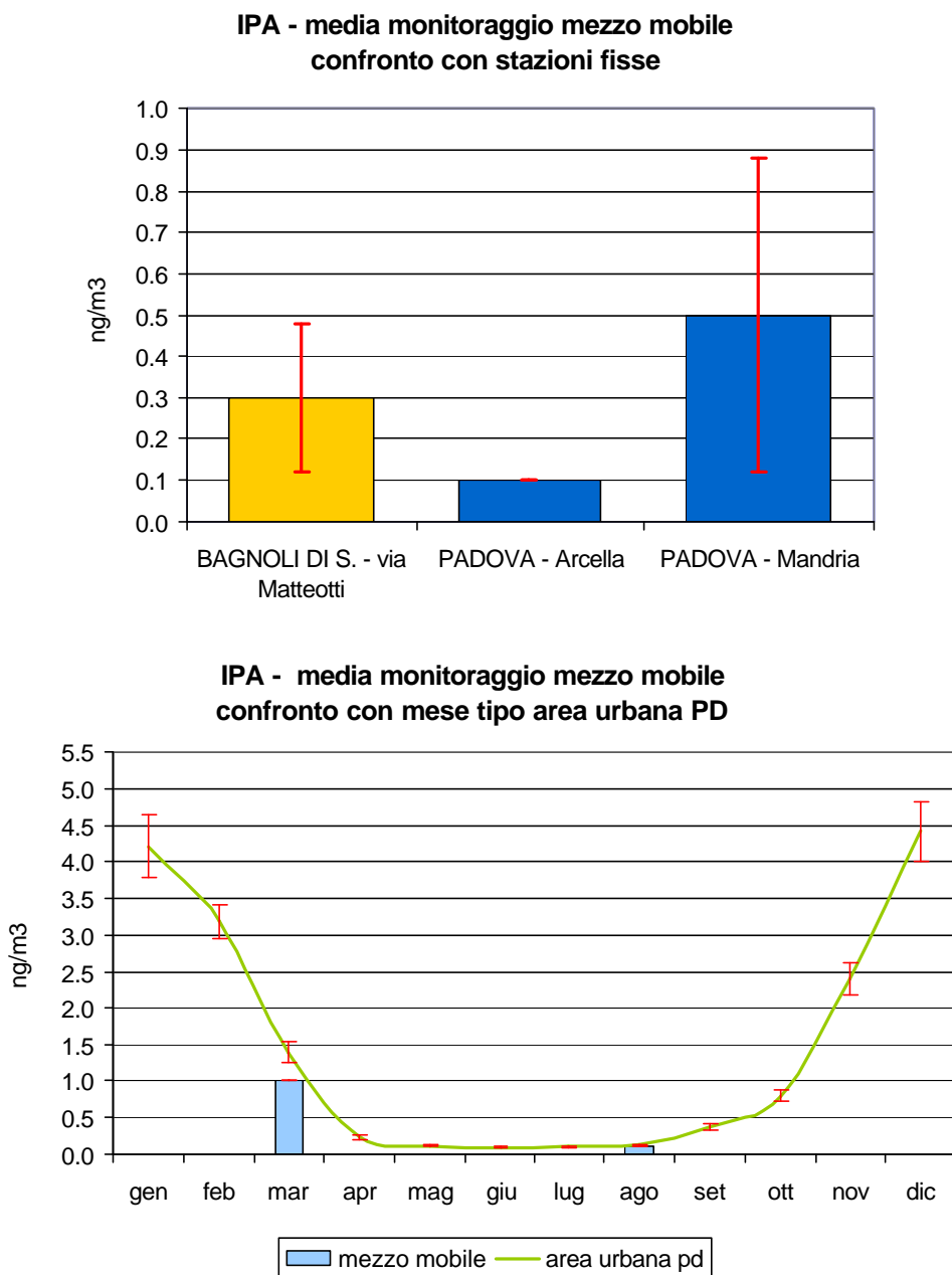
Figura 2.6 Benzo(a)pirene (IPA): concentrazione media rilevata durante il monitoraggio dal 10/03/05 al 30/03/05 e dal 03/08/05 al 31/08/05 in Via Matteotti nel Comune di Bagnoli di Sopra; confronto con i periodi corrispondenti presso le stazioni fisse di Arcella e Mandria nel Comune di Padova e con l'andamento caratteristico del 'mese tipo' ricavato dalla serie storica nell'area urbana di Padova; le barre indicano l'errore standard della media.
