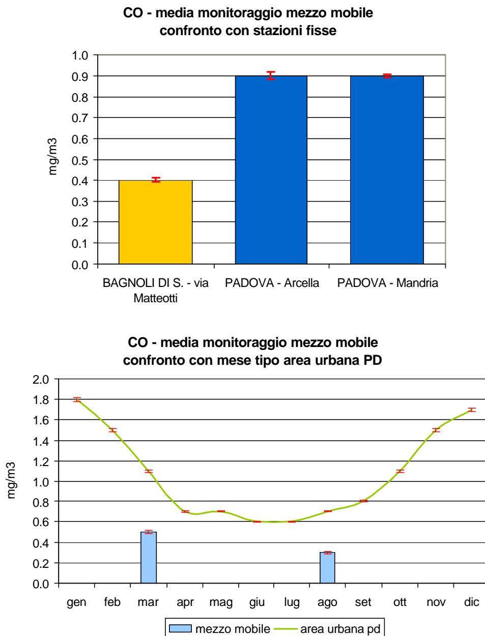
Figura 2.2 Monossido di carbonio (CO): concentrazione media rilevata durante il monitoraggio dal 10/03/05 al 30/03/05 e dal 03/08/05 al 31/08/05 in Via Matteotti nel Comune di Bagnoli di Sopra; confronto con i periodi corrispondenti presso le stazioni fisse di Arcella e Mandria nel Comune di Padova e con l'andamento caratteristico del 'mese tipo' ricavato dalla serie storica nell'area urbana di Padova; le barre indicano l'errore standard della media.
