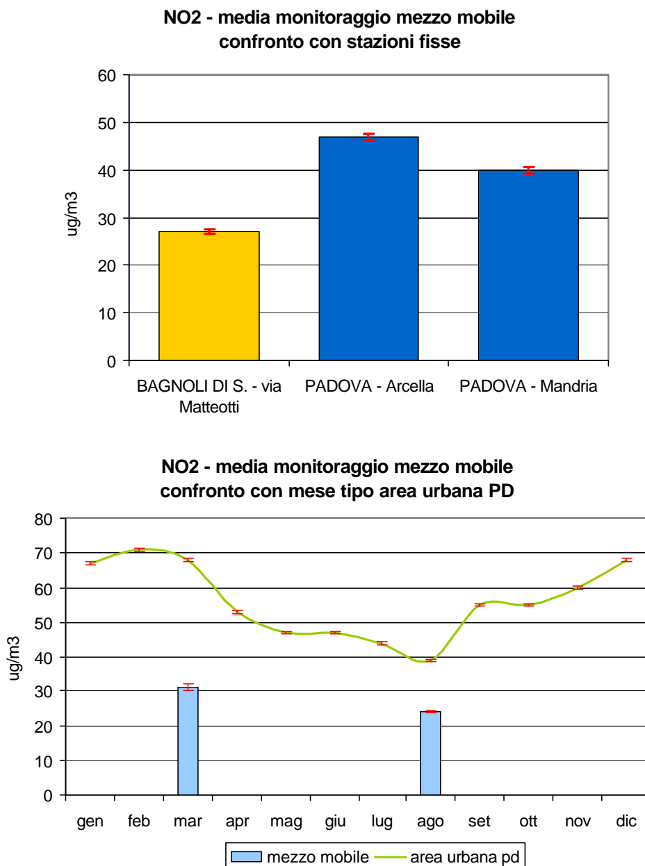
Figura 2.4 Biossido di azoto (NO 2 ): concentrazione media rilevata durante il monitoraggio dal 10/03/05 al 30/03/05 e dal 03/08/05 al 31/08/05 in Via Matteotti nel Comune di Bagnoli di Sopra; confronto con i periodi corrispondenti presso le stazioni fisse di Arcella e Mandria nel Comune di Padova e con l'andamento caratteristico del 'mese tipo' ricavato dalla serie storica nell'area urbana di Padova; le barre indicano l'errore standard della media.
