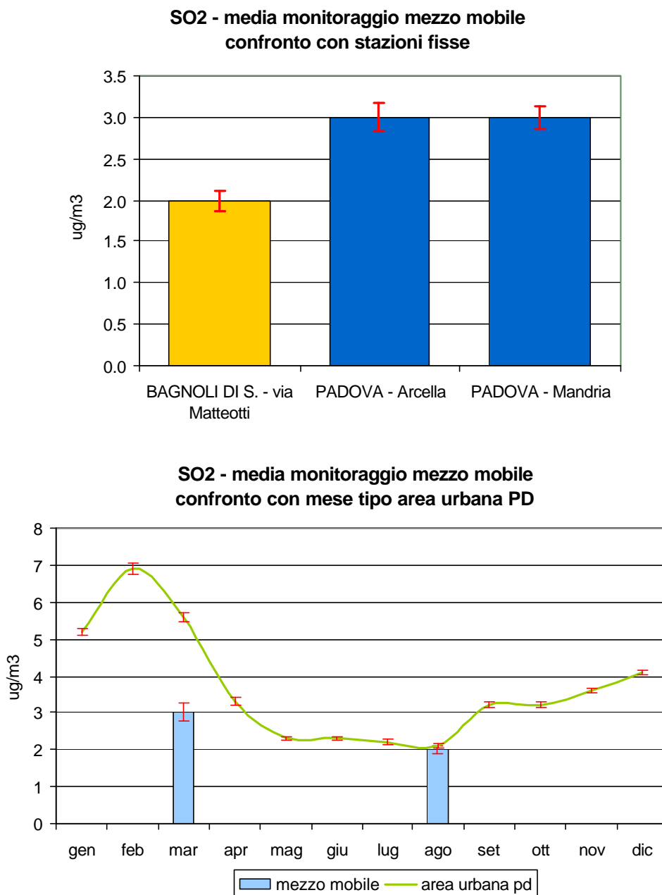
Figura 2.1 Biossido di zolfo (SO 2 ): concentrazione media rilevata durante il monitoraggio dal 10/03/05 al 30/03/05 e dal 03/08/05 al 31/08/05 in Via Matteotti nel Comune di Bagnoli di Sopra; confronto con i periodi corrispondenti presso la stazione fissa di Arcella e di Mandria nel Comune di Padova e con l'andamento caratteristico del 'mese tipo' ricavato dalla serie storica nell'area urbana di Padova; le barre indicano l'errore standard della media.
