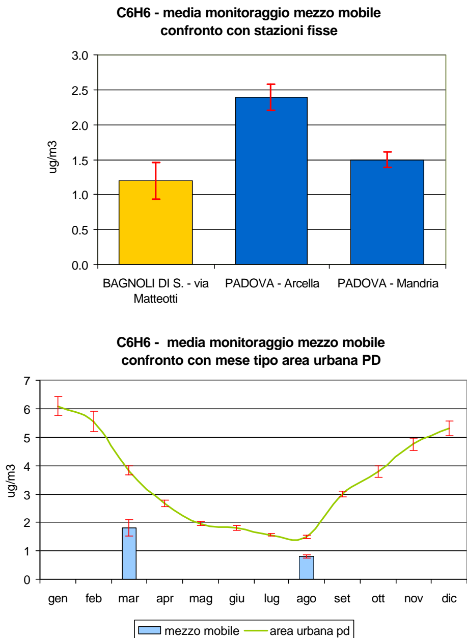
Figura 2.7 Benzene ( C_6H_6 ): concentrazione media rilevata durante il monitoraggio dal 10/03/05 al 30/03/05 e dal 03/08/05 al 31/08/05 in Via Matteotti nel Comune di Bagnoli di Sopra; confronto con i periodi corrispondenti presso le stazioni fisse di Arcella e Mandria nel Comune di Padova e con l'andamento caratteristico del 'mese tipo' ricavato dalla serie storica nell'area urbana di Padova; le barre indicano l'errore standard della media.
