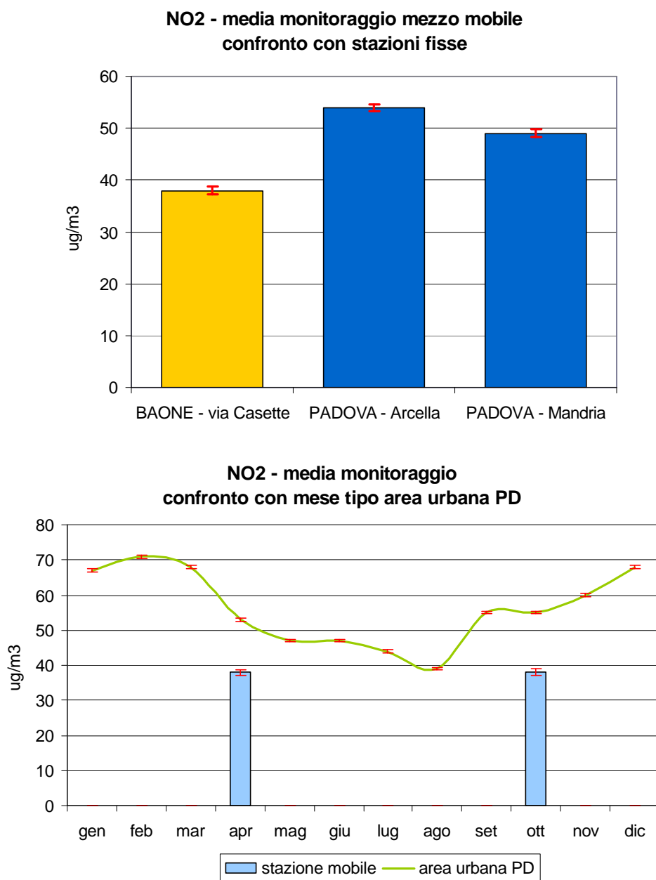
Figura 2.4 Biossido di azoto (NO 2 ): concentrazione media rilevata durante il monitoraggio dal 28/09/05 al 20/10/05 e dal 22/03/06 al 06/04/06 in Via Casette nel Comune di Baone; confronto con i periodi corrispondenti presso le stazioni fisse di Arcella e Mandria nel Comune di Padova e con l'andamento caratteristico del 'mese tipo' ricavato dalla serie storica nell'area urbana di Padova; le barre indicano l'errore standard della media.
