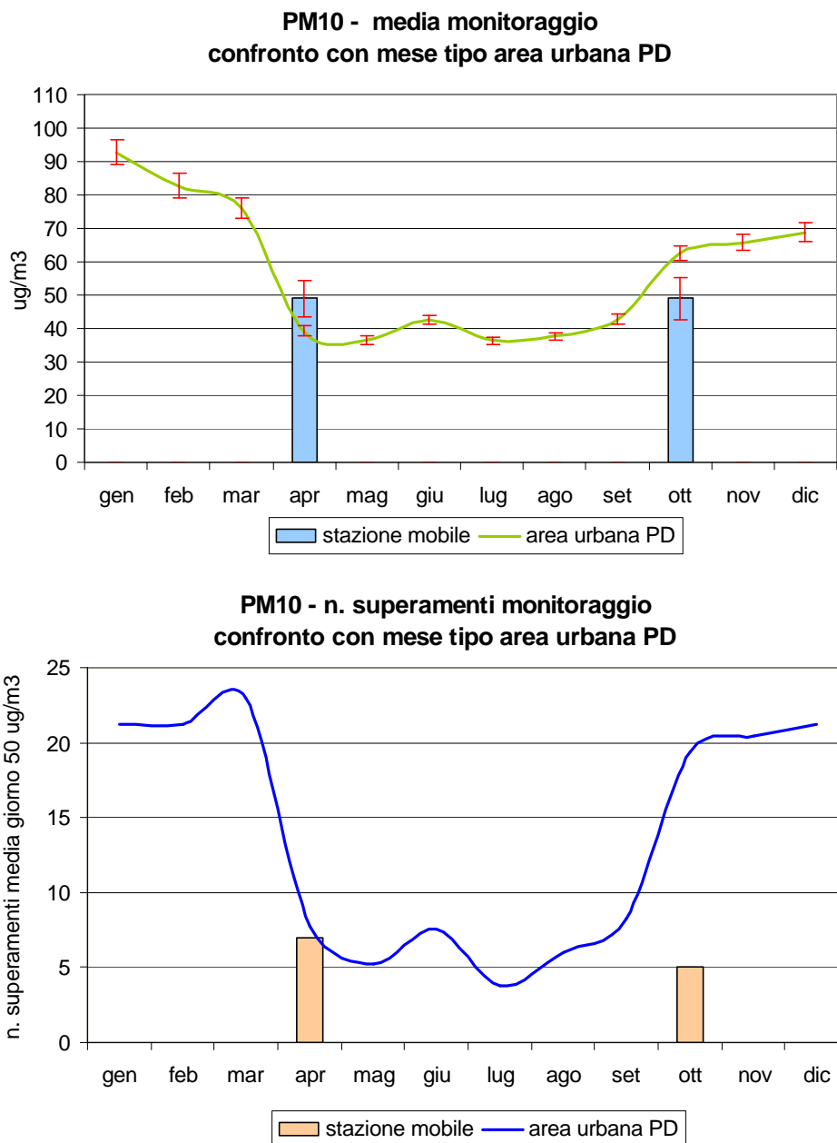
Figura 2.5 Polveri fini ( PM_{10} ): concentrazione media e numero di superamenti rilevati durante il monitoraggio dal 28/09/05 al 20/10/05 e dal 22/03/06 al 06/04/06 in Via Casette nel Comune di Baone; confronto con i periodi corrispondenti presso le stazioni fisse di Arcella e Mandria nel Comune di Padova e con l'andamento caratteristico del 'mese tipo' ricavato dalla serie storica nell'area urbana di Padova; per i valori di concentrazione mensile le barre indicano l'errore standard della media.
