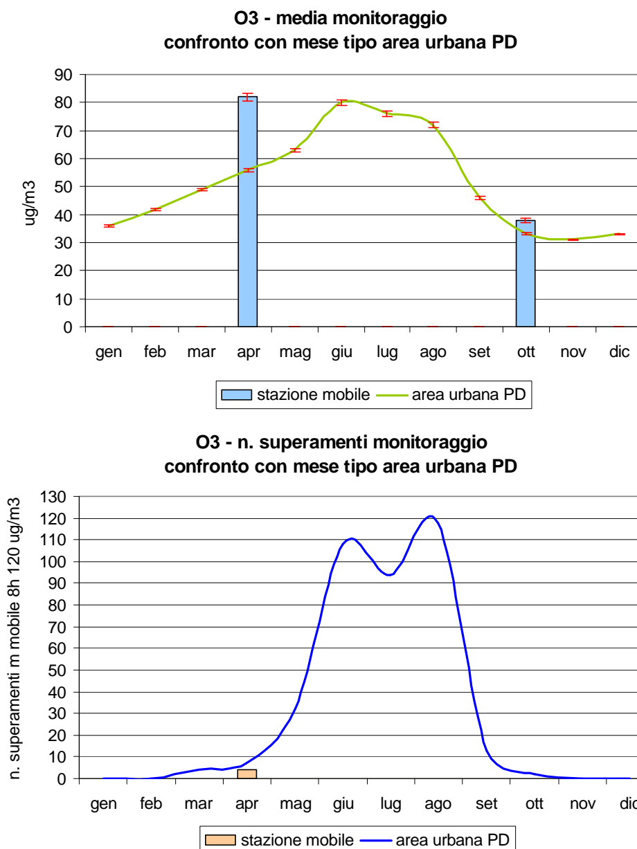
Figura 2.3 Ozono ( O_3 ): concentrazione media e numero di superamenti rilevati durante il monitoraggio dal 28/09/05 al 20/10/05 e dal 22/03/06 al 06/04/06 in Via Casette nel Comune di Baone; confronto con i periodi corrispondenti presso le stazioni fisse di Arcella e Mandria nel Comune di Padova e con l'andamento caratteristico del 'mese tipo' ricavato dalla serie storica nell'area urbana di Padova; per i valori di concentrazione mensile le barre indicano l'errore standard della media.
