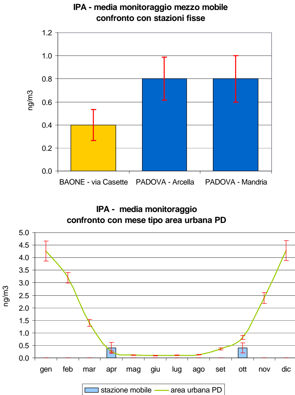
Figura 2.6 Benzo(a)pirene (IPA): concentrazione media rilevata durante il monitoraggio dal 28/09/05 al 20/10/05 e dal 22/03/06 al 06/04/06 in Via Casette nel Comune di Baone; confronto con i periodi corrispondenti presso le stazioni fisse di Arcella e Mandria nel Comune di Padova e con l'andamento caratteristico del 'mese tipo' ricavato dalla serie storica nell'area urbana di Padova; le barre indicano l'errore standard della media.
