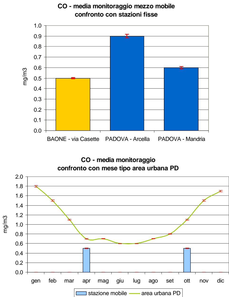
Figura 2.2 Monossido di carbonio (CO): concentrazione media rilevata durante il monitoraggio dal 28/09/05 al 20/10/05 e dal 22/03/06 al 06/04/06 in Via Casette nel Comune di Baone; confronto con i periodi corrispondenti presso le stazioni fisse di Arcella e Mandria nel Comune di Padova e con l'andamento caratteristico del 'mese tipo' ricavato dalla serie storica nell'area urbana di Padova; le barre indicano l'errore standard della media.
