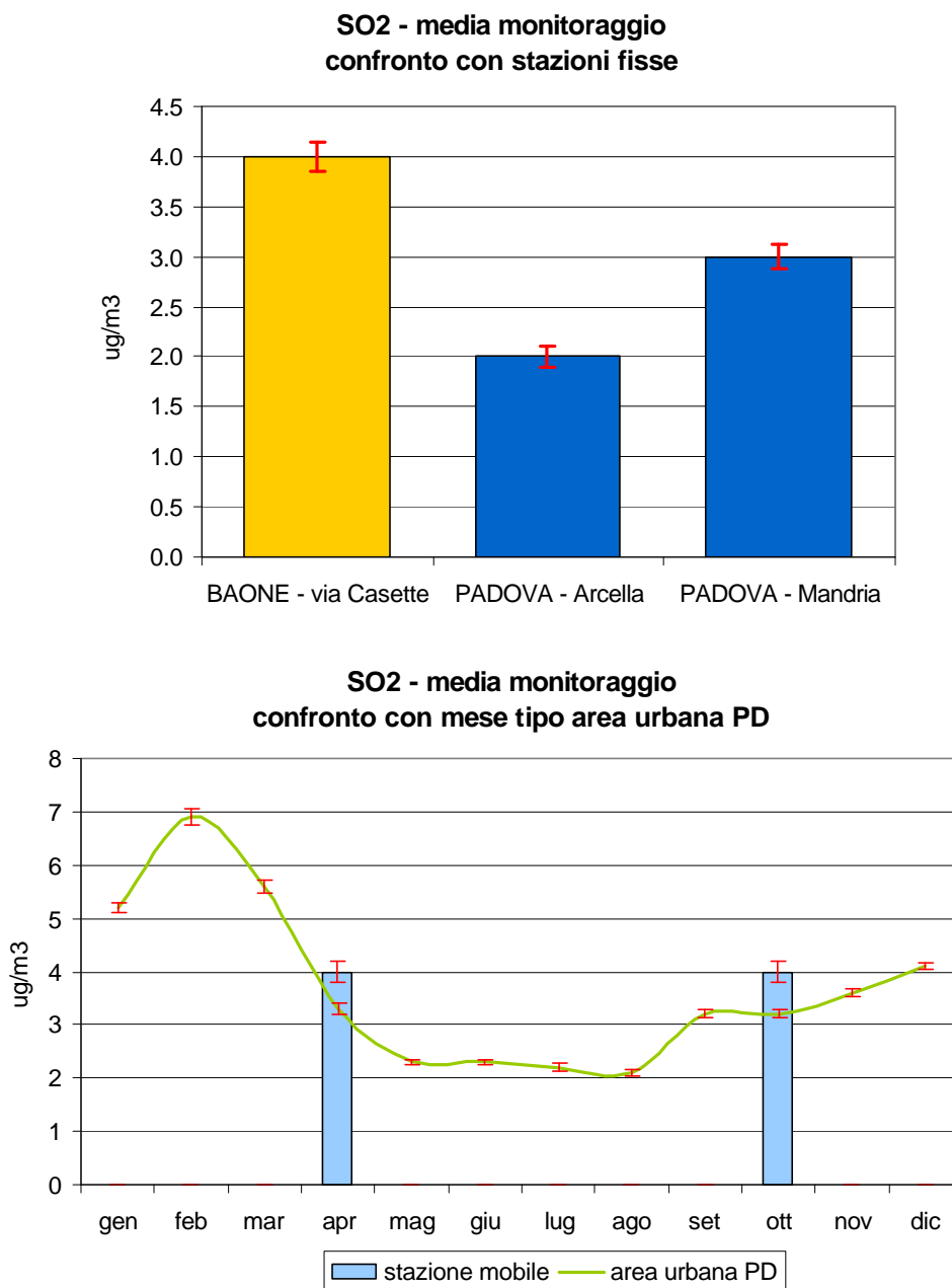
Figura 2.1 Biossido di zolfo (SO 2 ): concentrazione media rilevata durante il monitoraggio dal 28/09/05 al 20/10/05 e dal 22/03/06 al 06/04/06 in Via Casette nel Comune di Baone; confronto con i periodi corrispondenti presso la stazioni fissa di Arcella e di Mandria nel Comune di Padova e con l'andamento caratteristico del 'mese tipo' ricavato dalla serie storica nell'area urbana di Padova; le barre indicano l'errore standard della media.
