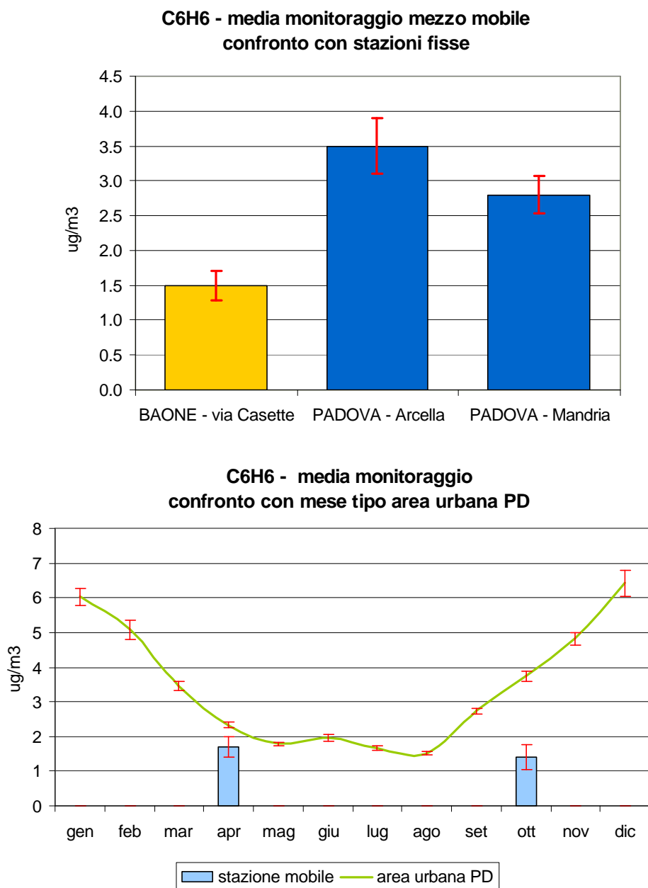
Figura 2.7 Benzene (C 6 H 6 ): concentrazione media rilevata durante il monitoraggio dal 28/09/05 al 20/10/05 e dal 22/03/06 al 06/04/06 in Via Casette nel Comune di Baone; confronto con i periodi corrispondenti presso le stazioni fisse di Arcella e Mandria nel Comune di Padova e con l'andamento caratteristico del 'mese tipo' ricavato dalla serie storica nell'area urbana di Padova; le barre indicano l'errore standard della media.
