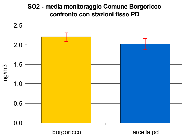
Figura 2.1 Biossido di zolfo (SO 2 ): concentrazione media rilevata durante il monitoraggio dal 12/08/04 al 02/09/04 in Via Desman nel Comune di Borgoricco e confronto con il periodo corrispondente presso la stazione fissa di Mandria nel Comune di Padova; le barre indicano l'errore standard della media.
