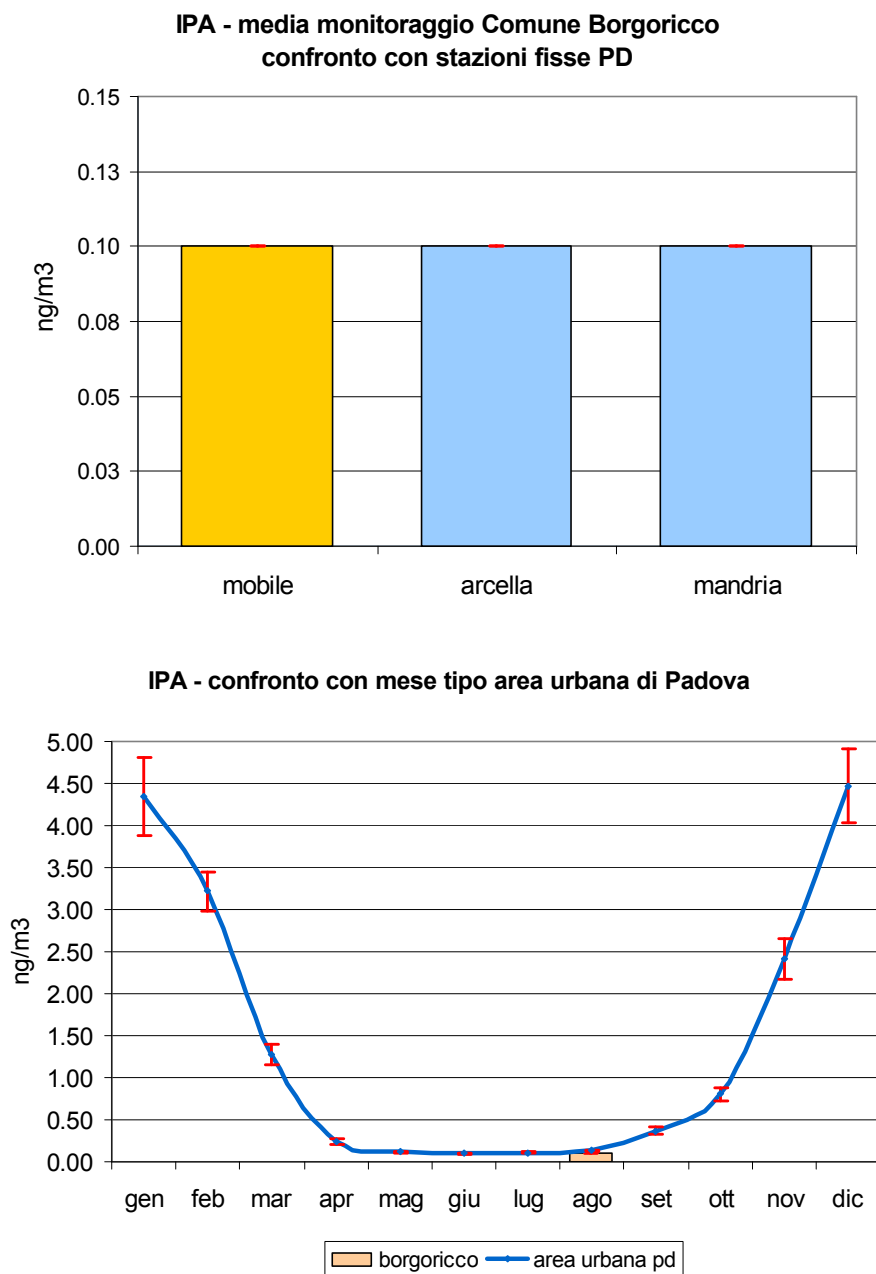
Figura 2.6 Benzo(a)pirene (IPA): concentrazione media rilevata durante il monitoraggio dal 12/08/04 al 02/09/04 in Via Desman nel Comune di Borgoricco e confronto con il periodo corrispondente presso le stazioni fisse di Arcella e Mandria nel Comune di Padova e con l'andamento caratteristico del 'mese tipo' ricavato dalla serie storica; le barre indicano l'errore standard della media.
