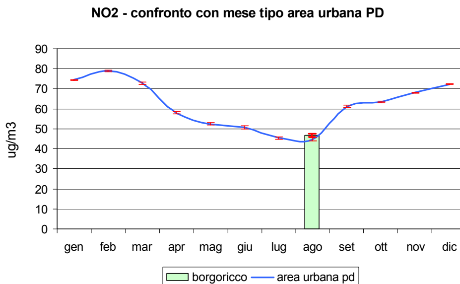
Figura 2.4 Biossido di azoto (NO 2 ): concentrazione media rilevata durante il monitoraggio dal 12/08/04 al 02/09/04 in Via Desman nel Comune di Borgoricco e confronto con il periodo corrispondente presso le stazioni fisse di Arcella e Mandria nel Comune di Padova e con l'andamento caratteristico del 'mese tipo' ricavato dalla serie storica nell'area urbana di Padova; le barre indicano l'errore standard della media.
