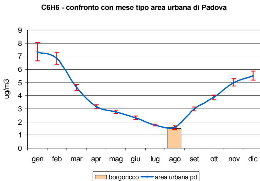
Figura 2.7 Benzene (C 6 H 6 ): concentrazione media rilevata durante il monitoraggio dal 12/08/04 al 02/09/04 in Via Desman nel Comune di Borgoricco e confronto con il periodo corrispondente presso le stazioni fisse di Arcella e Mandria nel Comune di Padova e con l'andamento caratteristico del 'mese tipo' ricavato dalla serie storica; le barre indicano l'errore standard della media.
