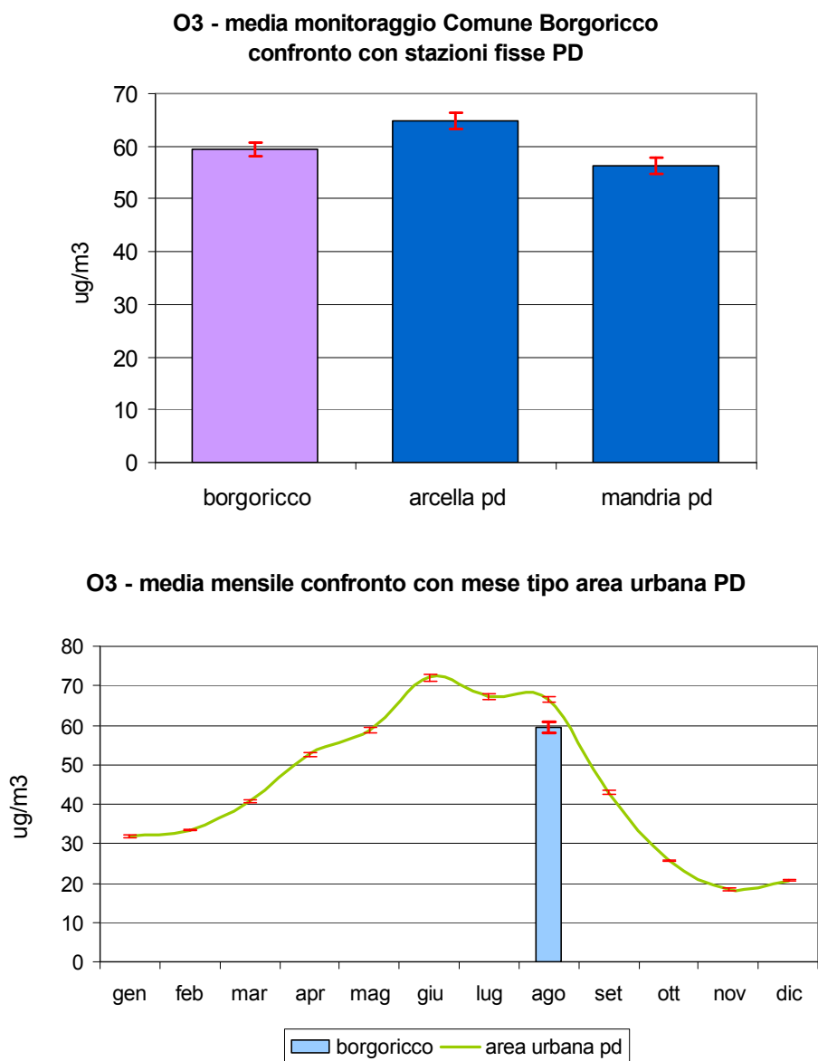
Figura 2.3 Ozono (O 3 ): concentrazione media rilevata durante il monitoraggio dal 12/08/04 al 02/09/04 in Via Desman nel Comune di Borgoricco e confronto con il periodo corrispondente presso le stazioni fisse di Arcella e Mandria nel Comune di Padova e con l'andamento caratteristico del 'mese tipo' ricavato dalla serie storica nell'area urbana di Padova; le barre indicano l'errore standard della media.
