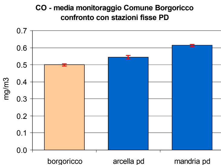
Figura 2.2 Monossido di carbonio (CO): concentrazione media rilevata durante il monitoraggio dal 12/08/04 al 02/09/04 in Via Desman nel Comune di Borgoricco e confronto con il periodo corrispondente presso le stazioni fisse di Arcella e Mandria nel Comune di Padova; le barre indicano l'errore standard della media.
