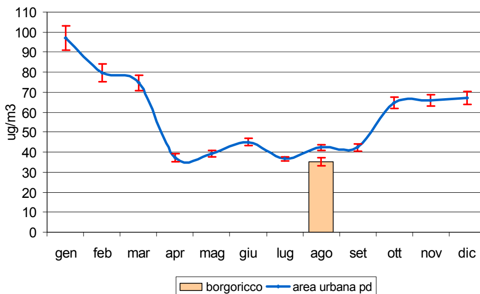
Figura 2.5 Polveri fini ( PM_{10} ): concentrazione media rilevata durante il monitoraggio dal 12/08/04 al 02/09/04 in Via Desman nel Comune di Borgoricco e confronto con il periodo corrispondente presso le stazioni fisse di Arcella e Mandria nel Comune di Padova e con l'andamento caratteristico del 'mese tipo' ricavato dalla serie storica; le barre indicano l'errore standard della media.
