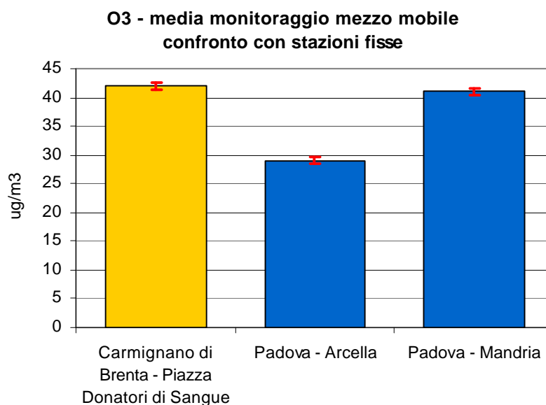
Figura 2.2 Ozono (O 3 ): concentrazione media rilevata durante il monitoraggio in Piazza Donatori di Sangue nel Comune di Carmignano di Brenta, e confronto con i periodi corrispondenti presso le stazioni fisse di Arcella e Mandria; le barre indicano l'errore standard della media.
