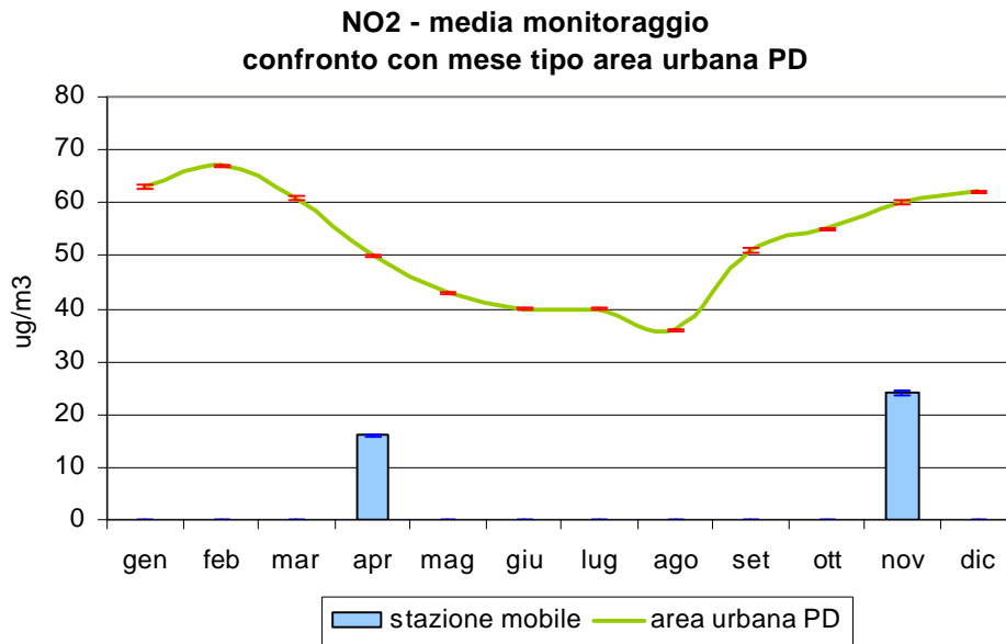
Figura 3.4 Biossido di azoto (NO 2 ): confronto delle concentrazioni medie rilevate durante il monitoraggio in Piazza Donatori di Sangue nel Comune di Carmignano di Brenta, con l'andamento caratteristico del 'mese tipo' ricavato dalla serie storica nell'area urbana di Padova; le barre indicano l'errore standard della media.
