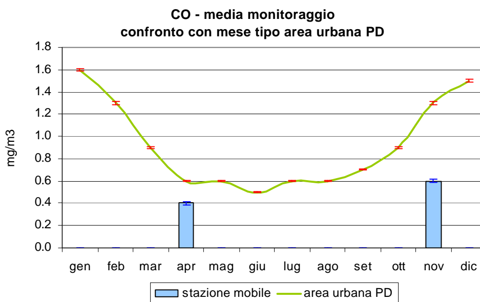
Figura 3.1 Monossido di carbonio (CO): confronto delle concentrazioni medie rilevate durante il monitoraggio in Piazza Donatori di Sangue nel Comune di Carmignano di Brenta, con l'andamento caratteristico del 'mese tipo' ricavato dalla serie storica nell'area urbana di Padova; le barre indicano l'errore standard della media.
