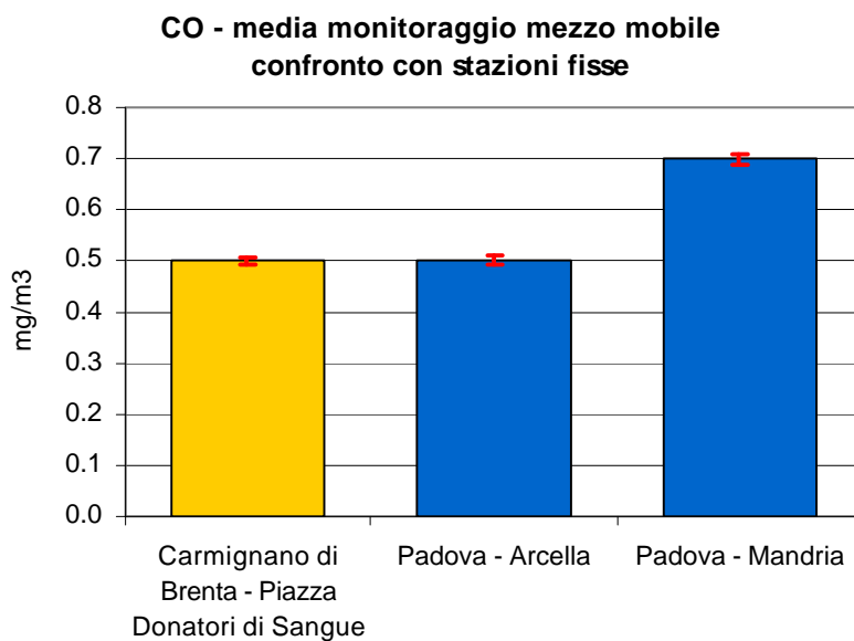
Figura 2.1 Monossido di carbonio (CO): concentrazione media rilevata durante il monitoraggio in Piazza Donatori di Sangue nel Comune di Carmignano di Brenta, e confronto con i periodi corrispondenti presso le stazioni fisse di Arcella e Mandria nel Comune di Padova; le barre indicano l'errore standard della media.
