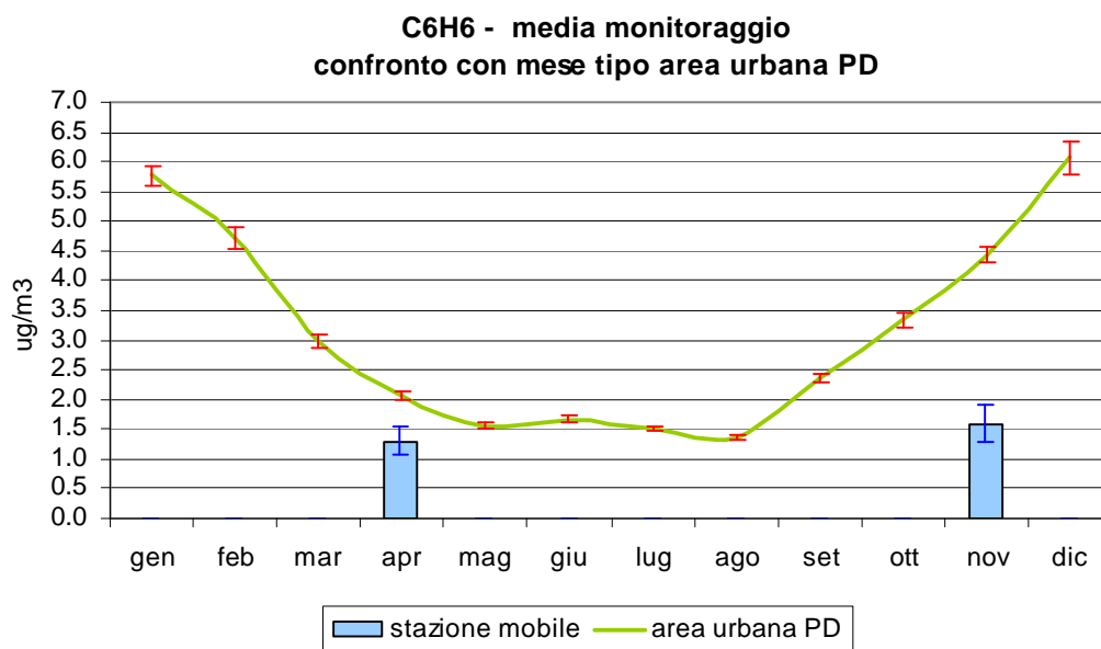
Figura 3.6 Benzene (C 6 H 6 ): confronto delle concentrazioni medie rilevate durante il monitoraggio in Piazza Donatori di Sangue nel Comune di Carmignano di Brenta, con l'andamento caratteristico del 'mese tipo' ricavato dalla serie storica nell'area urbana di Padova; le barre indicano l'errore standard della media.
