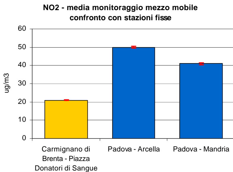
Figura 2.3 Biossido di azoto (NO 2 ): concentrazione media rilevata durante il monitoraggio in Piazza Donatori di Sangue nel Comune di Carmignano di Brenta, e confronto con i periodi corrispondenti presso le stazioni fisse di Arcella e Mandria; le barre indicano l'errore standard della media.
