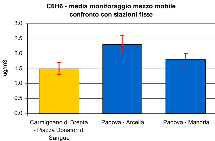
Figura 2.6 Benzene (C 6 H 6 ): concentrazione media rilevata durante il monitoraggio in Piazza Donatori di Sangue nel Comune di Carmignano di Brenta, e confronto con i periodi corrispondenti presso le stazioni fisse nel Comune di Padova; le barre indicano l'errore standard della media.
