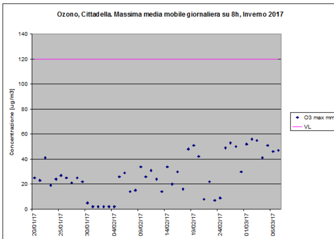
Figura 10.1: Concentrazione Massima Giornaliera della Media Mobile di 8h di Ozono - semestre invernale
