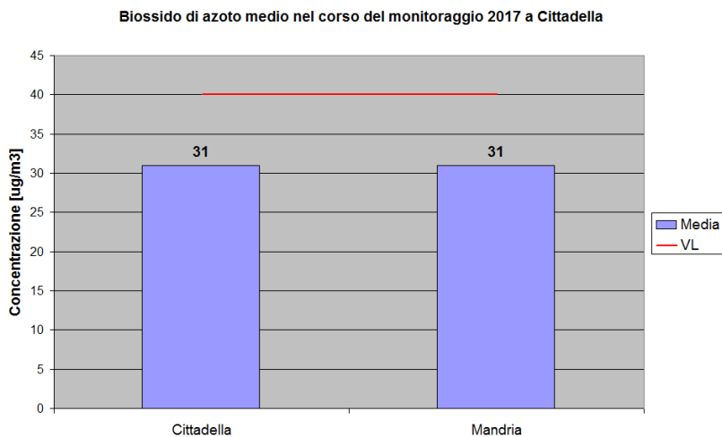
Figura 6.2: Monitoraggio del Biossido di Azoto a Cittadella
