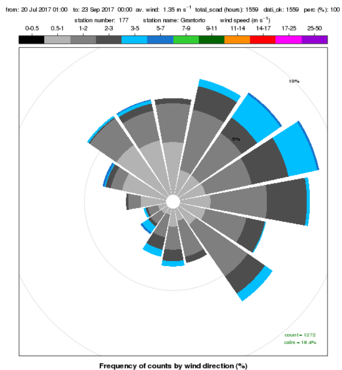
Figura 2.4: Rosa dei venti registrati presso la stazione di Grantorto nel corso della CAMPAGNA ESTIVA
