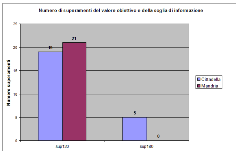
Figura 6.1: Monitoraggio dell'Ozono a Cittadella
