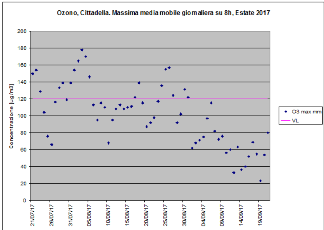
Figura 10.2: Concentrazione Massima Giornaliera della Media Mobile di 8h di Ozono - semestre estivo
