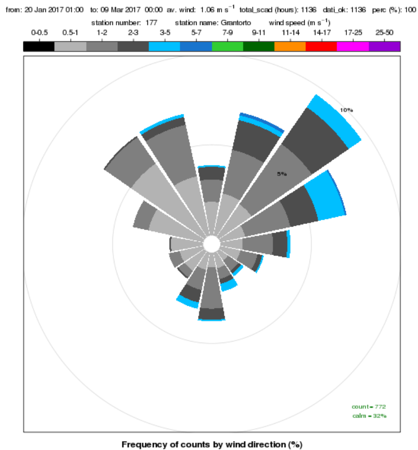
Figura 2.2: Rosa dei venti registrati presso la stazione meteo nel corso della CAMPAGNA INVERNALE
