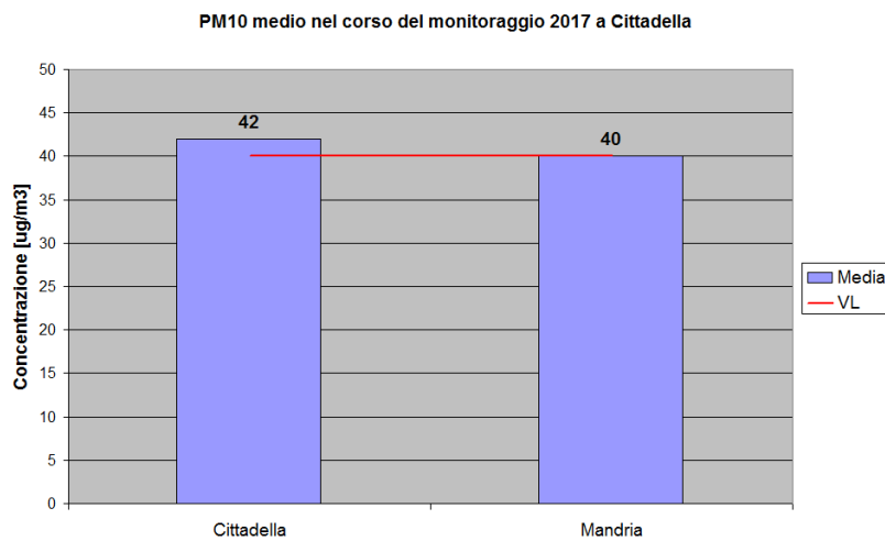
Figura 6.3: Monitoraggio del particolato sottile a Cittadella
