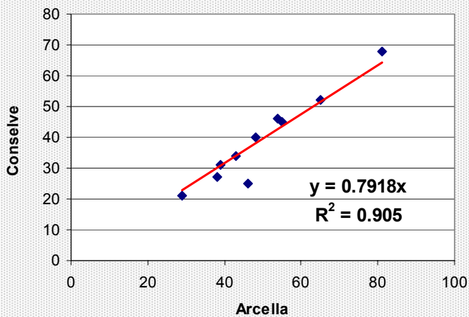
Correlazione Arcella - Conselve
