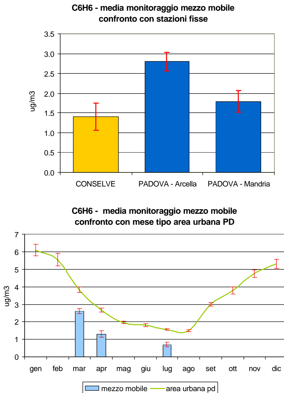
Figura 2.7 Benzene ( C_6H_6 ): concentrazione media rilevata durante il monitoraggio nel Comune di Conselve; confronto con i periodi corrispondenti presso le stazioni fisse di Arcella e Mandria nel Comune di Padova e con l'andamento caratteristico del 'mese tipo' ricavato dalla serie storica nell'area urbana di Padova; le barre indicano l'errore standard della media.
