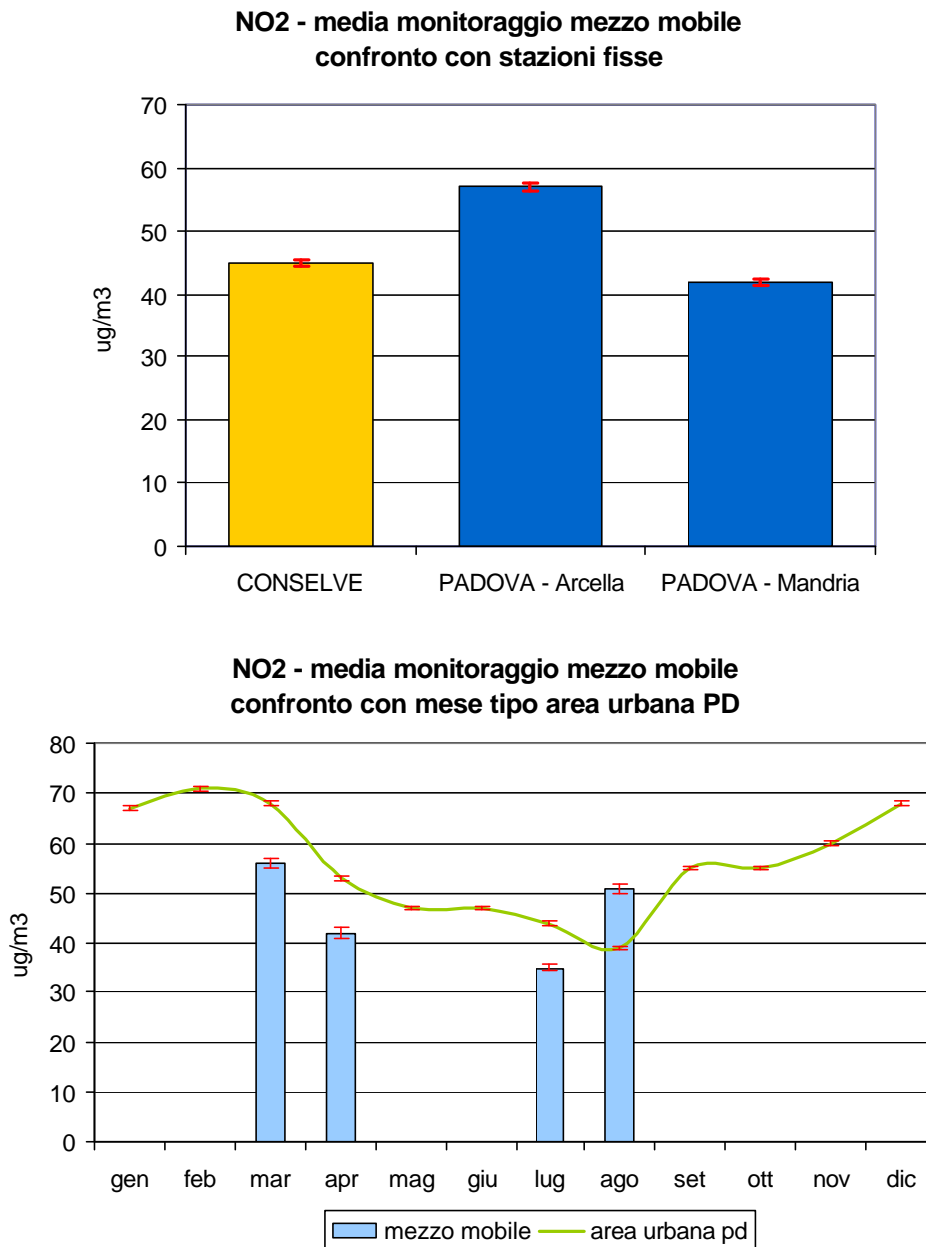
Figura 2.4 Biossido di azoto (NO 2 ): concentrazione media rilevata durante il monitoraggio nel Comune di Conselve; confronto con i periodi corrispondenti presso le stazioni fisse di Arcella e Mandria nel Comune di Padova e con l'andamento caratteristico del 'mese tipo' ricavato dalla serie storica nell'area urbana di Padova; le barre indicano l'errore standard della media.
