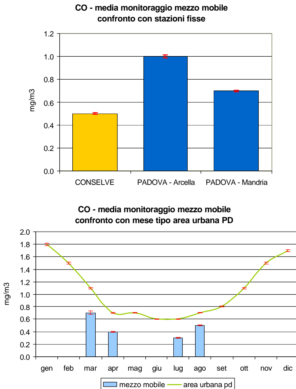
Figura 2.2 Monossido di carbonio (CO): concentrazione media rilevata durante il monitoraggio nel Comune di Conselve; confronto con i periodi corrispondenti presso le stazioni fisse di Arcella e di Mandria nel Comune di Padova e con l'andamento caratteristico del 'mese tipo' ricavato dalla serie storica nell'area urbana di Padova; le barre indicano l'errore standard della media.
