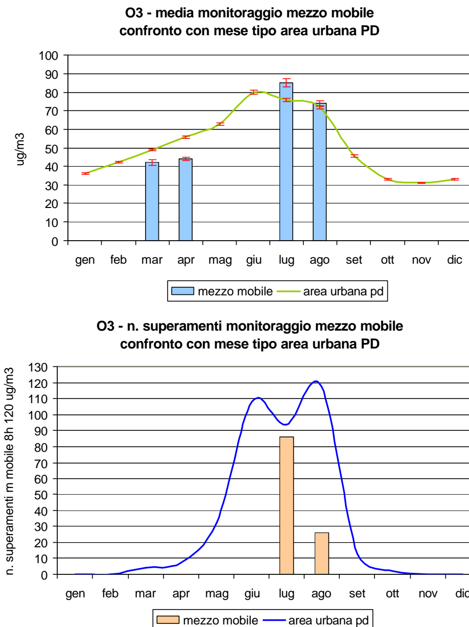
Figura 2.3 Ozono ( O_3 ): concentrazione media e numero di superamenti rilevati durante il monitoraggio nel Comune di Conselve; confronto con i periodi corrispondenti presso le stazioni fisse di Arcella e di Mandria nel Comune di Padova e con l'andamento caratteristico del 'mese tipo' ricavato dalla serie storica nell'area urbana di Padova; per i valori di concentrazione mensile le barre indicano l'errore standard della media.
