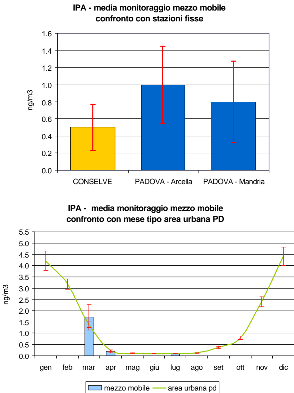
Figura 2.6 Benzo(a)pirene (IPA): concentrazione media rilevata durante il monitoraggio nel Comune di Conselve; confronto con i periodi corrispondenti presso le stazioni fisse di Arcella e Mandria nel Comune di Padova e con l'andamento caratteristico del 'mese tipo' ricavato dalla serie storica nell'area urbana di Padova; le barre indicano l'errore standard della media.
