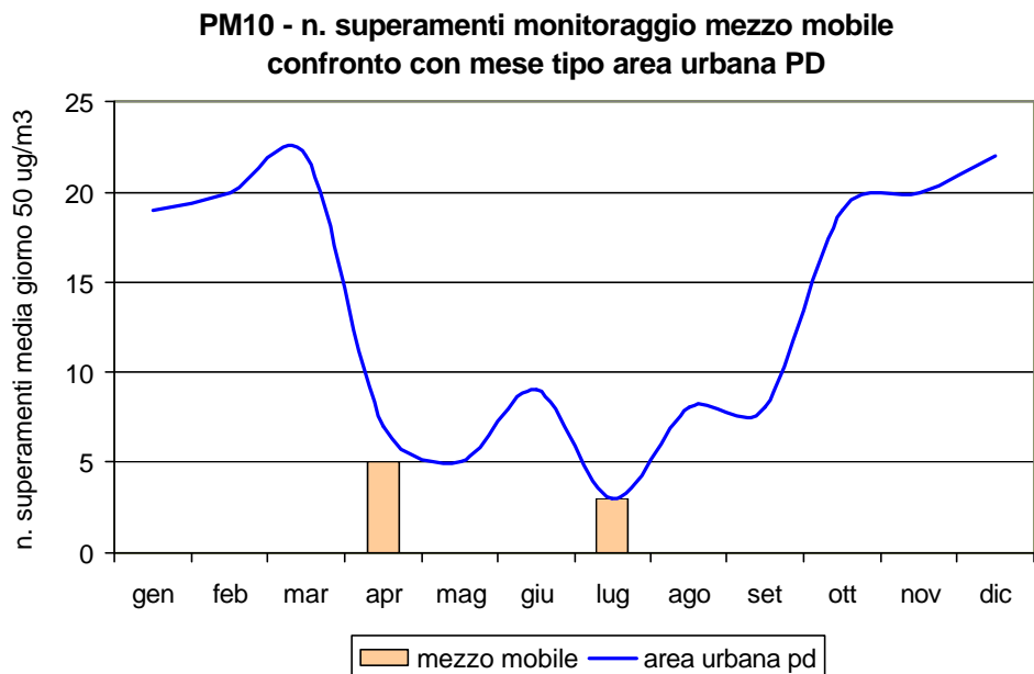
Figura 2.5 Polveri fini (PM 10 ): concentrazione media e numero di superamenti rilevati durante il monitoraggio nel Comune di Conselve; confronto con i periodi corrispondenti presso le stazioni fisse di Arcella e Mandria nel Comune di Padova e con l'andamento caratteristico del 'mese tipo' ricavato dalla serie storica nell'area urbana di Padova; per i valori di concentrazione mensile le barre indicano l'errore standard della media.
