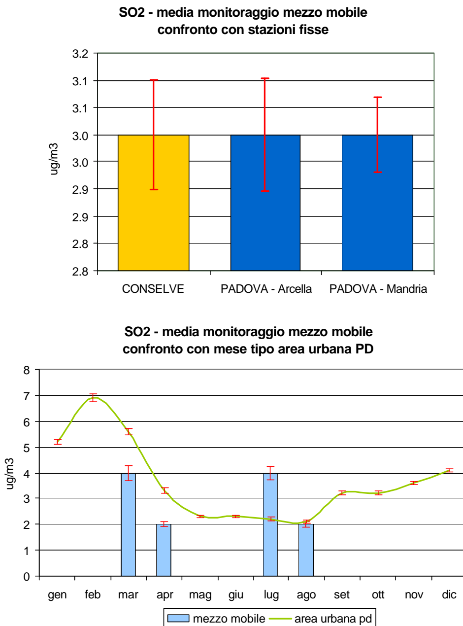
Figura 2.1 Biossido di zolfo (SO 2 ): concentrazione media rilevata durante il monitoraggio nel Comune di Conselve; confronto con i periodi corrispondenti presso la stazioni fisse di Arcella e Mandria nel Comune di Padova e con l'andamento caratteristico del 'mese tipo' ricavato dalla serie storica nell'area urbana di Padova; le barre indicano l'errore standard della media.
