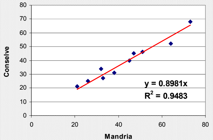
Correlazione Mandria - Conselve
