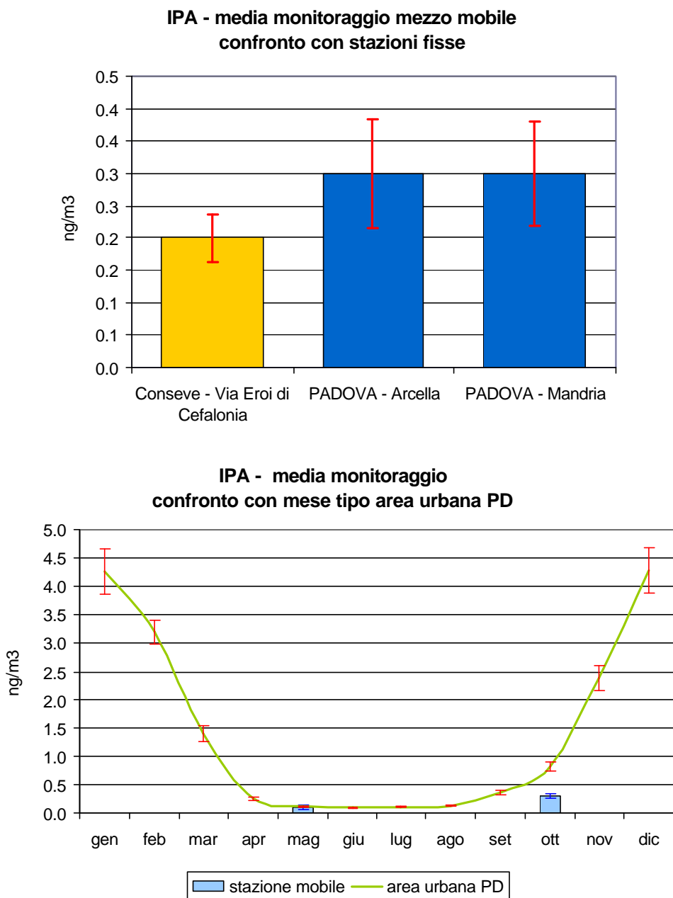
Figura 2.6 Benzo(a)pirene (IPA): concentrazione media rilevata durante il monitoraggio dal 20/04/07 al 16/05/07 e dal 27/09/07 al 23/10/07 in Via Eroi di Cefalonia nel Comune di Conserve; confronto con i periodi corrispondenti presso le stazioni fisse di Arcella e Mandria nel Comune di Padova e con l'andamento caratteristico del 'mese tipo' ricavato dalla serie storica nell'area urbana di Padova; le barre indicano l'errore standard della media.
