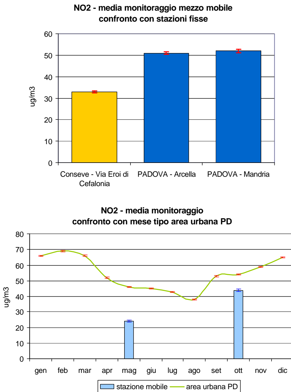
Figura 2.4 Biossido di azoto (NO 2 ): concentrazione media rilevata durante il monitoraggio dal 20/04/07 al 16/05/07 e dal 27/09/07 al 23/10/07 in Via Eroi di Cefalonia nel Comune di Conselve; confronto con i periodi corrispondenti presso le stazioni fisse di Arcella e Mandria nel Comune di Padova e con l'andamento caratteristico del 'mese tipo' ricavato dalla serie storica nell'area urbana di Padova; le barre indicano l'errore standard della media.
