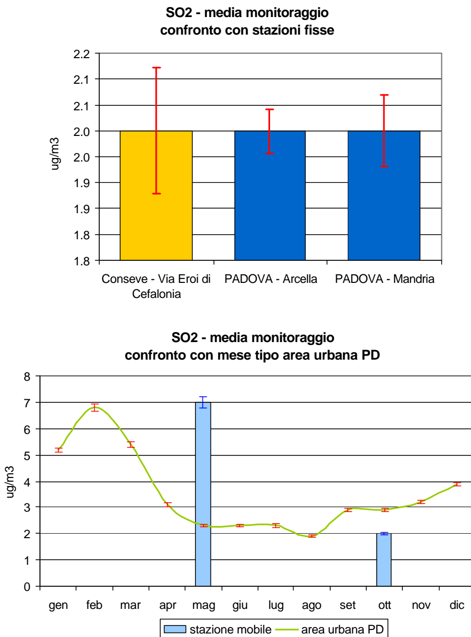
Figura 2.1 Biossido di zolfo (SO 2 ): concentrazione media rilevata durante il monitoraggio dal 20/04/07 al 16/05/07 e dal 27/09/07 al 23/10/07 in Via Eroi di Cefalonia nel Comune di Conserve; confronto con i periodi corrispondenti presso la stazioni fissa di Arcella e di Mandria nel Comune di Padova e con l'andamento caratteristico del 'mese tipo' ricavato dalla serie storica nell'area urbana di Padova; le barre indicano l'errore standard della media.
