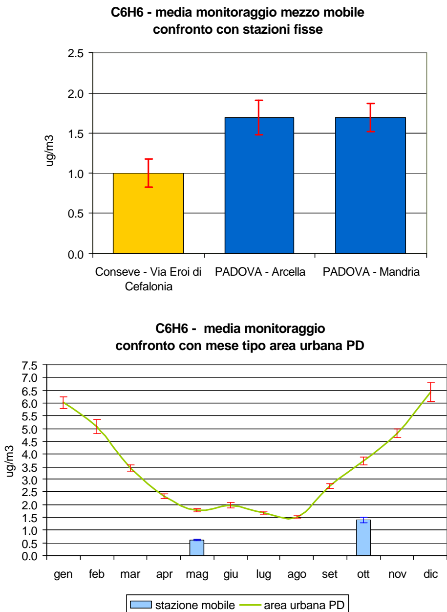
Figura 2.7 Benzene ( C_6H_6 ): concentrazione media rilevata durante il monitoraggio dal 20/04/07 al 16/05/07 e dal 27/09/07 al 23/10/07 in Via Eroi di Cefalonia nel Comune di Consegue; confronto con i periodi corrispondenti presso le stazioni fisse di Arcella e Mandria nel Comune di Padova e con l'andamento caratteristico del 'mese tipo' ricavato dalla serie storica nell'area urbana di Padova; le barre indicano l'errore standard della media.
