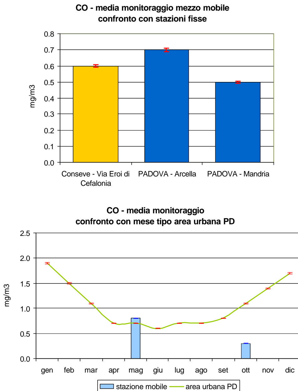
Figura 2.2 Monossido di carbonio (CO): concentrazione media rilevata durante il monitoraggio dal 20/04/07 al 16/05/07 e dal 27/09/07 al 23/10/07 in Via Eroi di Cefalonia nel Comune di Conserve; confronto con i periodi corrispondenti presso le stazioni fisse di Arcella e Mandria nel Comune di Padova e con l'andamento caratteristico del 'mese tipo' ricavato dalla serie storica nell'area urbana di Padova; le barre indicano l'errore standard della media.
