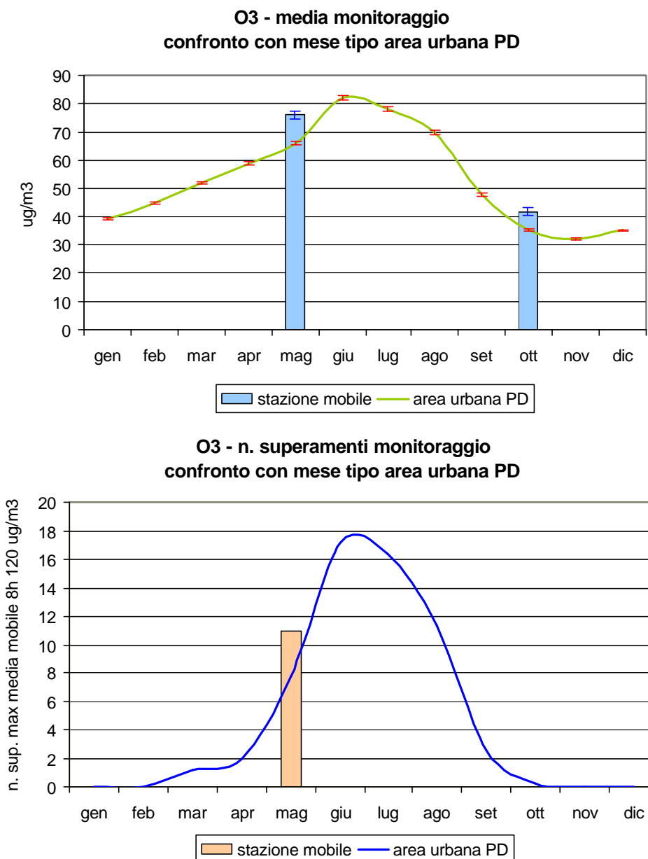
Figura 2.3 Ozono (O 3 ): concentrazione media e numero di superamenti rilevati durante il monitoraggio dal 20/04/07 al 16/05/07 e dal 27/09/07 al 23/10/07 in Via Eroi di Cefalonia nel Comune di Conselve; confronto con i periodi corrispondenti presso le stazioni fisse di Arcella e Mandria nel Comune di Padova e con l'andamento caratteristico del 'mese tipo' ricavato dalla serie storica nell'area urbana di Padova; per i valori di concentrazione mensile le barre indicano l'errore standard della media.
