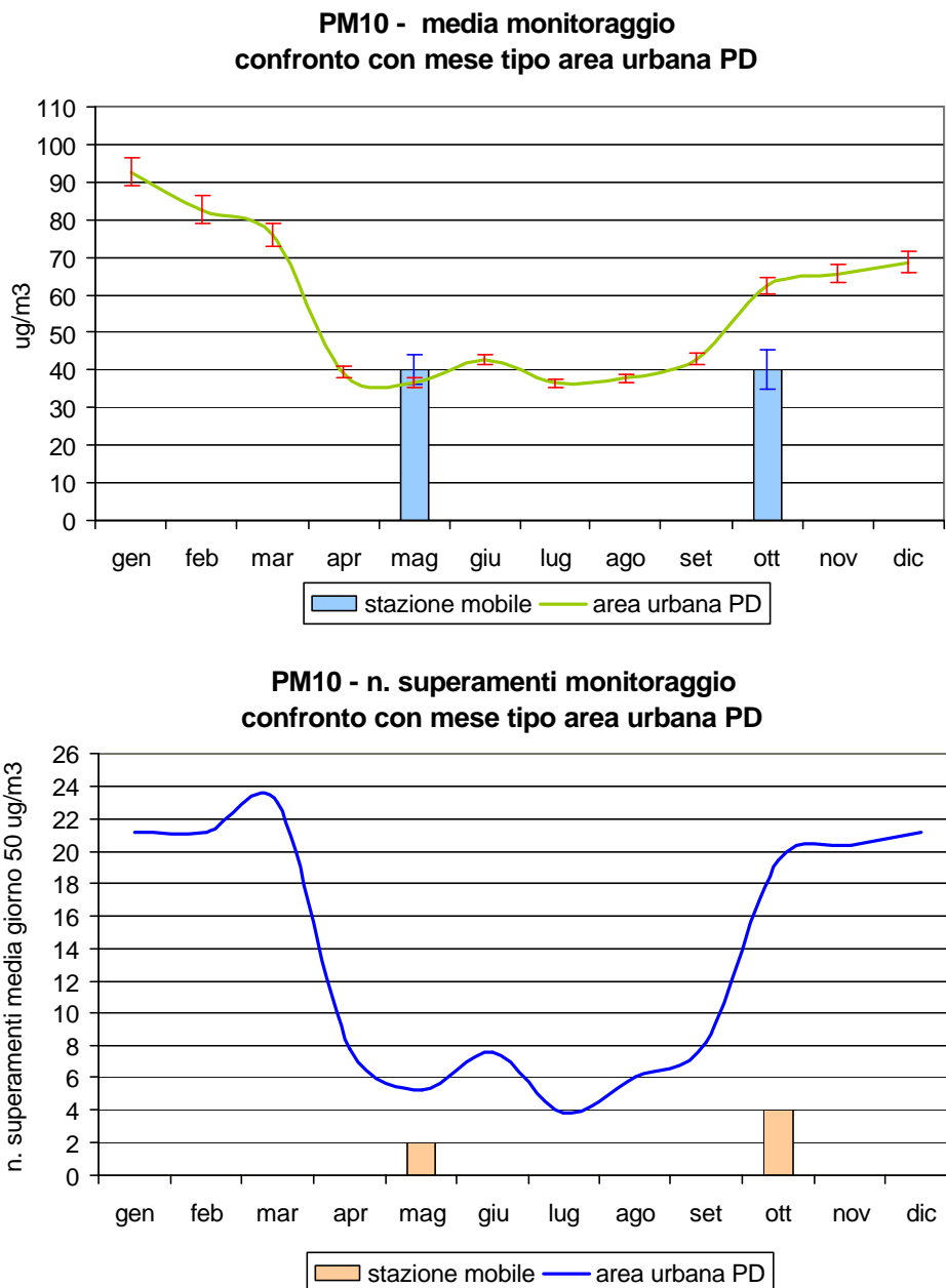
Figura 2.5 Polveri fini ( PM_{10} ): concentrazione media e numero di superamenti rilevati durante il monitoraggio dal 20/04/07 al 16/05/07 e dal 27/09/07 al 23/10/07 in Via Eroi di Cefalonia nel Comune di Conselve; confronto con i periodi corrispondenti presso le stazioni fisse di Arcella e Mandria nel Comune di Padova e con l'andamento caratteristico del 'mese tipo' ricavato dalla serie storica nell'area urbana di Padova; per i valori di concentrazione mensile le barre indicano l'errore standard della media.
