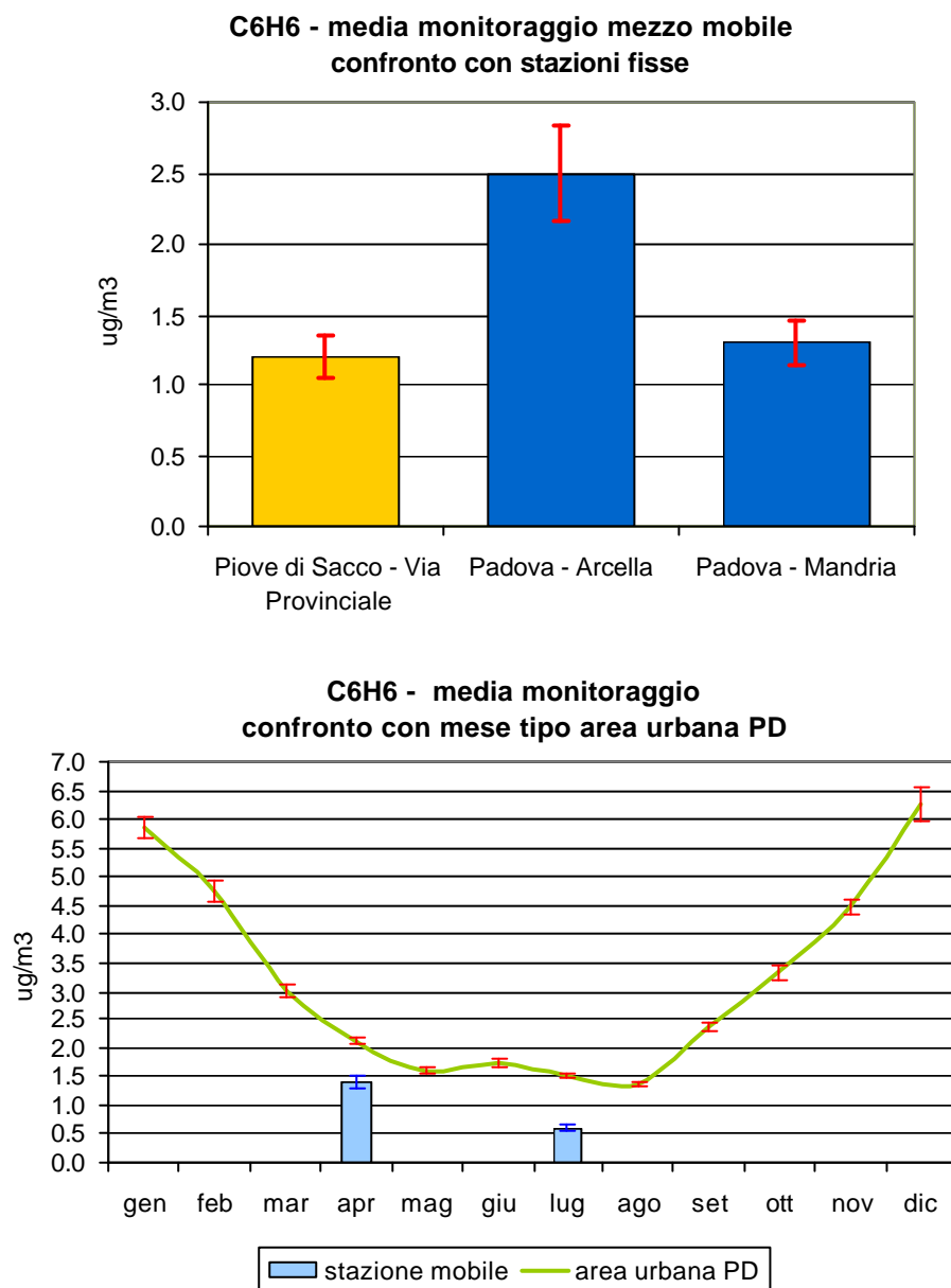
Figura 2.7 Benzene (C 6 H 6 ): concentrazione media rilevata durante il monitoraggio dal 29/02/08 al 27/04/08 e dal 17/06/08 al 08/07/08 in Via Provinciale nel Comune di Piove di Sacco; confronto con i periodi corrispondenti presso le stazioni fisse di Arcella e Mandria nel Comune di Padova e con l'andamento caratteristico del 'mese tipo' ricavato dalla serie storica nell'area urbana di Padova; le barre indicano l'errore standard della media.
