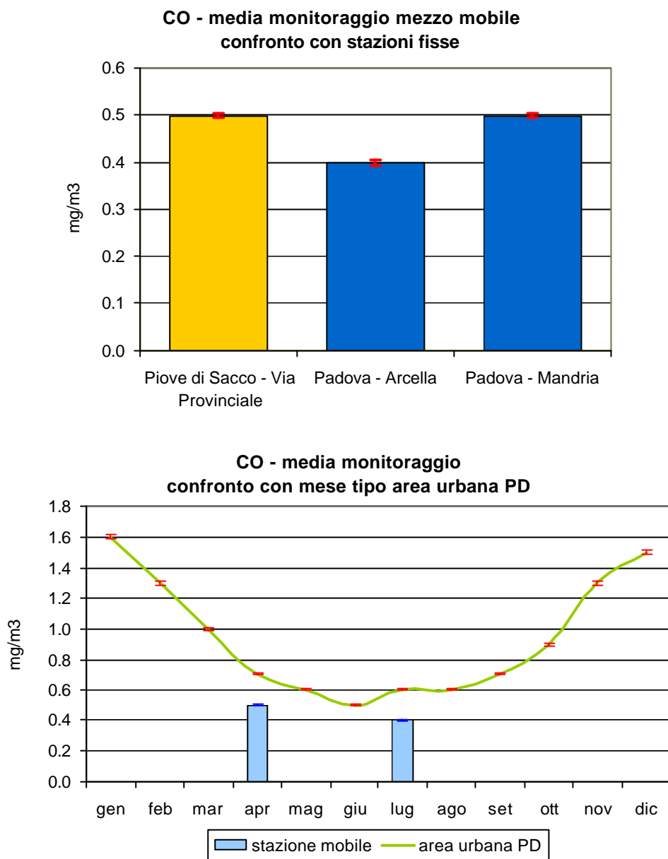
Figura 2.2 Monossido di carbonio (CO): concentrazione media rilevata durante il monitoraggio dal 29/02/08 al 27/04/08 e dal 17/06/08 al 08/07/08 in Via Provinciale nel Comune di Piove di Sacco; confronto con i periodi corrispondenti presso le stazioni fisse di Arcella e Mandria nel Comune di Padova e con l'andamento caratteristico del 'mese tipo' ricavato dalla serie storica nell'area urbana di Padova; le barre indicano l'errore standard della media.
