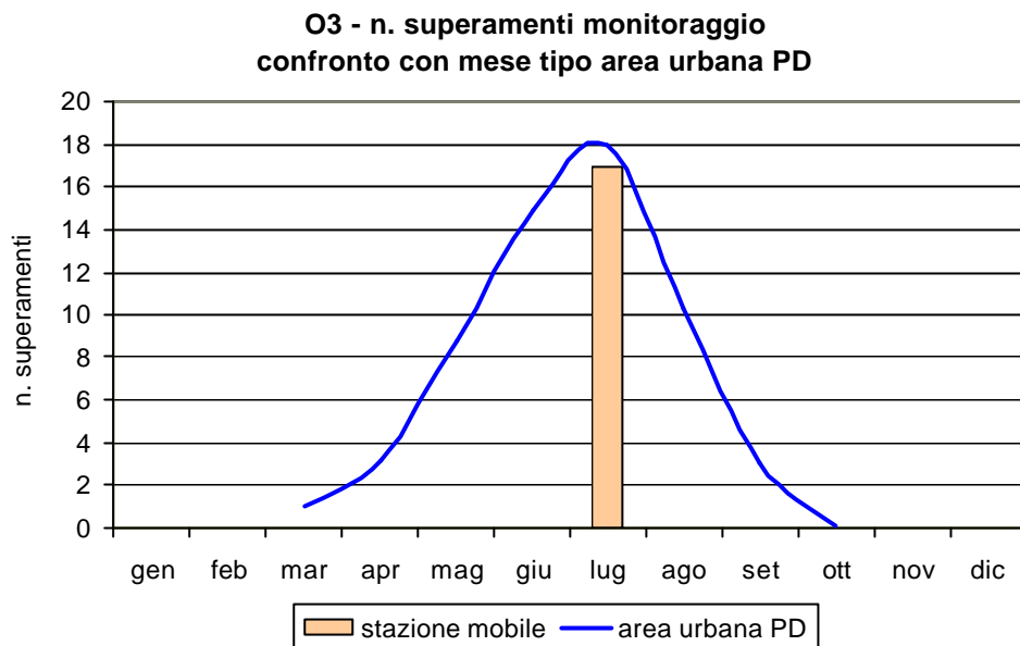
Figura 2.3 Ozono (O 3 ): concentrazione media e numero di superamenti del valore del limite di protezione della salute (120 \mu\text{g}/\text{m}^3 ) rilevati durante il monitoraggio 29/02/08 al 27/04/08 e dal 17/06/08 al 08/07/08 in Via Provinciale nel Comune di Piove di Sacco; confronto con i periodi corrispondenti presso le stazioni fisse di Arcella e Mandria nel Comune di Padova e con l'andamento caratteristico del 'mese tipo' ricavato dalla serie storica nell'area urbana di Padova; per i valori di concentrazione mensile le barre indicano l'errore standard della media.
