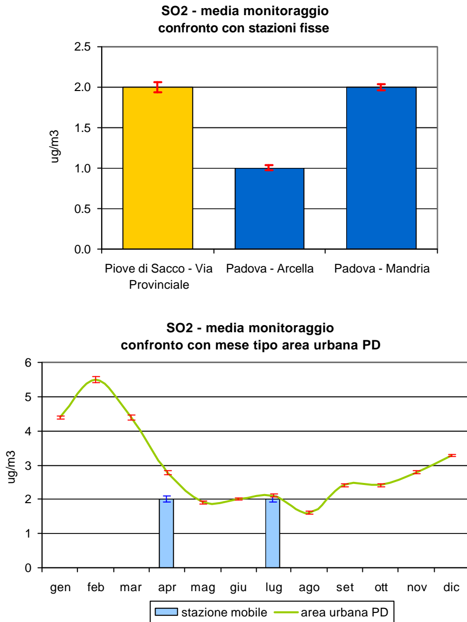
Figura 2.1 Biossido di zolfo (SO 2 ): concentrazione media rilevata durante il monitoraggio dal 29/02/08 al 27/04/08 e dal 17/06/08 al 08/07/08 in Via Provinciale nel Comune di Piove di Sacco; confronto con i periodi corrispondenti presso le stazioni fisse di Arcella e di Mandria nel Comune di Padova e con l'andamento caratteristico del 'mese tipo' ricavato dalla serie storica nell'area urbana di Padova; le barre indicano l'errore standard della media.
