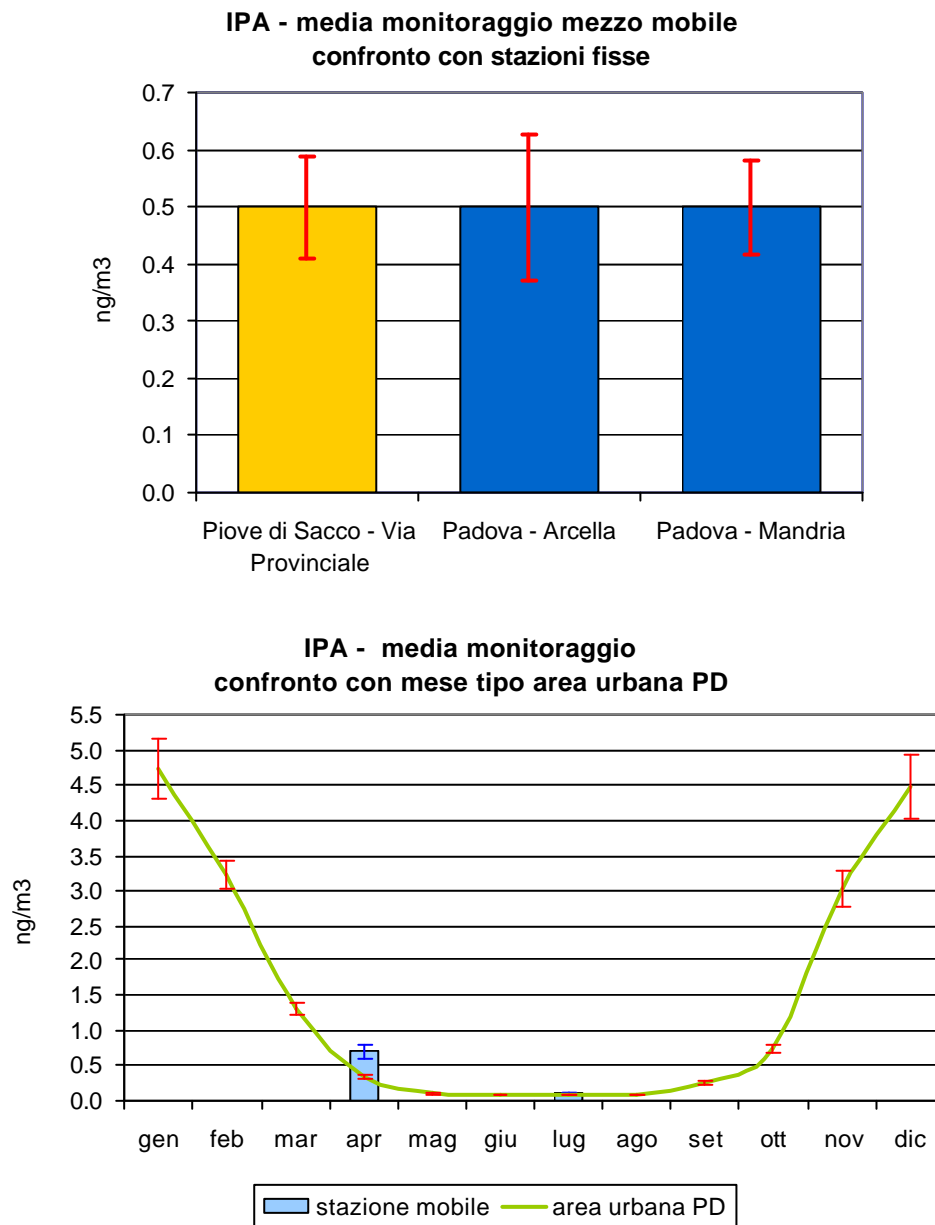
Figura 2.6 Benzo(a)pirene (IPA): concentrazione media rilevata durante il monitoraggio dal 29/02/08 al 27/04/08 e dal 17/06/08 al 08/07/08 in Via Provinciale nel Comune di Piove di Sacco; confronto con i periodi corrispondenti presso le stazioni fisse di Arcella e Mandria nel Comune di Padova e con l'andamento caratteristico del 'mese tipo' ricavato dalla serie storica nell'area urbana di Padova; le barre indicano l'errore standard della media.
