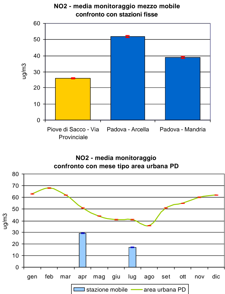
Figura 2.4 Biossido di azoto (NO 2 ): concentrazione media rilevata durante il monitoraggio dal 29/02/08 al 27/04/08 e dal 17/06/08 al 08/07/08 in Via Provinciale nel Comune di Piove di Sacco; confronto con i periodi corrispondenti presso le stazioni fisse di Arcella e Mandria nel Comune di Padova e con l'andamento caratteristico del 'mese tipo' ricavato dalla serie storica nell'area urbana di Padova; le barre indicano l'errore standard della media.
