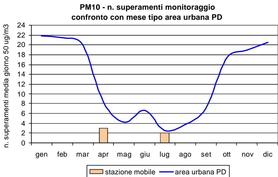
Figura 2.5 Polveri fini (PM 10 ): concentrazione media e numero di superamenti rilevati durante il monitoraggio dal 29/02/08 al 27/04/08 e dal 17/06/08 al 08/07/08 in Via Provinciale nel Comune di Piove di Sacco; confronto con i periodi corrispondenti presso le stazioni fisse di Arcella e Mandria nel Comune di Padova e con l'andamento caratteristico del 'mese tipo' ricavato dalla serie storica nell'area urbana di Padova; per i valori di concentrazione mensile le barre indicano l'errore standard della media.
