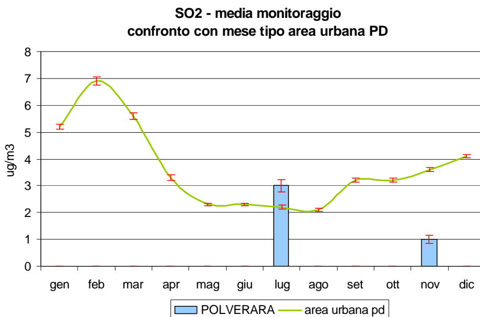
Figura 2.1 Biossido di zolfo (SO 2 ): concentrazione media rilevata durante il monitoraggio dal 16/06/05 al 06/07/05 e dal 26/10/05 al 10/11/05 nel Comune di Polverara; confronto con i periodi corrispondenti presso la stazioni fissa di Arcella e di Mandria nel Comune di Padova e con l'andamento caratteristico del 'mese tipo' ricavato dalla serie storica nell'area urbana di Padova; le barre indicano l'errore standard della media.
