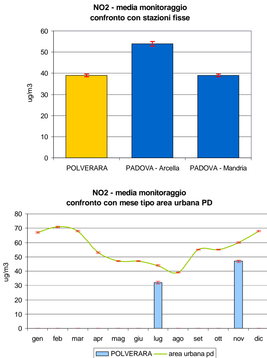
Figura 2.4 Biossido di azoto ( \text{NO}_2 ): concentrazione media rilevata durante il monitoraggio dal 16/06/05 al 06/07/05 e dal 26/10/05 al 10/11/05 nel Comune di Polverara; confronto con i periodi corrispondenti presso le stazioni fisse di Arcella e Mandria nel Comune di Padova e con l'andamento caratteristico del 'mese tipo' ricavato dalla serie storica nell'area urbana di Padova; le barre indicano l'errore standard della media.
