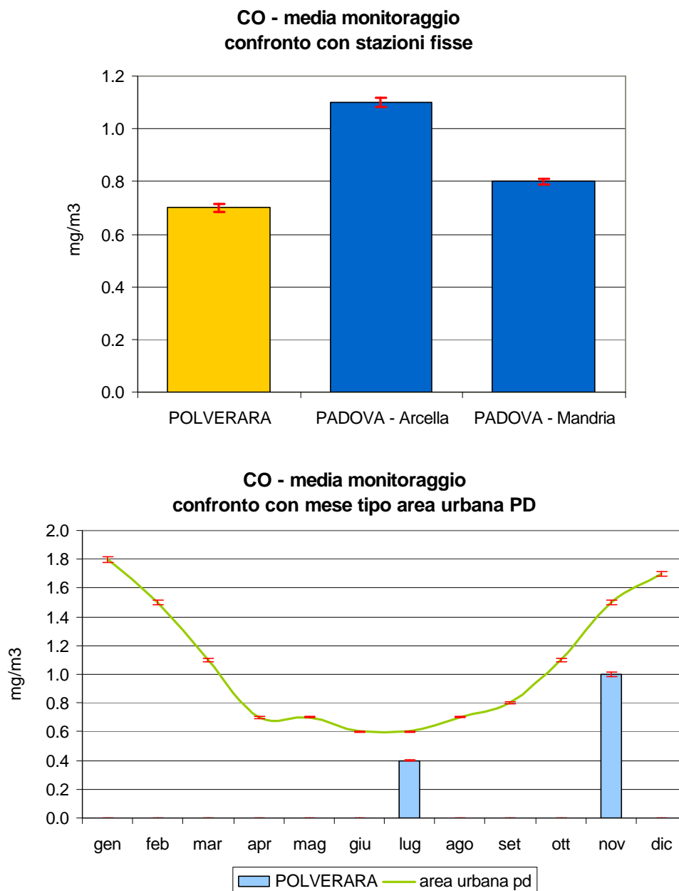
Figura 2.2 Monossido di carbonio (CO): concentrazione media rilevata durante il monitoraggio dal 16/06/05 al 06/07/05 e dal 26/10/05 al 10/11/05 nel Comune di Polverara; confronto con i periodi corrispondenti presso le stazioni fisse di Arcella e Mandria nel Comune di Padova e con l'andamento caratteristico del 'mese tipo' ricavato dalla serie storica nell'area urbana di Padova; le barre indicano l'errore standard della media.
