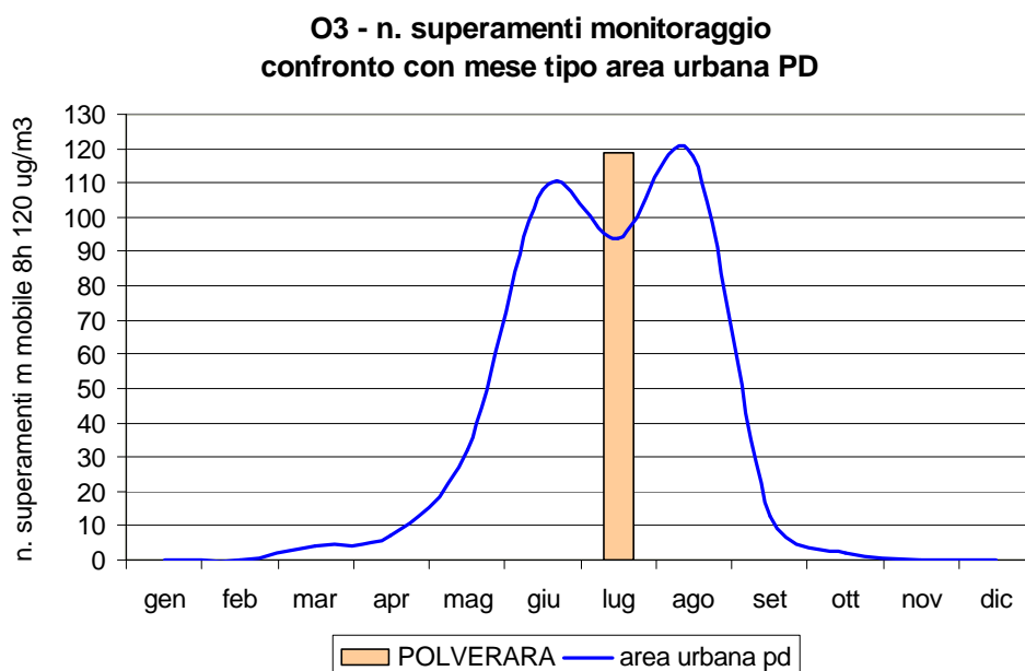
Figura 2.3 Ozono ( O_3 ): concentrazione media e numero di superamenti rilevati durante il monitoraggio dal 16/06/05 al 06/07/05 e dal 26/10/05 al 10/11/05 nel Comune di Polverara; confronto con i periodi corrispondenti presso le stazioni fisse di Arcella e Mandria nel Comune di Padova e con l'andamento caratteristico del 'mese tipo' ricavato dalla serie storica nell'area urbana di Padova; per i valori di concentrazione mensile le barre indicano l'errore standard della media.
