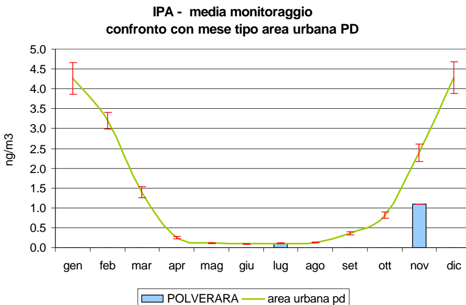
Figura 2.6 Benzo(a)pirene (IPA): concentrazione media rilevata durante il monitoraggio dal 16/06/05 al 06/07/05 e dal 26/10/05 al 10/11/05 nel Comune di Polverara; confronto con i periodi corrispondenti presso le stazioni fisse di Arcella e Mandria nel Comune di Padova e con l'andamento caratteristico del 'mese tipo' ricavato dalla serie storica nell'area urbana di Padova; le barre indicano l'errore standard della media.
