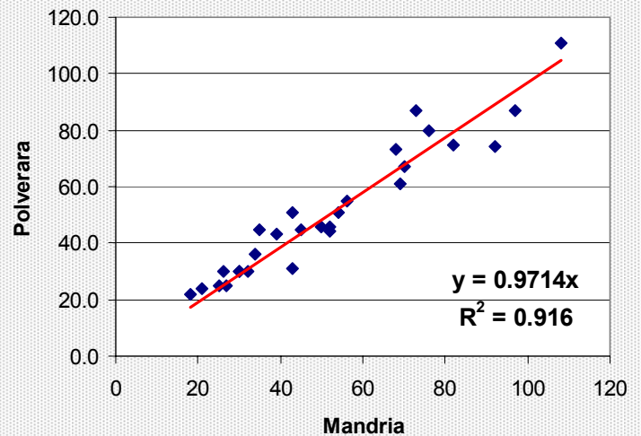
Correlazione Mandria - Polverara
