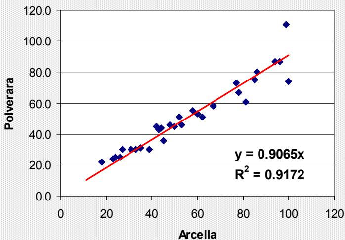
Correlazione Arcella - Polverara
