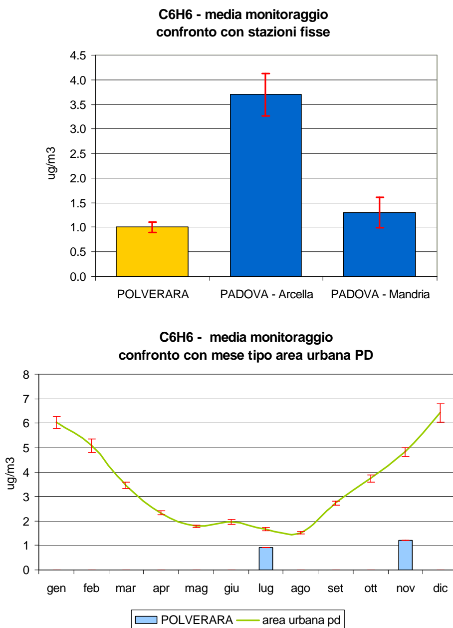
Figura 2.7 Benzene (C 6 H 6 ): concentrazione media rilevata durante il monitoraggio dal 16/06/05 al 06/07/05 e dal 26/10/05 al 10/11/05 nel Comune di Polverara; confronto con i periodi corrispondenti presso le stazioni fisse di Arcella e Mandria nel Comune di Padova e con l'andamento caratteristico del 'mese tipo' ricavato dalla serie storica nell'area urbana di Padova; le barre indicano l'errore standard della media.
