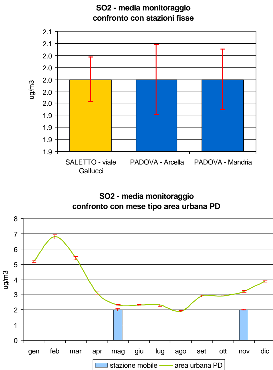
Figura 2.1 Biossido di zolfo (SO 2 ): concentrazione media rilevata durante il monitoraggio dal 05/05/06 al 24/05/06 e dal 18/10/06 al 08/11/06 in Via Gallucci nel Comune di Saletto; confronto con i periodi corrispondenti presso la stazioni fissa di Arcella e di Mandria nel Comune di Padova e con l'andamento caratteristico del 'mese tipo' ricavato dalla serie storica nell'area urbana di Padova; le barre indicano l'errore standard della media.
