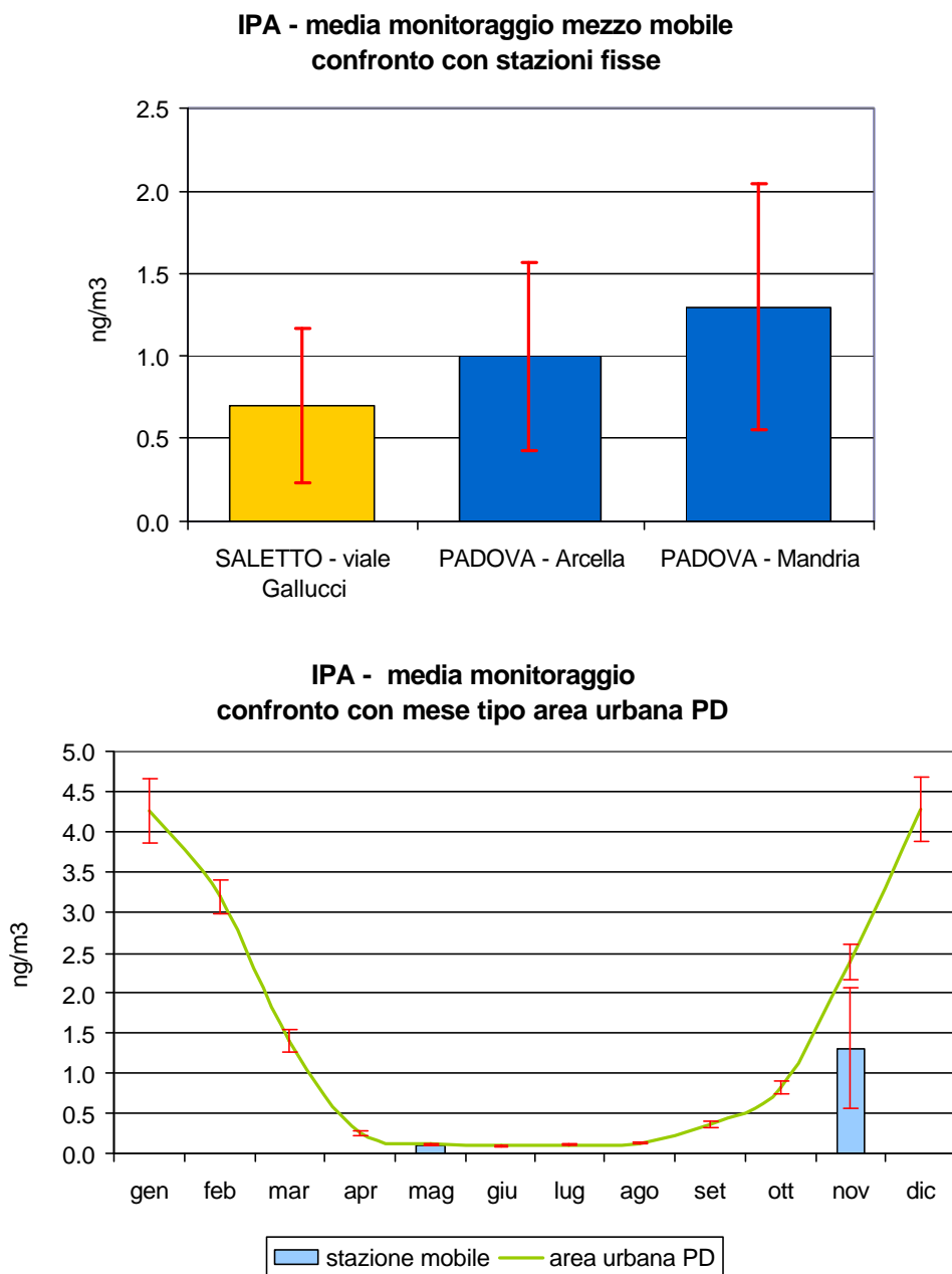
Figura 2.6 Benzo(a)pirene (IPA): concentrazione media rilevata durante il monitoraggio dal 05/05/06 al 24/05/06 e dal 18/10/06 al 08/11/06 in Via Gallucci nel Comune di Saletto; confronto con i periodi corrispondenti presso le stazioni fisse di Arcella e Mandria nel Comune di Padova e con l'andamento caratteristico del 'mese tipo' ricavato dalla serie storica nell'area urbana di Padova; le barre indicano l'errore standard della media.
