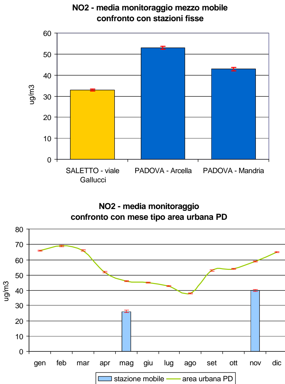
Figura 2.4 Biossido di azoto (NO 2 ): concentrazione media rilevata durante il monitoraggio dal 05/05/06 al 24/05/06 e dal 18/10/06 al 08/11/06 in Via Gallucci nel Comune di Saletto; confronto con i periodi corrispondenti presso le stazioni fisse di Arcella e Mandria nel Comune di Padova e con l'andamento caratteristico del 'mese tipo' ricavato dalla serie storica nell'area urbana di Padova; le barre indicano l'errore standard della media.
