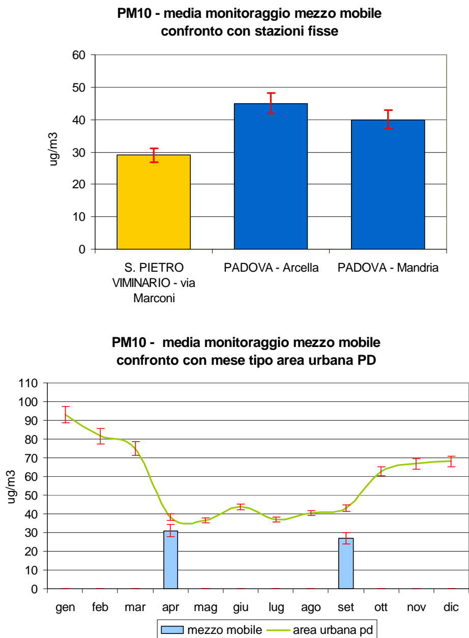
Figura 2.5 Polveri fini ( PM_{10} ): concentrazione media rilevata durante il monitoraggio dal 01/04/05 al 20/04/05 e dal 31/08/05 al 21/09/05 in Via Marconi nel Comune di San Pietro Viminario; confronto con i periodi corrispondenti presso le stazioni fisse di Arcella e Mandria nel Comune di Padova e con l'andamento caratteristico del 'mese tipo' ricavato dalla serie storica nell'area urbana di Padova; per i valori di concentrazione mensile le barre indicano l'errore standard della media.
