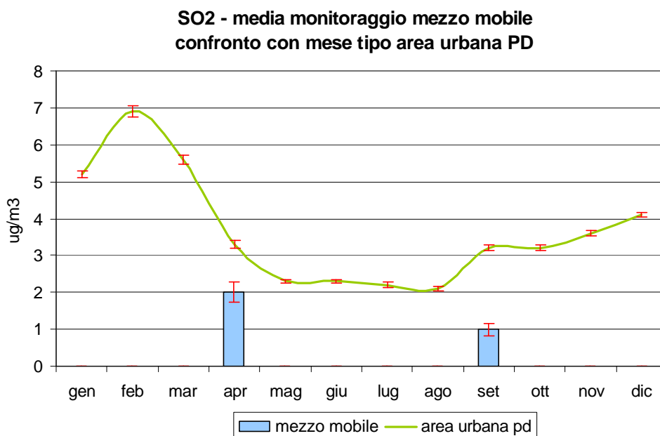
Figura 2.1 Biossido di zolfo (SO 2 ): concentrazione media rilevata durante il monitoraggio dal 01/04/05 al 20/04/05 e dal 31/08/05 al 21/09/05 in Via Marconi nel Comune di San Pietro Viminario; confronto con i periodi corrispondenti presso la stazioni fissa di Arcella e di Mandria nel Comune di Padova e con l'andamento caratteristico del 'mese tipo' ricavato dalla serie storica nell'area urbana di Padova; le barre indicano l'errore standard della media.
