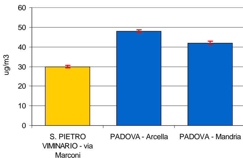
NO 2 - media monitoraggio mezzo mobile confronto con stazioni fisse
