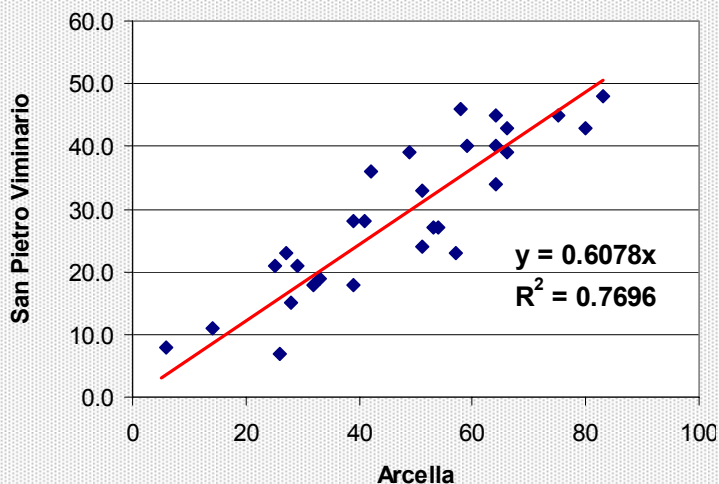
Correlazione Arcella - San Pietro Viminario
