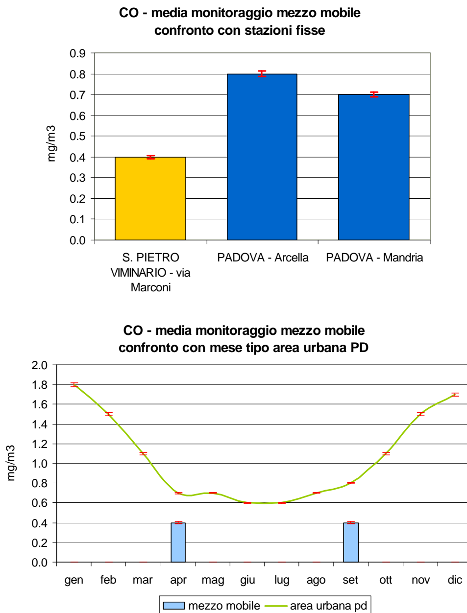
Figura 2.2 Monossido di carbonio (CO): concentrazione media rilevata durante il monitoraggio dal 01/04/05 al 20/04/05 e dal 31/08/05 al 21/09/05 in Via Marconi nel Comune di San Pietro Viminario; confronto con i periodi corrispondenti presso le stazioni fisse di Arcella e Mandria nel Comune di Padova e con l'andamento caratteristico del 'mese tipo' ricavato dalla serie storica nell'area urbana di Padova; le barre indicano l'errore standard della media.
