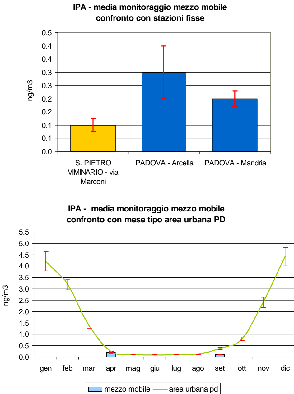
Figura 2.6 Benzo(a)pirene (IPA): concentrazione media rilevata durante il monitoraggio dal 01/04/05 al 20/04/05 e dal 31/08/05 al 21/09/05 in Via Marconi nel Comune di San Pietro Viminario; confronto con i periodi corrispondenti presso le stazioni fisse di Arcella e Mandria nel Comune di Padova e con l'andamento caratteristico del 'mese tipo' ricavato dalla serie storica nell'area urbana di Padova; le barre indicano l'errore standard della media.
