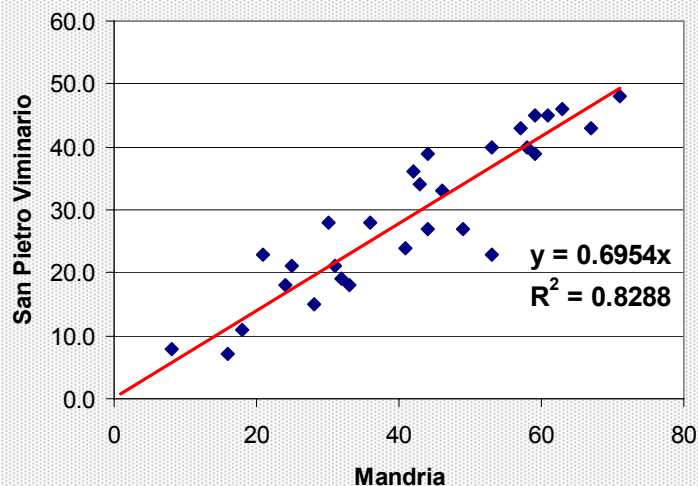
Correlazione Mandria - San Pietro Viminario
