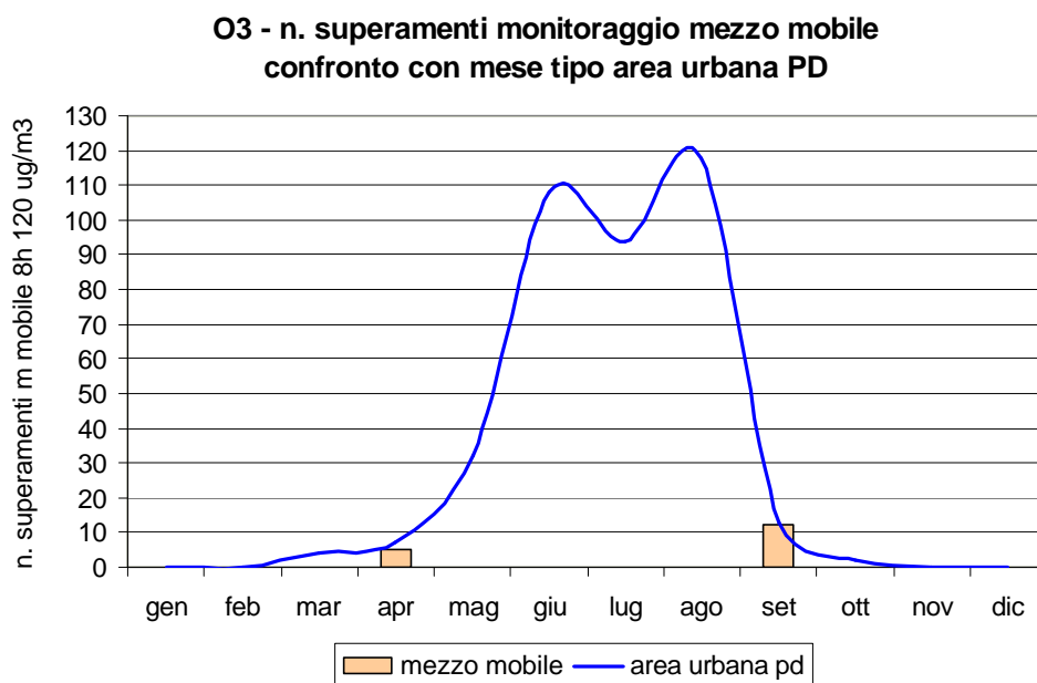
Figura 2.3 Ozono ( O_3 ): concentrazione media e numero di superamenti rilevati durante il monitoraggio dal 01/04/05 al 20/04/05 e dal 31/08/05 al 21/09/05 in Via Marconi nel Comune di San Pietro Viminario; confronto con i periodi corrispondenti presso le stazioni fisse di Arcella e Mandria nel Comune di Padova e con l'andamento caratteristico del 'mese tipo' ricavato dalla serie storica nell'area urbana di Padova; per i valori di concentrazione mensile le barre indicano l'errore standard della media.
