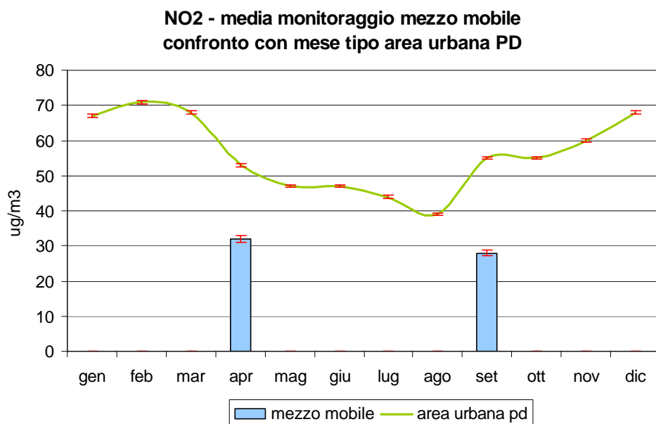
Figura 2.4 Biossido di azoto (NO 2 ): concentrazione media rilevata durante il monitoraggio dal 01/04/05 al 20/04/05 e dal 31/08/05 al 21/09/05 in Via Marconi nel Comune di San Pietro Viminario; confronto con i periodi corrispondenti presso le stazioni fisse di Arcella e Mandria nel Comune di Padova e con l'andamento caratteristico del 'mese tipo' ricavato dalla serie storica nell'area urbana di Padova; le barre indicano l'errore standard della media.
