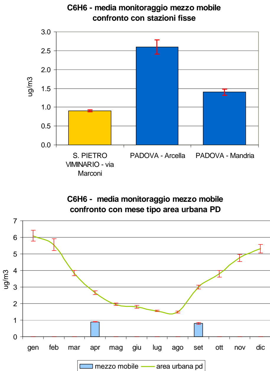
Figura 2.7 Benzene (C 6 H 6 ): concentrazione media rilevata durante il monitoraggio dal 01/04/05 al 20/04/05 e dal 31/08/05 al 21/09/05 in Via Marconi nel Comune di San Pietro Viminario; confronto con i periodi corrispondenti presso le stazioni fisse di Arcella e Mandria nel Comune di Padova e con l'andamento caratteristico del 'mese tipo' ricavato dalla serie storica nell'area urbana di Padova; le barre indicano l'errore standard della media.
