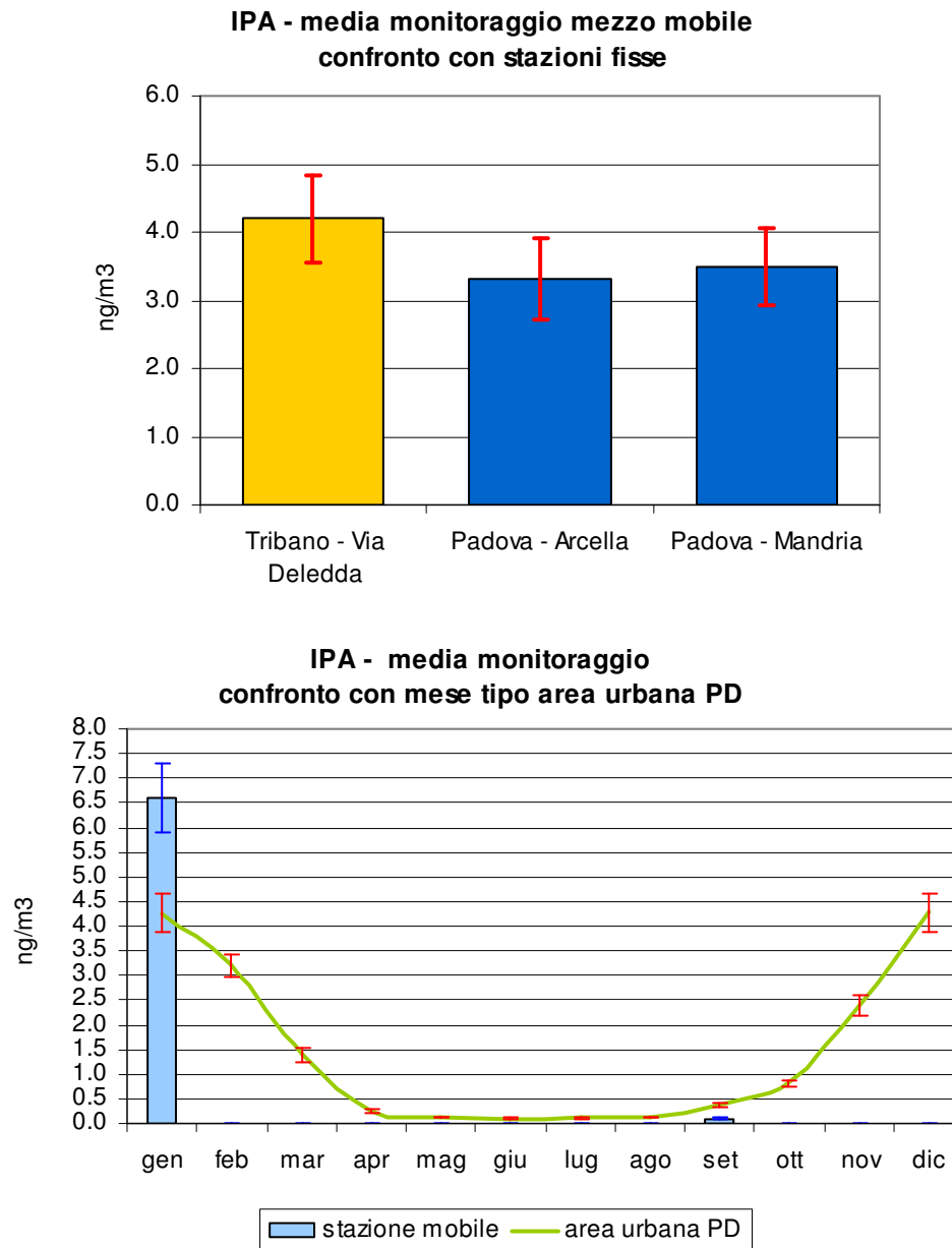
Figura 2.6 Benzo(a)pirene (IPA): concentrazione media rilevata durante il monitoraggio dal 23/08/07 al 26/09/07 e dal 28/11/07 al 28/01/08 in Via Deledda nel Comune di Tribano; confronto con i periodi corrispondenti presso le stazioni fisse di Arcella e Mandria nel Comune di Padova e con l'andamento caratteristico del 'mese tipo' ricavato dalla serie storica nell'area urbana di Padova; le barre indicano l'errore standard della media.
