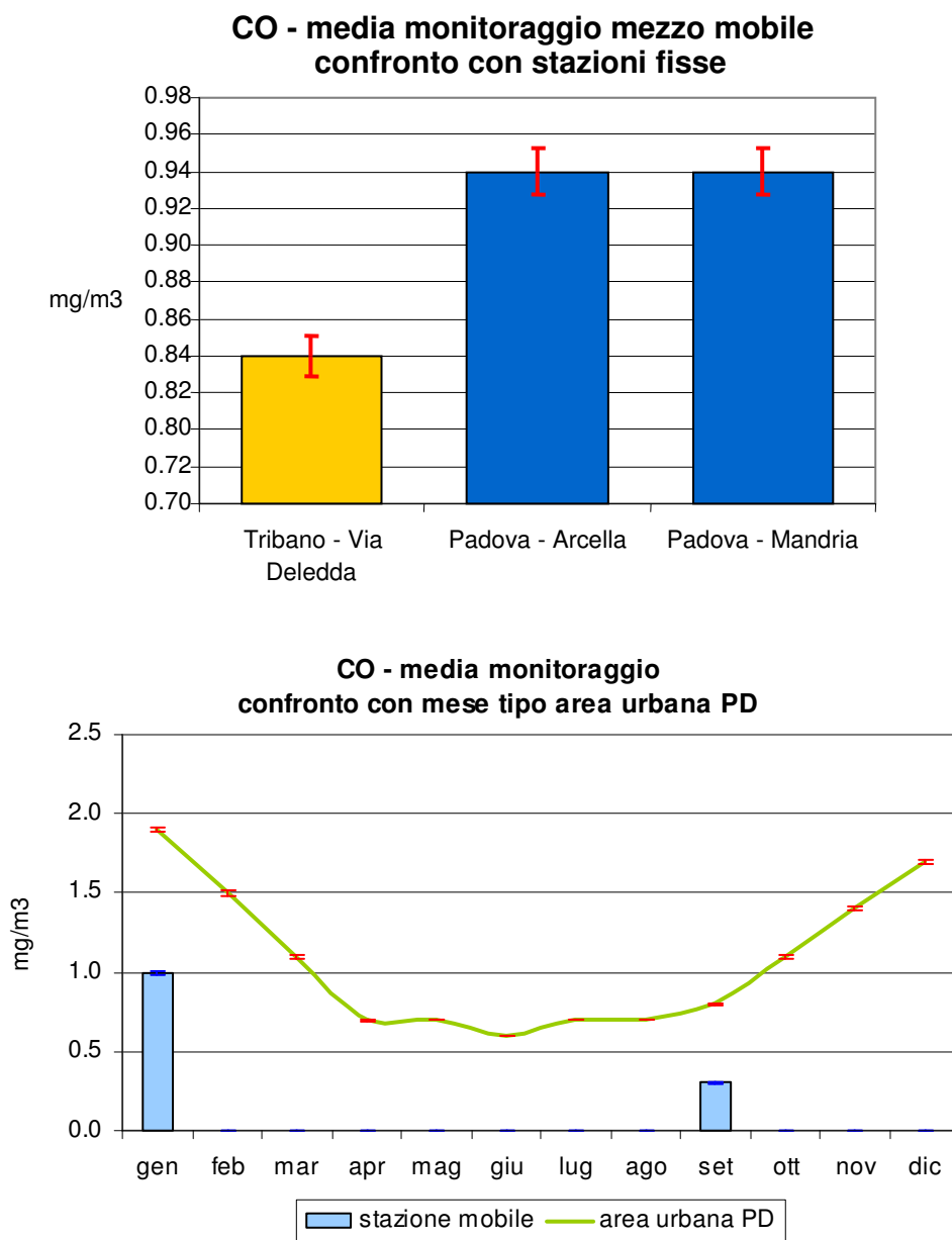
Figura 2.2 Monossido di carbonio (CO): concentrazione media rilevata durante il monitoraggio dal 23/08/07 al 26/09/07 e dal 28/11/07 al 28/01/08 in Via Deledda nel Comune di Tribano; confronto con i periodi corrispondenti presso le stazioni fisse di Arcella e Mandria nel Comune di Padova e con l'andamento caratteristico del 'mese tipo' ricavato dalla serie storica nell'area urbana di Padova; le barre indicano l'errore standard della media.
