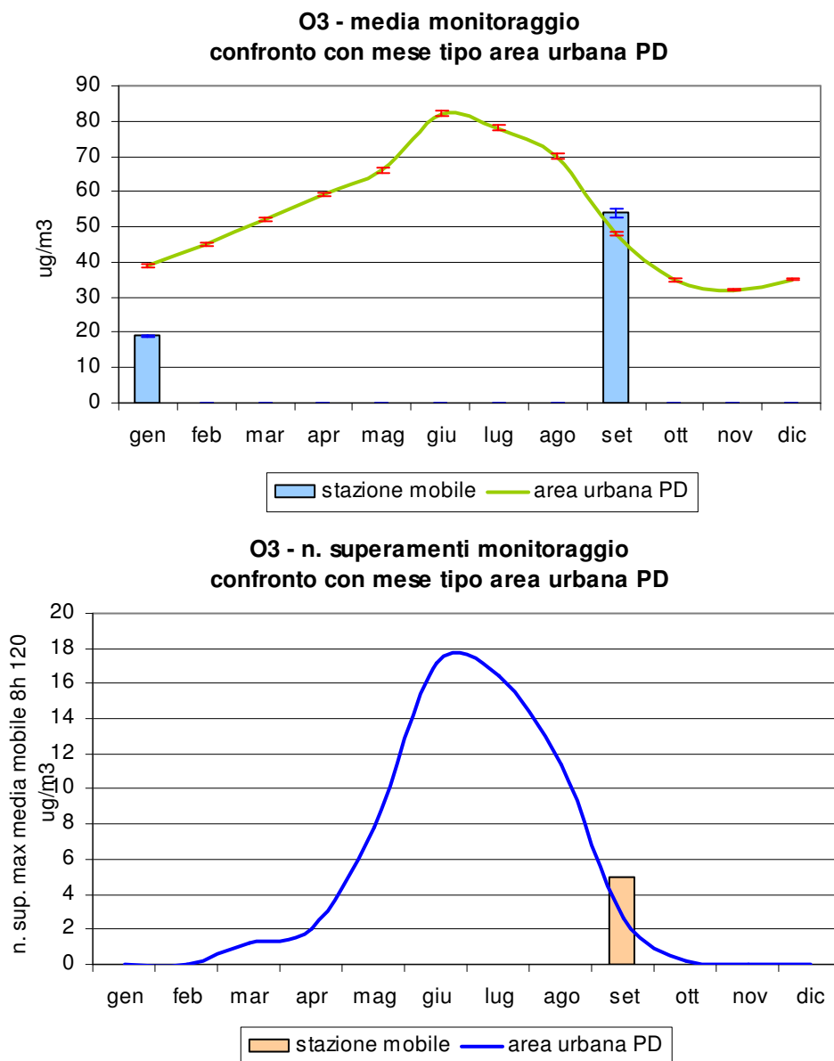
Figura 2.3 Ozono (O 3 ): concentrazione media e numero di superamenti rilevati durante il monitoraggio dal 23/08/07 al 26/09/07 e dal 28/11/07 al 28/01/08 in Via Deledda nel Comune di Tribano; confronto con i periodi corrispondenti presso le stazioni fisse di Arcella e Mandria nel Comune di Padova e con l'andamento caratteristico del 'mese tipo' ricavato dalla serie storica nell'area urbana di Padova; per i valori di concentrazione mensile le barre indicano l'errore standard della media.
