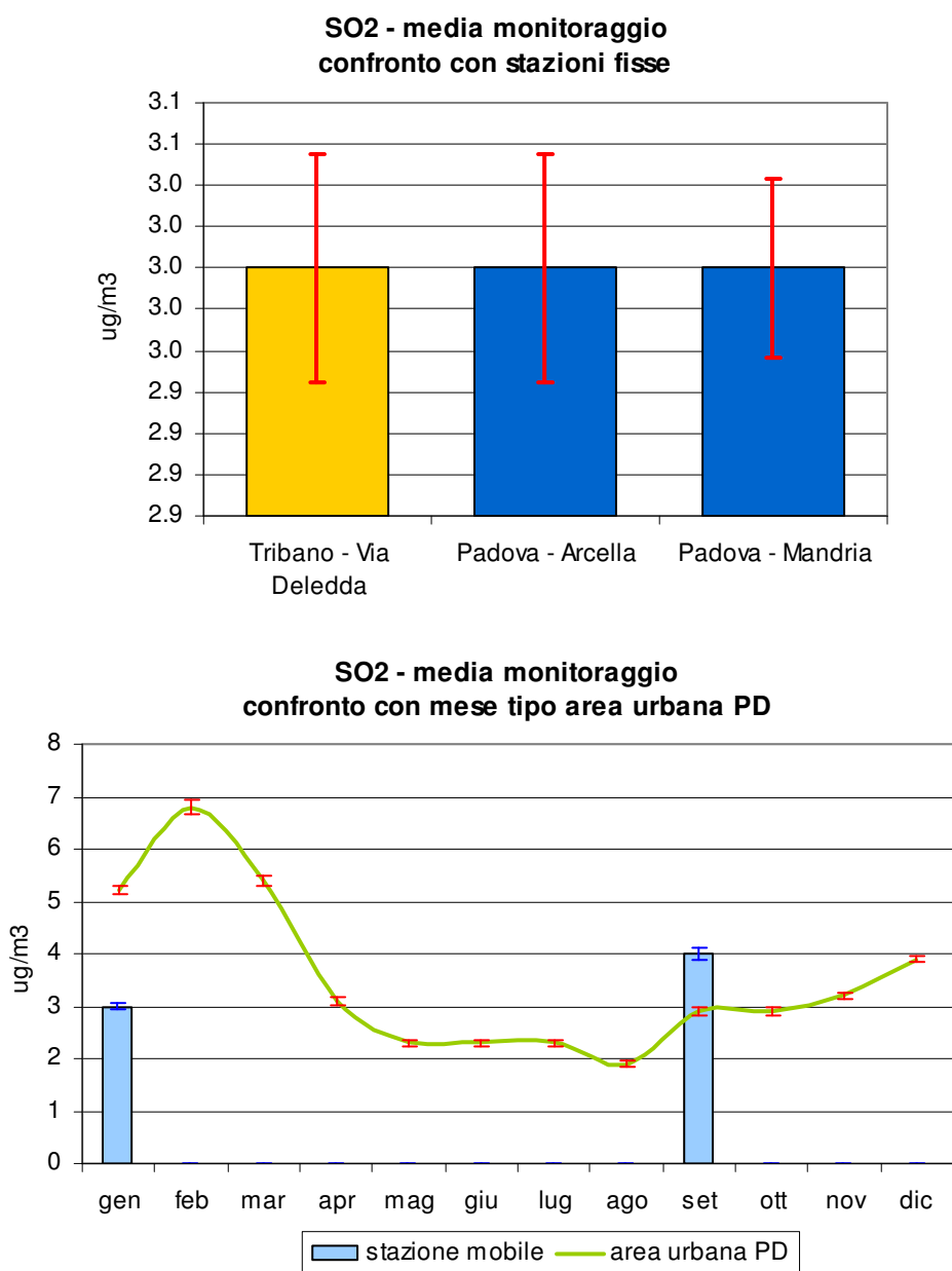
Figura 2.1 Biossido di zolfo (SO 2 ): concentrazione media rilevata durante il monitoraggio dal 23/08/07 al 26/09/07 e dal 28/11/07 al 28/01/08 in Via Deledda nel Comune di Tribano; confronto con i periodi corrispondenti presso la stazioni fissa di Arcella e di Mandria nel Comune di Padova e con l'andamento caratteristico del 'mese tipo' ricavato dalla serie storica nell'area urbana di Padova; le barre indicano l'errore standard della media.
