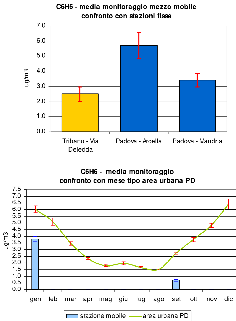
Figura 2.7 Benzene (C 6 H 6 ): concentrazione media rilevata durante il monitoraggio dal 23/08/07 al 26/09/07 e dal 28/11/07 al 28/01/08 in Via Deledda nel Comune di Tribano; confronto con i periodi corrispondenti presso le stazioni fisse di Arcella e Mandria nel Comune di Padova e con l'andamento caratteristico del 'mese tipo' ricavato dalla serie storica nell'area urbana di Padova; le barre indicano l'errore standard della media.
