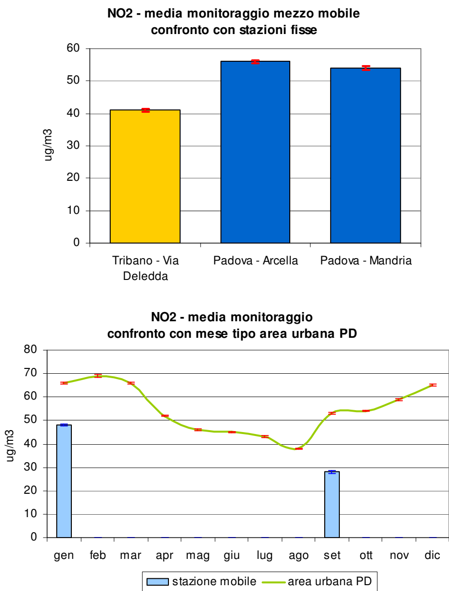
Figura 2.4 Biossido di azoto (NO 2 ): concentrazione media rilevata durante il monitoraggio dal 23/08/07 al 26/09/07 e dal 28/11/07 al 28/01/08 in Via Deledda nel Comune di Tribano; confronto con i periodi corrispondenti presso le stazioni fisse di Arcella e Mandria nel Comune di Padova e con l'andamento caratteristico del 'mese tipo' ricavato dalla serie storica nell'area urbana di Padova; le barre indicano l'errore standard della media.
