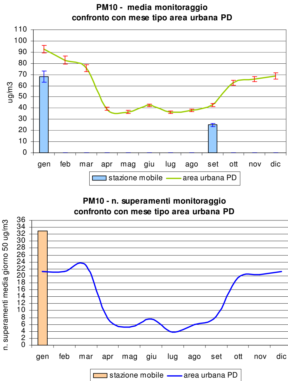
Figura 2.5 Polveri fini ( PM_{10} ): concentrazione media e numero di superamenti rilevati durante il monitoraggio dal 23/08/07 al 26/09/07 e dal 28/11/07 al 28/01/08 in Via Deledda nel Comune di Tribano; confronto con i periodi corrispondenti presso le stazioni fisse di Arcella e Mandria nel Comune di Padova e con l'andamento caratteristico del 'mese tipo' ricavato dalla serie storica nell'area urbana di Padova; per i valori di concentrazione mensile le barre indicano l'errore standard della media.
