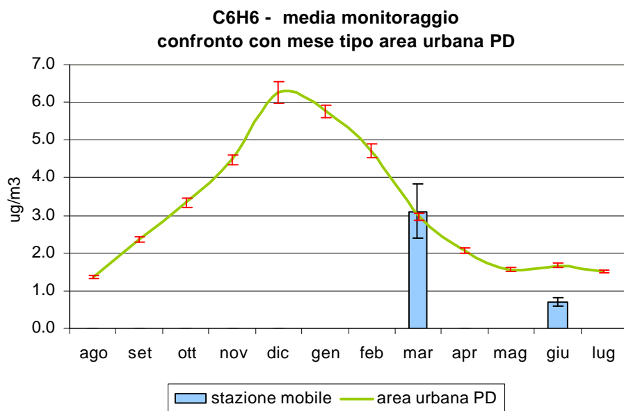
Figura 3.7 Benzene (C 6 H 6 ): confronto delle concentrazioni medie rilevate durante il monitoraggio in Via L. da Vinci nel Comune di Vigodarzere con l'andamento caratteristico del 'mese tipo' ricavato dalla serie storica nell'area urbana di Padova; le barre indicano l'errore standard della media.
