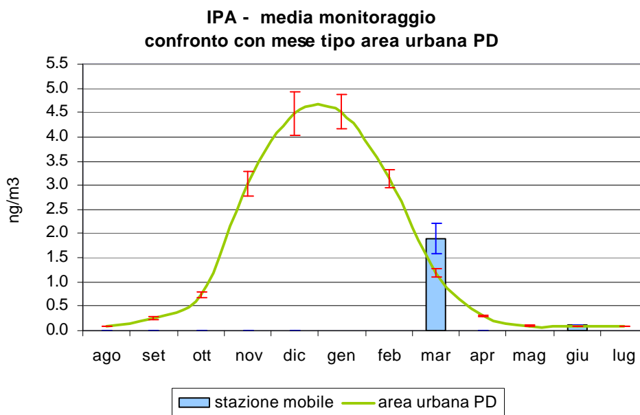
Figura 3.6 Benzo(a)pirene (IPA): confronto delle concentrazioni medie rilevate durante il monitoraggio in Via L. da Vinci nel Comune di Vigodarzere con l'andamento caratteristico del 'mese tipo' ricavato dalla serie storica nell'area urbana di Padova; le barre indicano l'errore standard della media.
