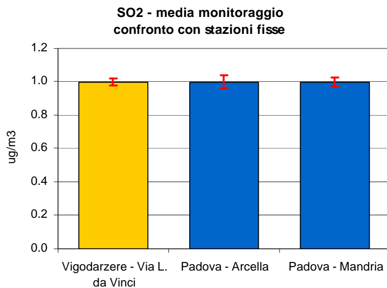
Figura 2.1 Biossido di zolfo (SO 2 ): concentrazione media rilevata durante il monitoraggio dal 24/02/09 al 30/03/09 e dal 06/06/09 al 08/07/09 in Via L. da Vinci nel Comune di Vigodarzere e confronto con i periodi corrispondenti presso le stazioni fisse di Arcella e di Mandria; le barre indicano l'errore standard della media.
