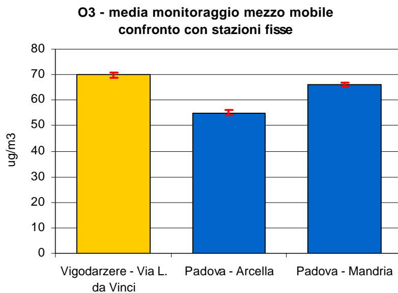
Figura 2.3 Ozono ( O_3 ): concentrazione media rilevata durante il monitoraggio in Via L. da Vinci nel Comune di Vigodarzere e confronto con i periodi corrispondenti presso le stazioni fisse di Arcella e Mandria; le barre indicano l'errore standard della media.
