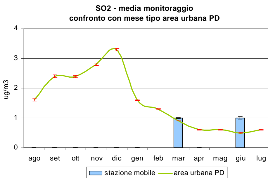
Figura 3.1 Biossido di zolfo (SO 2 ): confronto delle concentrazioni medie rilevate durante il monitoraggio in Via L. da Vinci nel Comune di Vigodarzere con l’andamento caratteristico del ‘mese tipo’ ricavato dalla serie storica nell’area urbana di Padova; le barre indicano l’errore standard della media.
