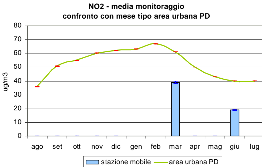
Figura 3.3 Biossido di azoto (NO 2 ): confronto delle concentrazioni medie rilevate durante il monitoraggio in Via L. da Vinci nel Comune di Vigodarzere con l'andamento caratteristico del 'mese tipo' ricavato dalla serie storica nell'area urbana di Padova; le barre indicano l'errore standard della media.
