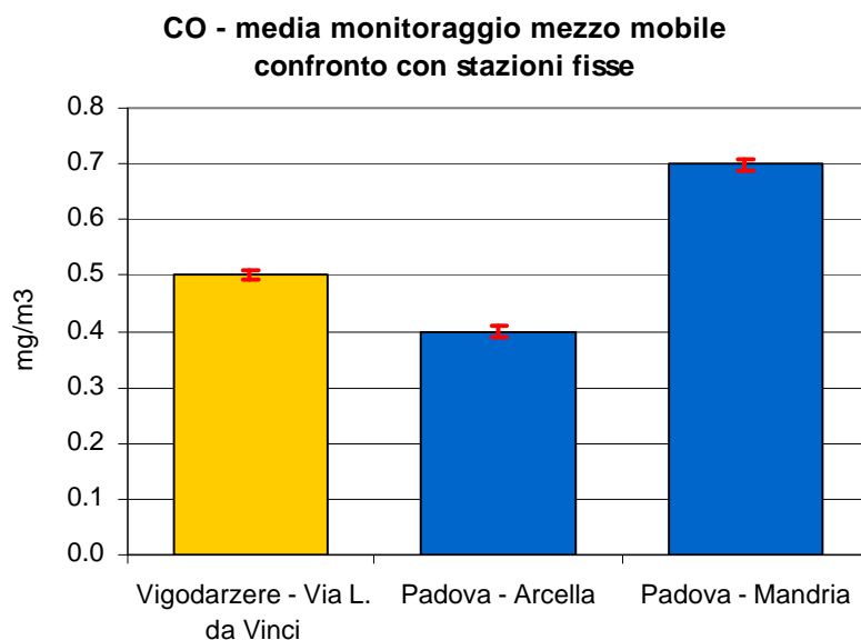
Figura 2.2 Monossido di carbonio (CO): concentrazione media rilevata durante il monitoraggio dal 24/02/09 al 30/03/09 e dal 06/06/09 al 08/07/09 in Via L. da Vinci nel Comune di Vigodarzere e confronto con i periodi corrispondenti presso le stazioni fisse di Arcella e Mandria; le barre indicano l'errore standard della media.
