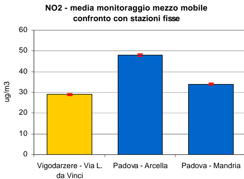
Figura 2.4 Biossido di azoto (NO 2 ): concentrazione media rilevata durante il monitoraggio dal 24/02/09 al 30/03/09 e dal 06/06/09 al 08/07/09 in Via L. da Vinci nel Comune di Vigodarzere e confronto con i periodi corrispondenti presso le stazioni fisse di Arcella e Mandria; le barre indicano l'errore standard della media.
