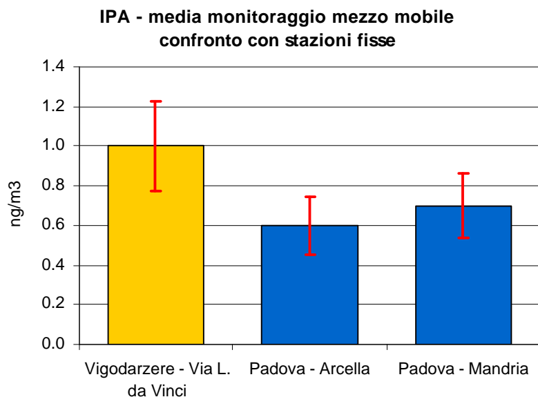
Figura 2.6 Benzo(a)pirene (IPA): concentrazione media rilevata durante il monitoraggio dal 24/02/09 al 30/03/09 e dal 06/06/09 al 08/07/09 in Via L. da Vinci nel Comune di Vigodarzere e confronto con i periodi corrispondenti presso le stazioni fisse di Arcella e Mandria nel Comune di Padova; le barre indicano l'errore standard della media.
