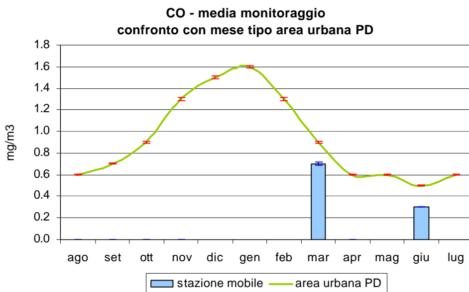
Figura 3.2 Monossido di carbonio (CO): concentrazione media rilevata durante il monitoraggio in Via L. da Vinci nel Comune di Vigodarzere con l'andamento caratteristico del 'mese tipo' ricavato dalla serie storica nell'area urbana di Padova; le barre indicano l'errore standard della media.
