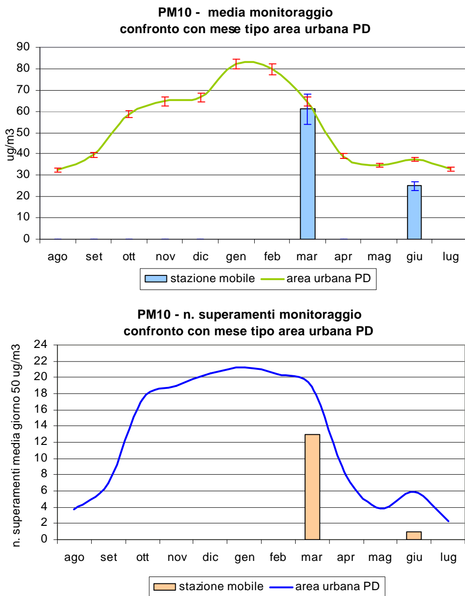
Figura 3.5 Polveri fini (PM 10 ): confronto delle concentrazioni medie e del numero di superamenti del valore limite di protezione della salute (50 \mu\text{g}/\text{m}^3 ) rilevati durante il monitoraggio in Via L. da Vinci nel Comune di Vigodarzere con l'andamento caratteristico del 'mese tipo' ricavato dalla serie storica nell'area urbana di Padova; per i valori di concentrazione mensile le barre indicano l'errore standard della media.
