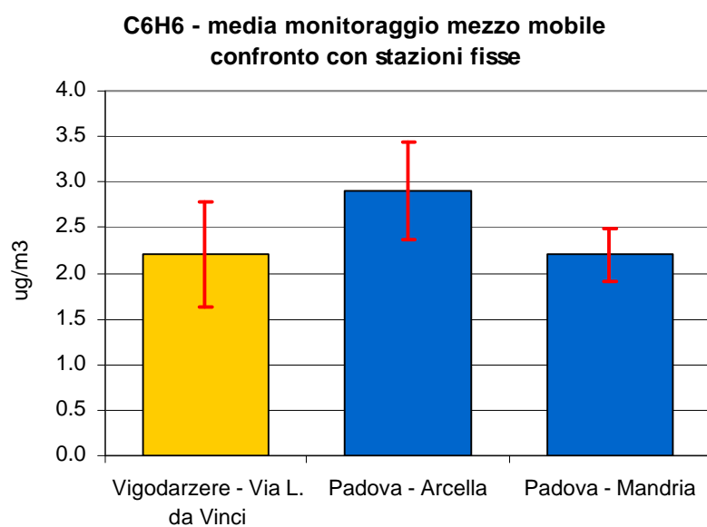
Figura 2.7 Benzene (C 6 H 6 ): concentrazione media rilevata durante il monitoraggio in Via L. da Vinci nel Comune di Vigodarzere e confronto con i periodi corrispondenti presso le stazioni fisse di Arcella e Mandria nel Comune di Padova; le barre indicano l'errore standard della media.
