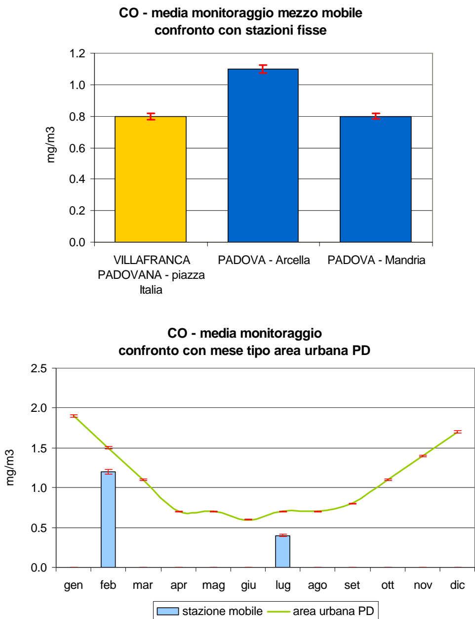
Figura 2.2 Monossido di carbonio (CO): concentrazione media rilevata durante il monitoraggio dal 10/01/06 al 01/02/06 e dal 05/07/06 al 26/07/06 in Piazza Italia nel Comune di Villafranca Padovana; confronto con i periodi corrispondenti presso le stazioni fisse di Arcella e Mandria nel Comune di Padova e con l'andamento caratteristico del 'mese tipo' ricavato dalla serie storica nell'area urbana di Padova; le barre indicano l'errore standard della media.
