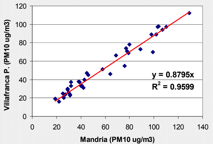
Correlazione Mandria - Villafranca P.
