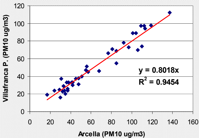
Correlazione Arcella - Villafranca P.
