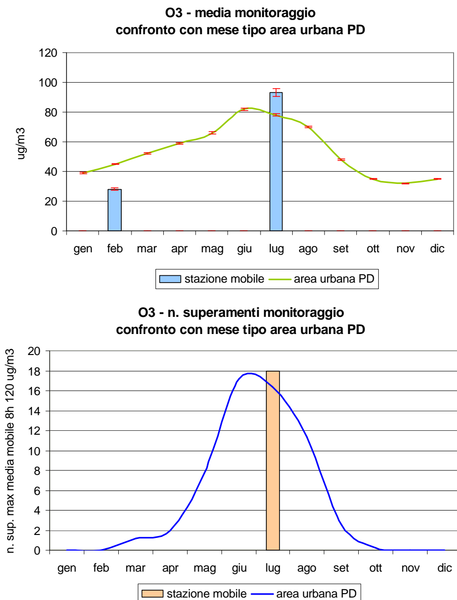
Figura 2.3 Ozono (O 3 ): concentrazione media e numero di superamenti rilevati durante il monitoraggio dal 10/01/06 al 01/02/06 e dal 05/07/06 al 26/07/06 in Piazza Italia nel Comune di Villafranca Padovana; confronto con i periodi corrispondenti presso le stazioni fisse di Arcella e Mandria nel Comune di Padova e con l'andamento caratteristico del 'mese tipo' ricavato dalla serie storica nell'area urbana di Padova; per i valori di concentrazione mensile le barre indicano l'errore standard della media.
