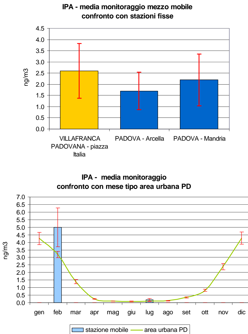
Figura 2.6 Benzo(a)pirene (IPA): concentrazione media rilevata durante il monitoraggio dal 10/01/06 al 01/02/06 e dal 05/07/06 al 26/07/06 in Piazza Italia nel Comune di Villafranca Padovana; confronto con i periodi corrispondenti presso le stazioni fisse di Arcella e Mandria nel Comune di Padova e con l'andamento caratteristico del 'mese tipo' ricavato dalla serie storica nell'area urbana di Padova; le barre indicano l'errore standard della media.
