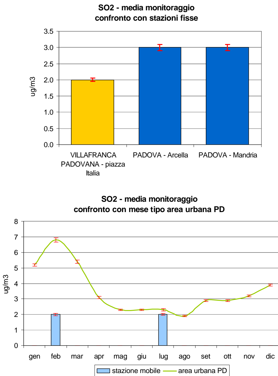
Figura 2.1 Biossido di zolfo (SO 2 ): concentrazione media rilevata durante il monitoraggio dal 10/01/06 al 01/02/06 e dal 05/07/06 al 26/07/06 in Piazza Italia nel Comune di Villafranca Padovana; confronto con i periodi corrispondenti presso la stazioni fissa di Arcella e di Mandria nel Comune di Padova e con l'andamento caratteristico del 'mese tipo' ricavato dalla serie storica nell'area urbana di Padova; le barre indicano l'errore standard della media.
