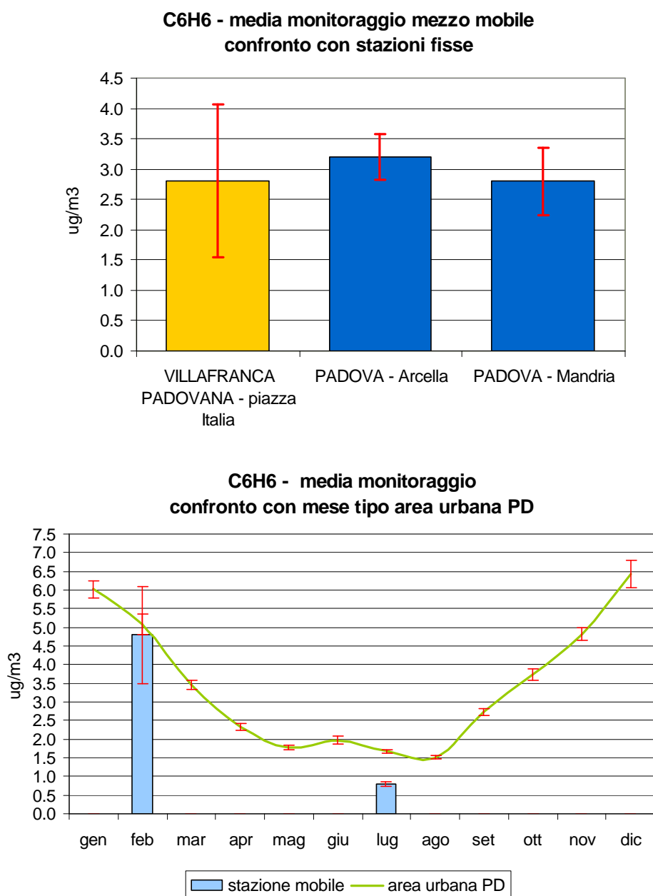
Figura 2.7 Benzene (C 6 H 6 ): concentrazione media rilevata durante il monitoraggio dal 10/01/06 al 01/02/06 e dal 05/07/06 al 26/07/06 in Piazza Italia nel Comune di Villafranca Padovana; confronto con i periodi corrispondenti presso le stazioni fisse di Arcella e Mandria nel Comune di Padova e con l'andamento caratteristico del 'mese tipo' ricavato dalla serie storica nell'area urbana di Padova; le barre indicano l'errore standard della media.
