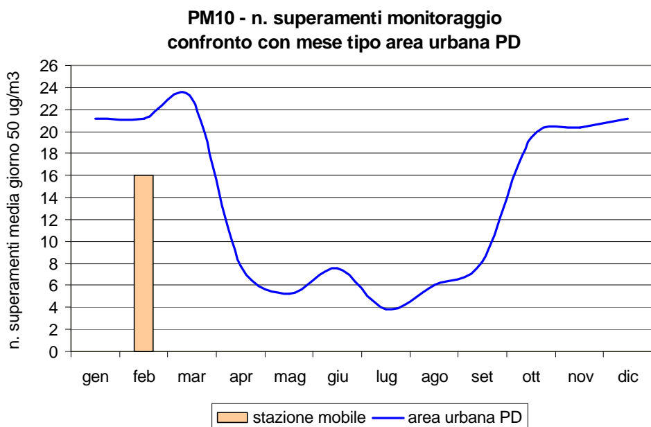
Figura 2.5 Polveri fini (PM 10 ): concentrazione media e numero di superamenti rilevati durante il monitoraggio dal 10/01/06 al 01/02/06 e dal 05/07/06 al 26/07/06 in Piazza Italia nel Comune di Villafranca Padovana; confronto con i periodi corrispondenti presso le stazioni fisse di Arcella e Mandria nel Comune di Padova e con l'andamento caratteristico del 'mese tipo' ricavato dalla serie storica nell'area urbana di Padova; per i valori di concentrazione mensile le barre indicano l'errore standard della media.
