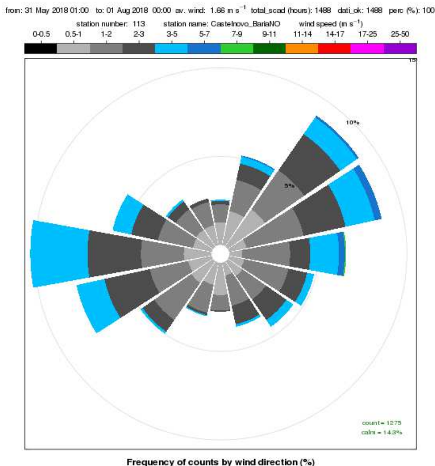
Figura 6: rosa dei venti registrati presso la stazione meteorologica di Castelnuovo Bariano (RO) nel periodo 31 maggio – 31 luglio 2018
