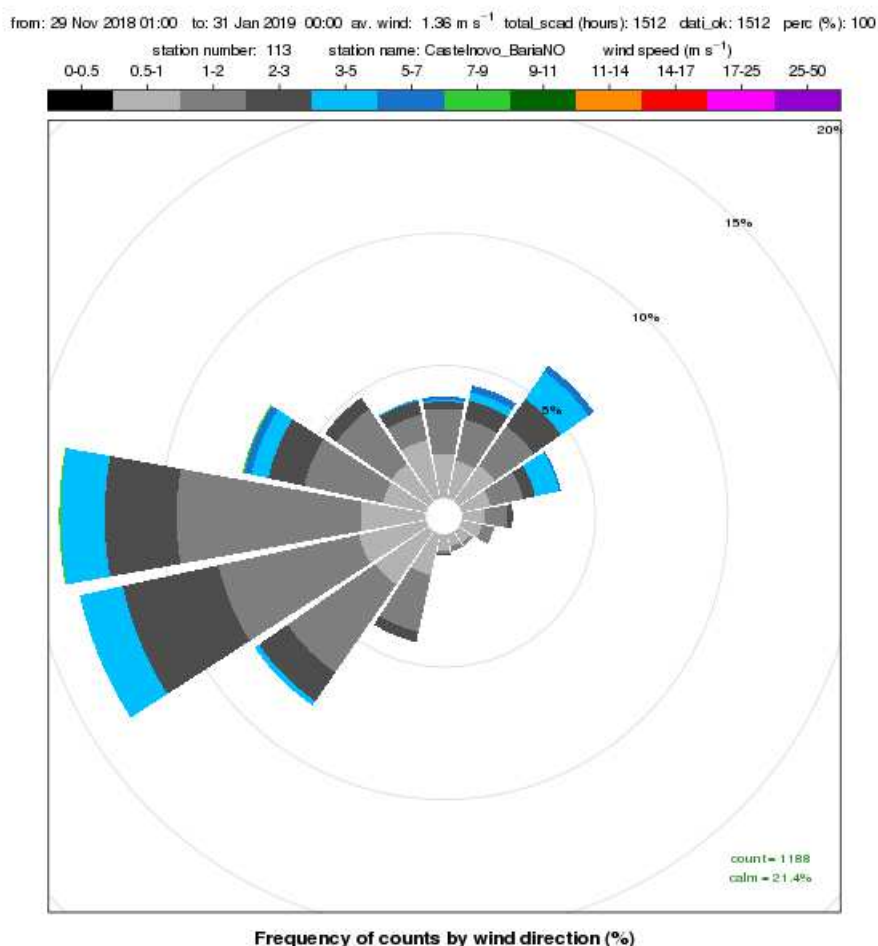
Figura 4: rosa dei venti registrati presso la stazione meteorologica di Castelnuovo Bariano (RO) nel periodo
