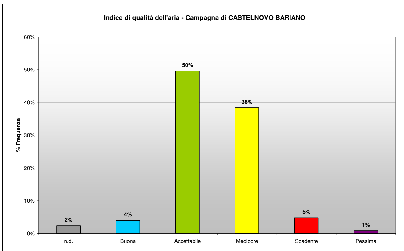
Figura 7. Calcolo dell'indice sintetico di qualità dell'aria per la campagna di Castelnuovo Bariano
