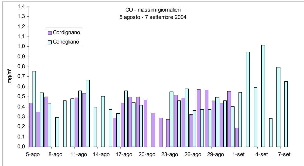
Figura 2 –Valori massimi di monossido di carbonio CO rilevati presso la stazione fissa di Conegliano e il Laboratorio Mobile posizionato a Cordignano
