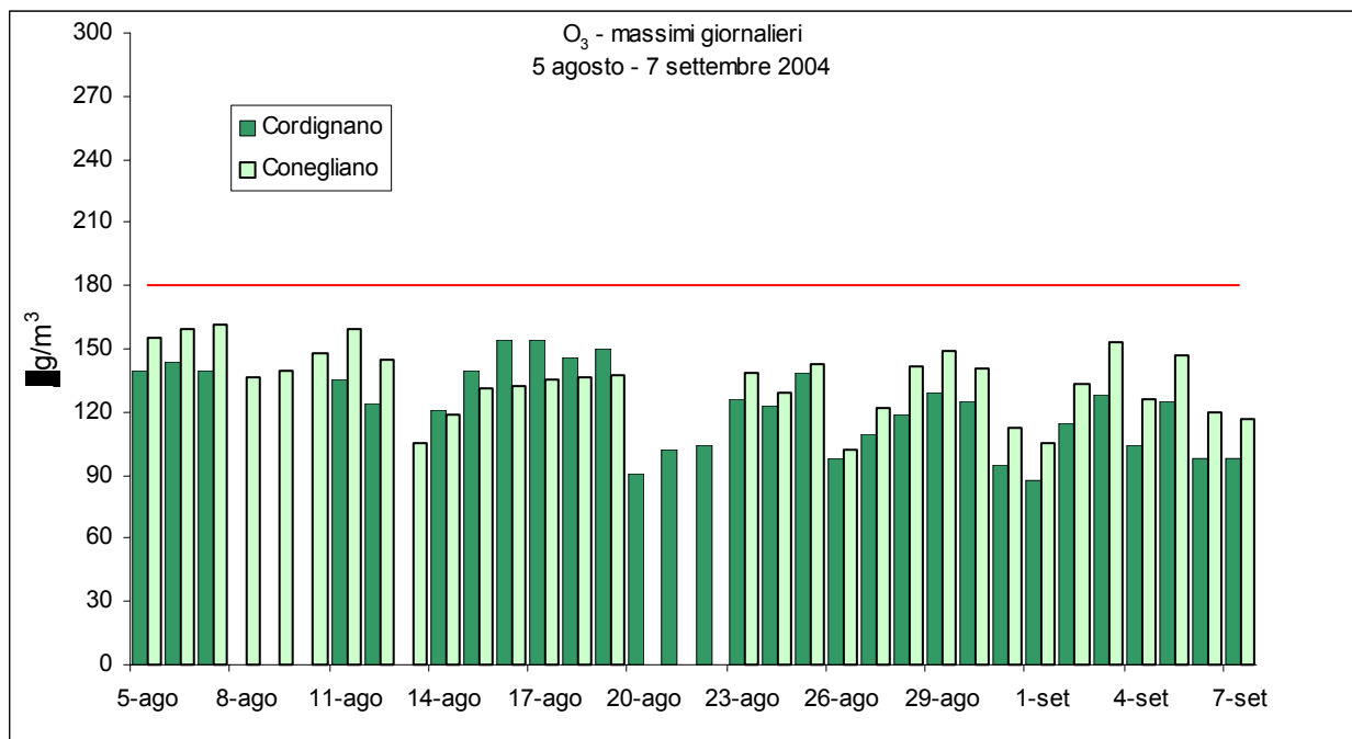
Figura 4 –Valori massimi di ozono O 3 rilevati presso la stazione fissa di Conegliano e il Laboratorio Mobile posizionato a Cordignano
