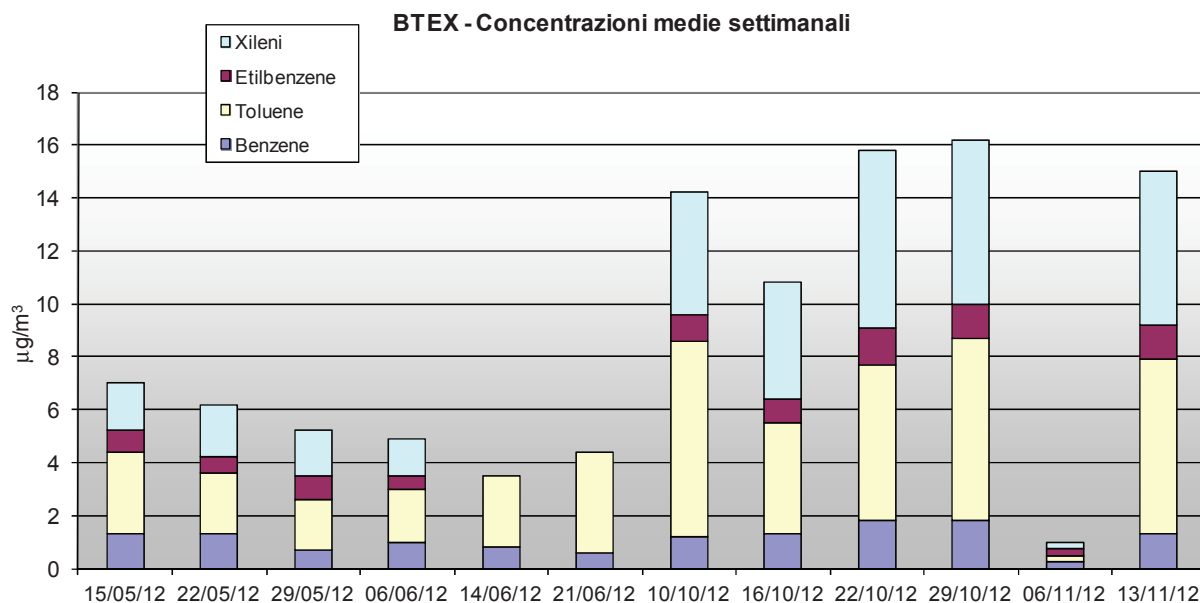
Grafico 3 Valori settimanali di BTEX (Benzene, Toluene, Etilbenzene, Xilene) rilevati a Follina. Causa problemi strumentali non sono disponibili i dati di Etilbenzene e Xileni per i campioni del 14/06/2012 e del 21/06/2012.
