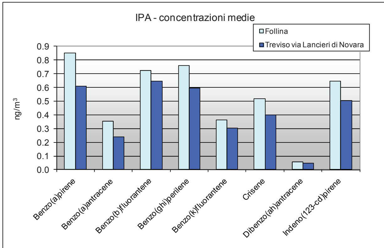
Grafico 4 Confronto tra i valori di IPA determinati su campioni di PM10 prelevati nel sito di monitoraggio e presso la stazione fissa di Treviso durante le due campagne.
