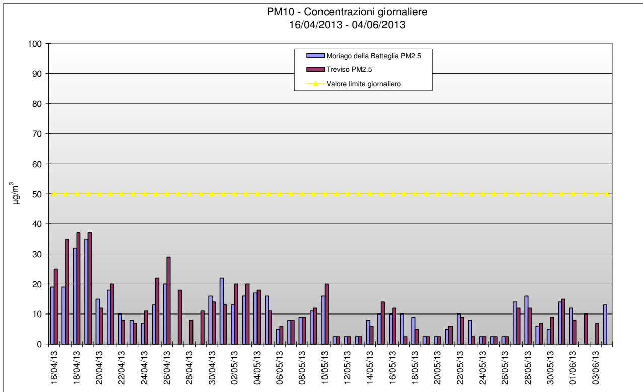
Grafico 8 – Concentrazione Giornaliera di PM2.5 ( \mu\text{g}/\text{m}^3 ).
