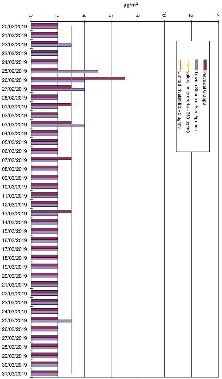
Gráfico 3 – Concentrazione Massima Giornaliera della Media Oraria di SO 2 (µg/m 3 ). Semestre "invernale"
