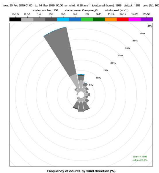
Figura 4. rosa dei venti a scansione oraria registrati presso la stazione meteorologica di Crespano del Grappa nel periodo 20 febbraio – 13 maggio 2019
