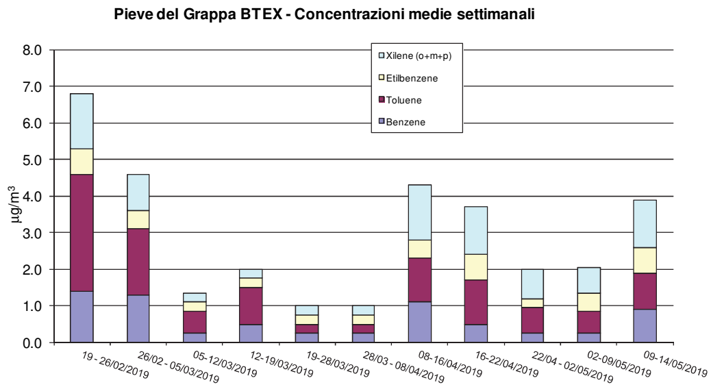
Grafico 9 Concentrazioni Medie Settimanali di BTEX.
