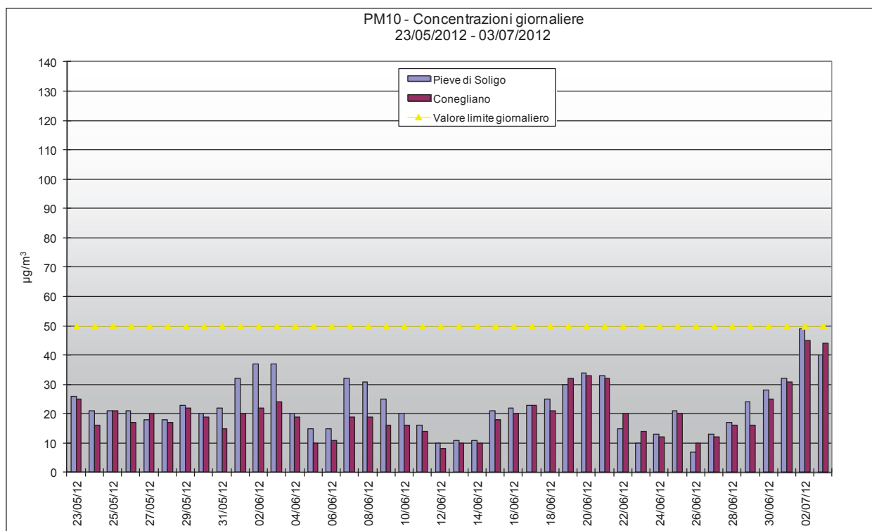
Grafico 1 Valori medi giornalieri di PM10 rilevati presso la stazione fissa di Conegliano ed il campionatore rilocabile posizionato a Pieve di Soligo – campagna estiva.
