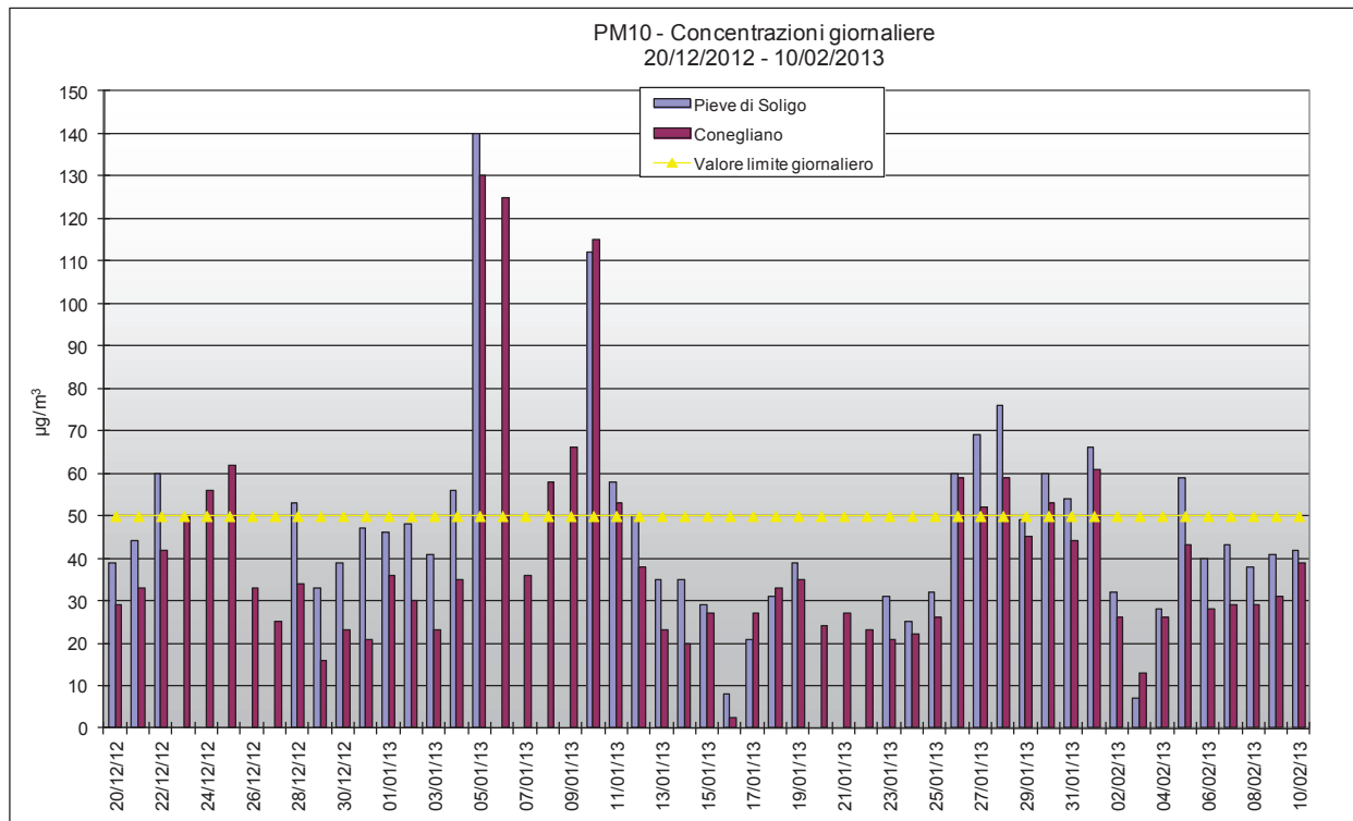
Grafico 2 Valori medi giornalieri di PM10 rilevati presso la stazione fissa di Conegliano ed il campionatore rilocabile posizionato a Pieve di Soligo – campagna invernale.
