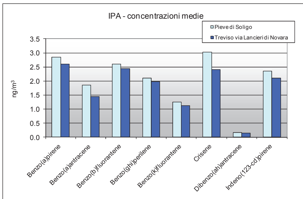
Grafico 4 Confronto tra i valori di IPA determinati su campioni di PM10 prelevati nel sito di monitoraggio e presso la stazione fissa di Treviso durante le due campagne.
