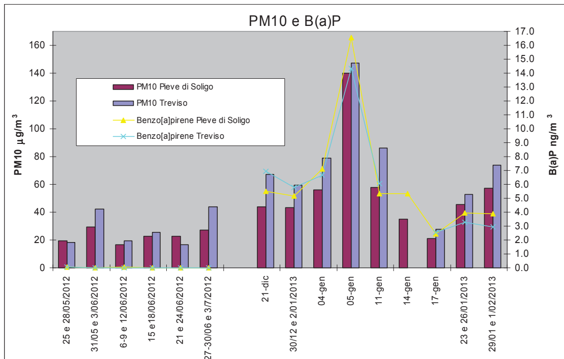
Grafico 5 Confronto tra i valori di B(a)P e PM10 prelevati nel sito di monitoraggio e presso la stazione fissa di Treviso durante le due campagne.
