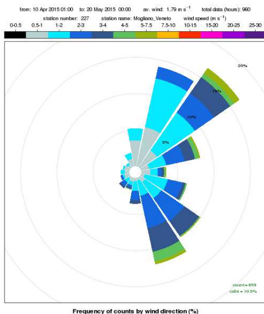
Figura 4. rosa dei venti a scansione oraria registrati presso la stazione meteorologica di Mogliano Veneto nel periodo 10 aprile – 19 maggio 2015.
