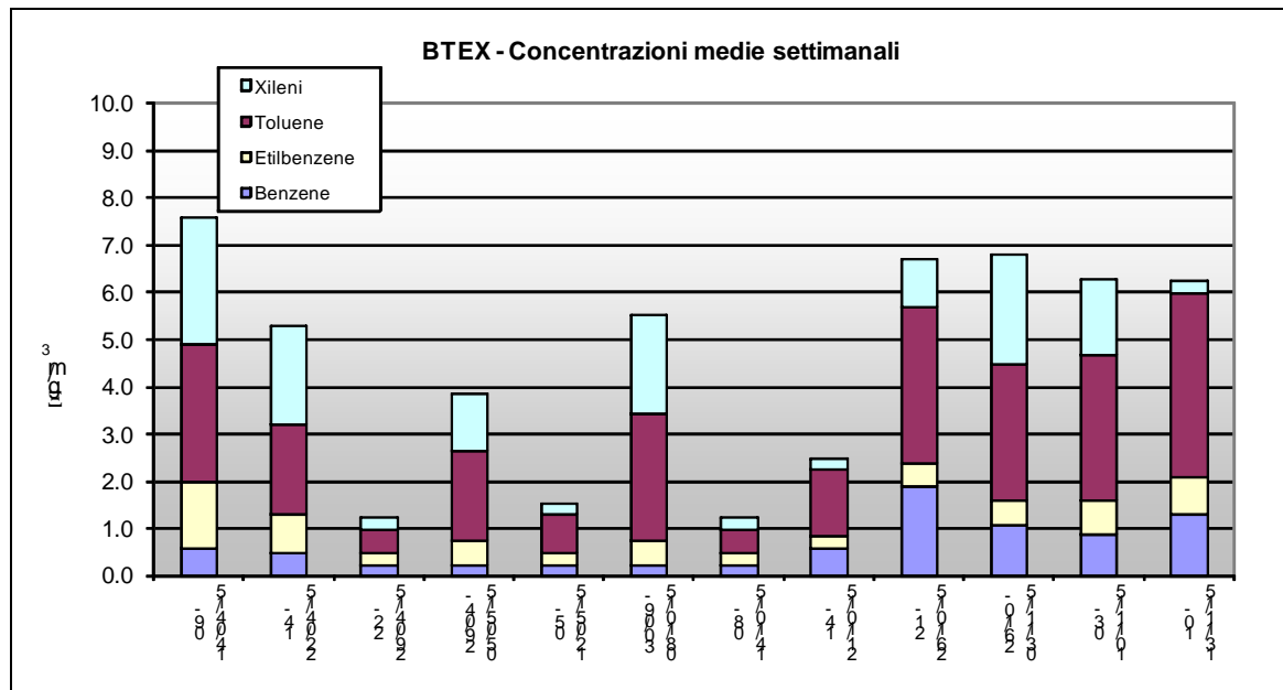
Grafico 2 - Valori settimanali di BTEX (benzene, toluene, etilbenzene e xilene) rilevati a Ponzano Veneto.
