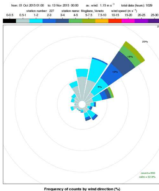
Figura 6. rosa dei venti a scansione oraria registrati presso la stazione meteorologica di Mogliano Veneto nel periodo 1 ottobre - 12 novembre 2015.
