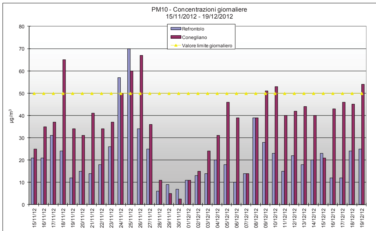
Grafico 14 Valori medi giornalieri di PM10 rilevati presso la stazione fissa di Conegliano e la stazione rilocabile posizionata a Refrontolo – campagna invernale.
