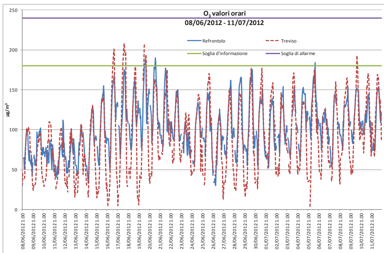
Grafico 5: Valori orari di O 3 rilevati presso la stazione fissa di Treviso e la stazione rilocabile posizionata a Refrontolo – campagna estiva.
