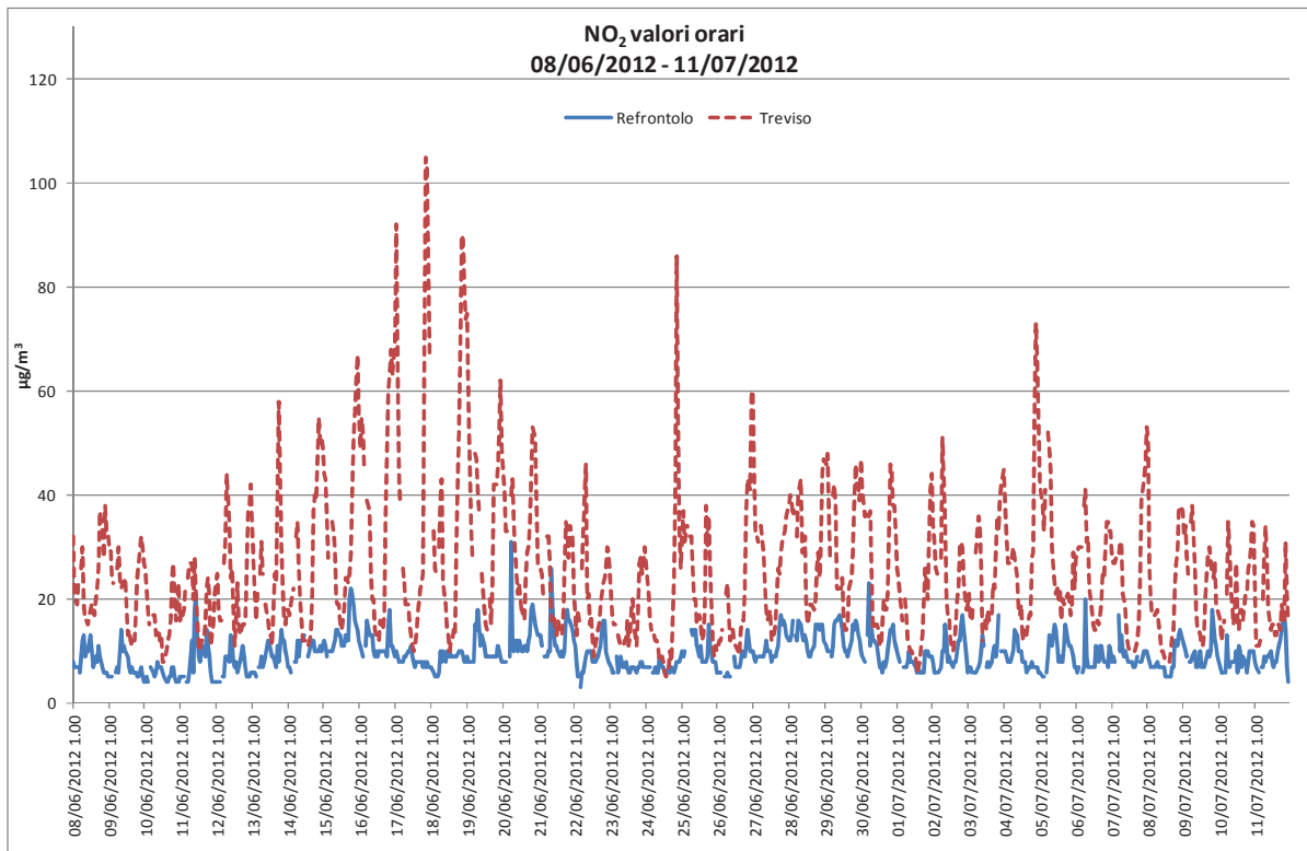
Grafico 3: Valori orari di NO 2 rilevati presso la stazione fissa di Treviso e la stazione rilocabile posizionata a Refrontolo – campagna estiva.
