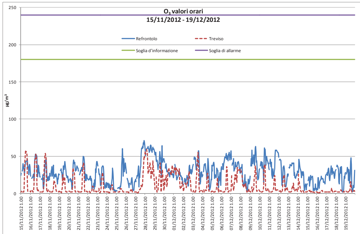
Grafico 6: Valori orari di O 3 rilevati presso la stazione fissa di Treviso e la stazione rilocabile posizionata a Refrontolo – campagna invernale.
