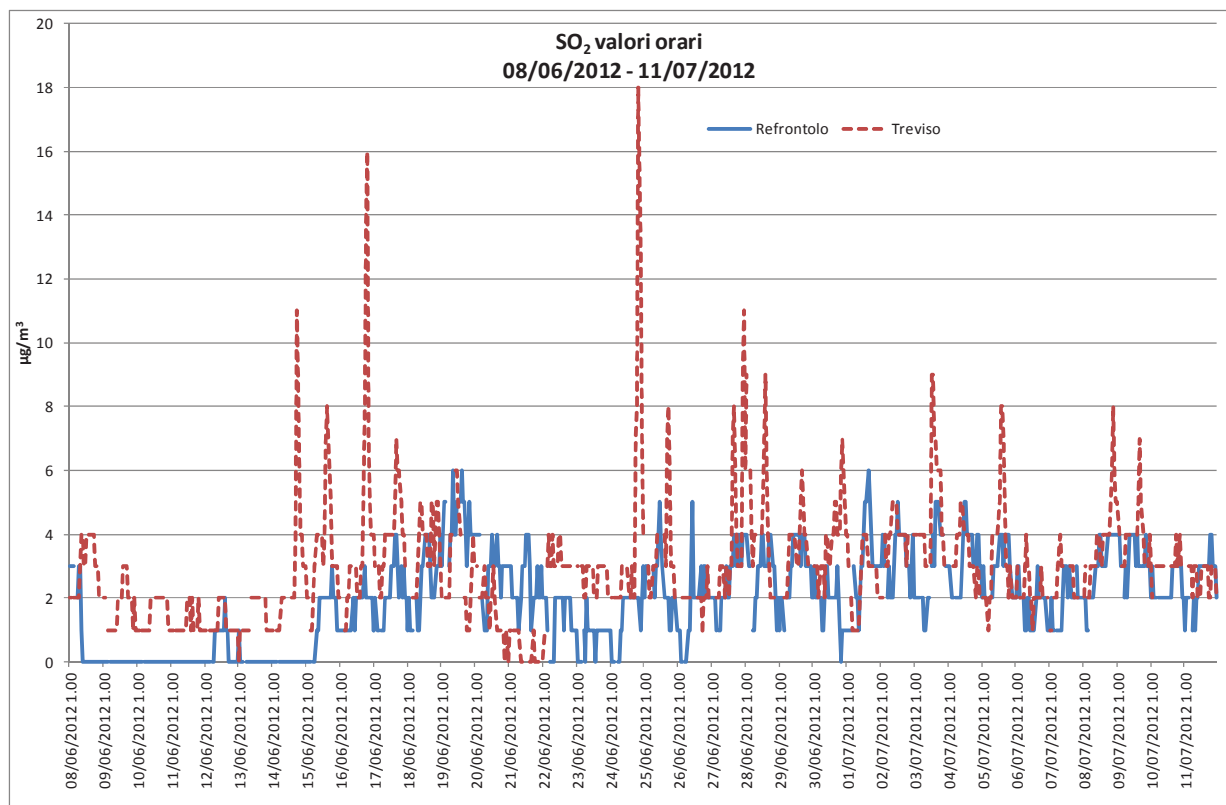
Grafico 9: Valori orari di SO 2 rilevati presso la stazione fissa di Treviso e la stazione rilocabile posizionata a Refrontolo – campagna estiva.
