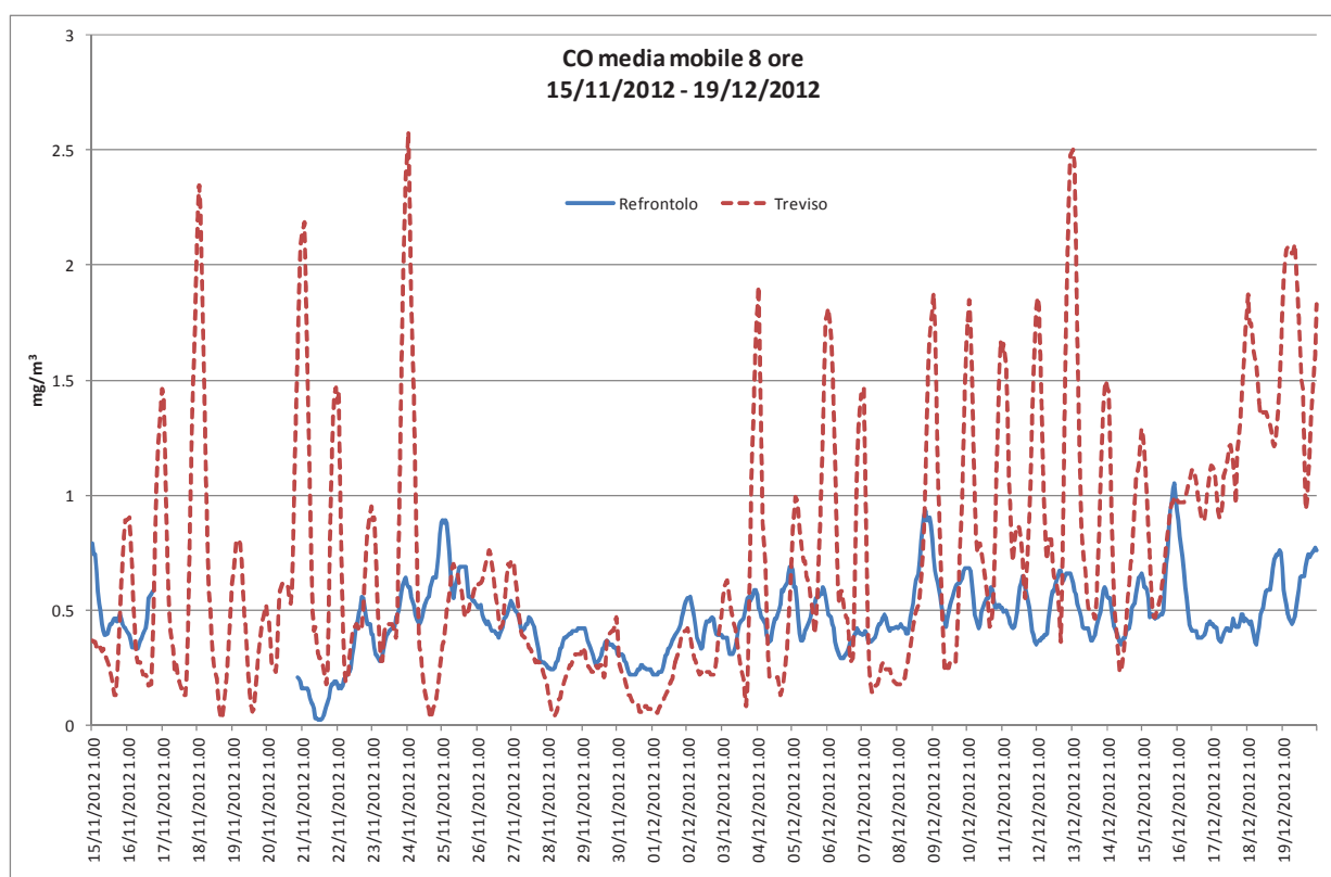
Grafico 2: Media orario di 8 ore di CO rilevati presso la stazione fissa di Treviso e la stazione rilocabile posizionata a Refrontolo – campagna invernale.
