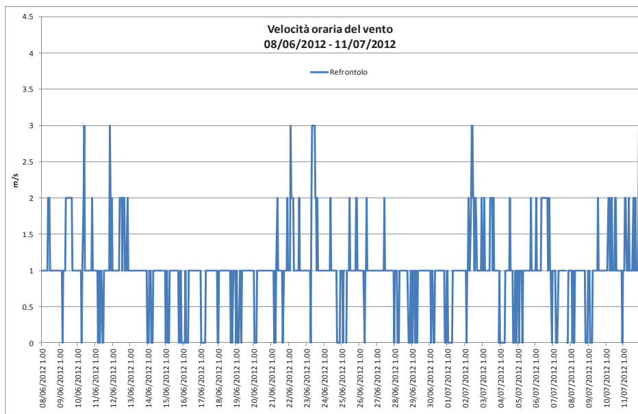
Grafico 16 Valori orari di velocità del vento osservati presso la stazione rilocabile – campagna estiva.
