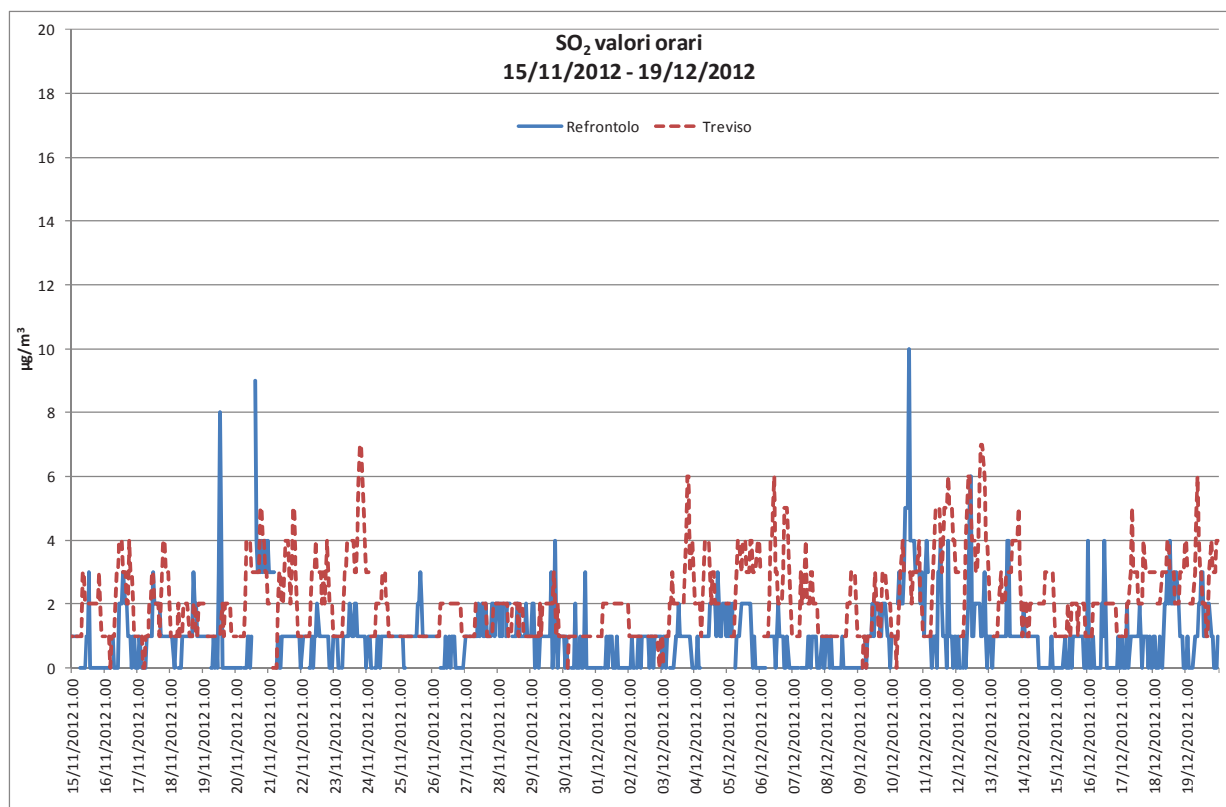
Grafico 10: Valori orari di SO 2 rilevati presso la stazione fissa di Treviso e la stazione rilocabile posizionata a Refrontolo – campagna invernale.
