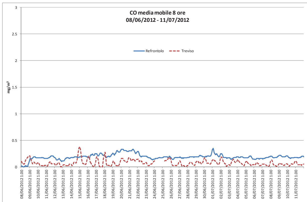
Grafico 1: Media mobile di 8 ore di CO rilevati presso la stazione fissa di Treviso e la stazione rilocabile posizionata a Refrontolo – campagna estiva.
