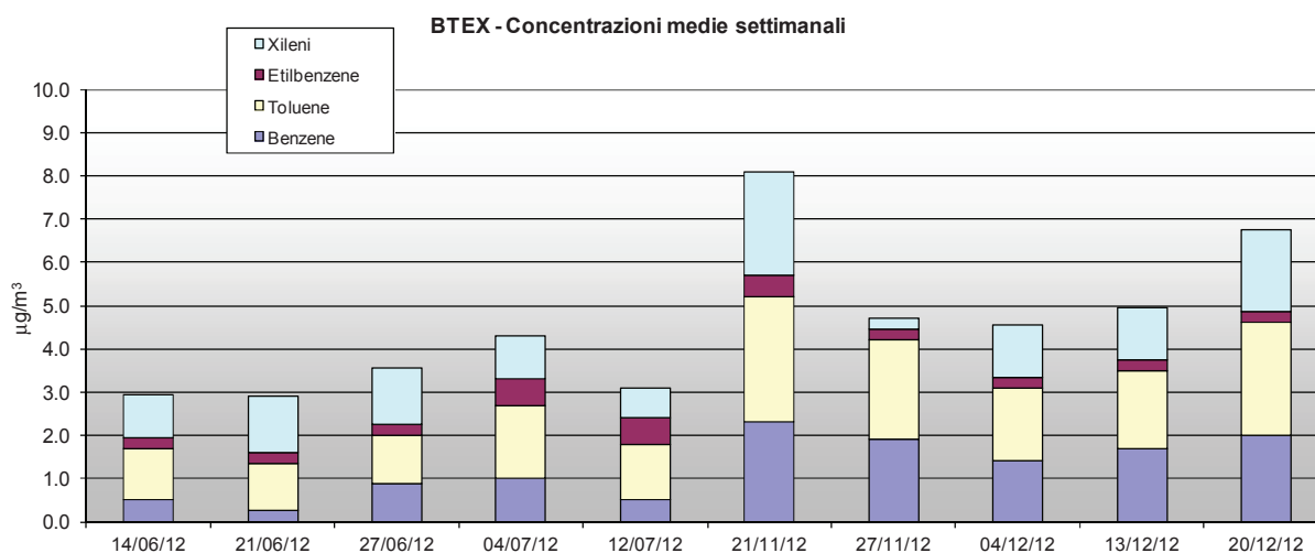
Grafico 15 Valori settimanali di BTEX (Benzene, Toluene, Etilbenzene, Xilene) rilevati a Refrontolo.
