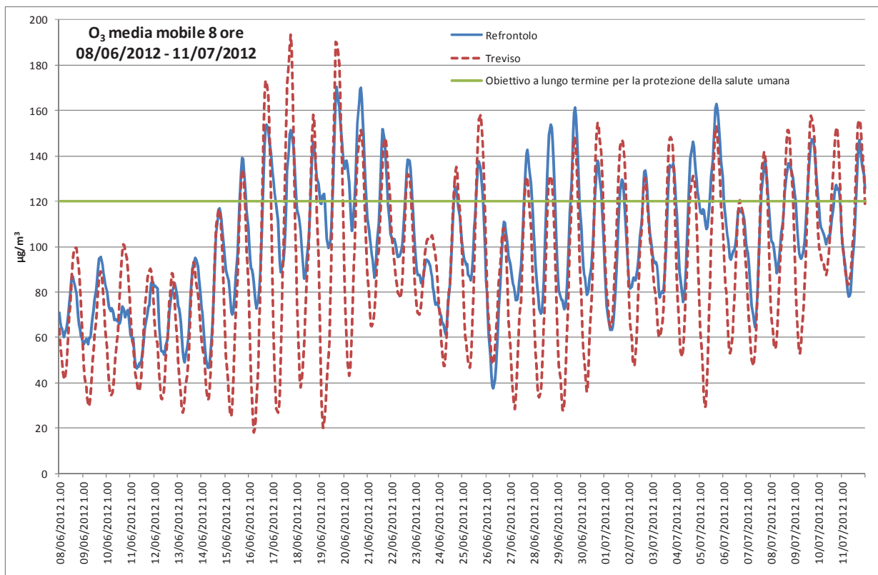
Grafico 7: Media mobile su otto ore di O 3 rilevati presso la stazione fissa di Treviso e la stazione rilocabile posizionata a Refrontolo – campagna estiva.
