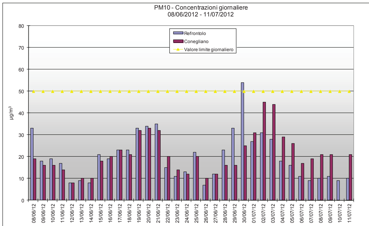
Grafico 13 Valori medi giornalieri di PM10 rilevati presso la stazione fissa di Conegliano e la stazione rilocabile posizionata a Refrontolo – campagna estiva.
