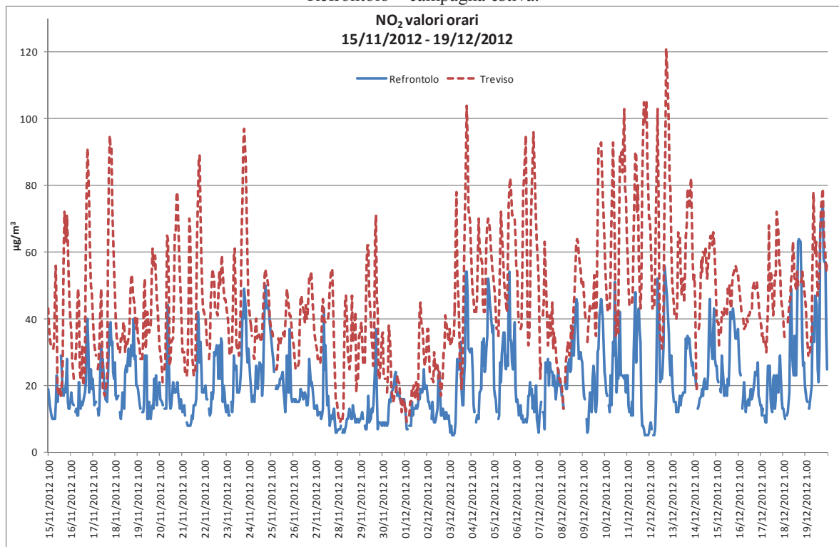
Grafico 4: Valori orari di NO 2 rilevati presso la stazione fissa di Treviso e la stazione rilocabile posizionata a Refrontolo – campagna invernale.
