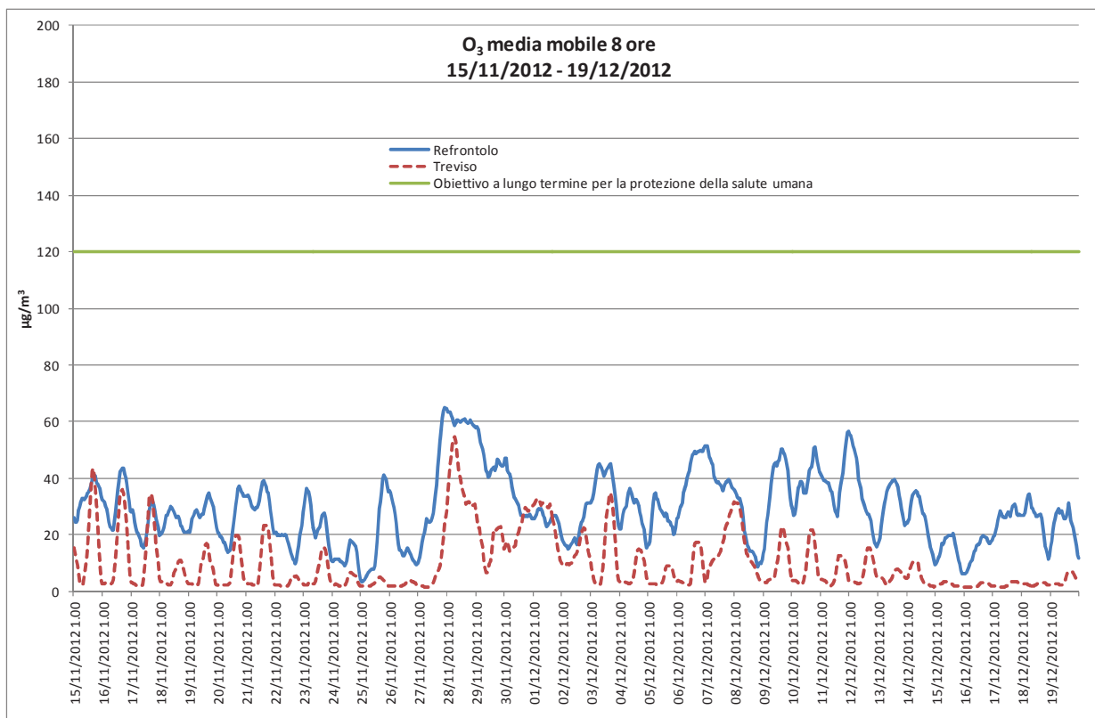
Grafico 8: Media mobile su otto ore di O 3 rilevati presso la stazione fissa di Treviso e la stazione rilocabile posizionata a Refrontolo – campagna invernale.
