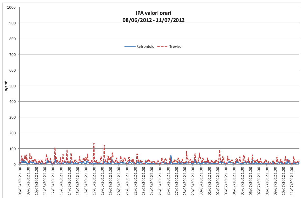
Grafico 11 Confronto tra le concentrazioni medie orarie di IPA totali in fase gassosa a Treviso e presso la stazione rilocabile posizionata a Refrontolo – campagna estiva.
