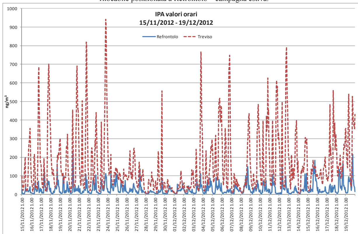
Grafico 12 Confronto tra le concentrazioni medie orarie di IPA totali in fase gassosa a Treviso e presso la stazione rilocabile posizionata a Refrontolo – campagna invernale.
