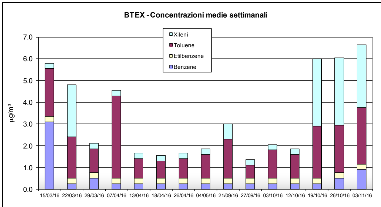
Grafico 2 - Valori settimanali di BTEX (benzene, toluene, etilbenzene e xilene) rilevati a San Vendemiano.
