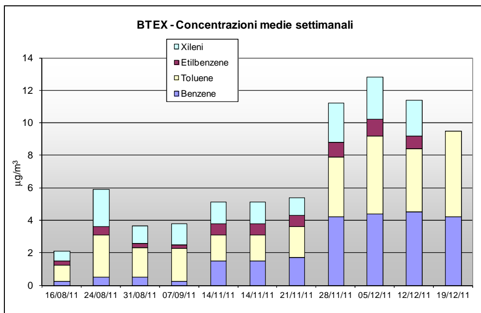
Grafico 3 Valori settimanali di BTEX (Benzene, Toluene, Etilbenzene, Xilene) rilevati a Vidor. Causa problemi strumentali non sono disponibili i dati di Etilbenzene e Xileni per il campione del 19/12/2011.
