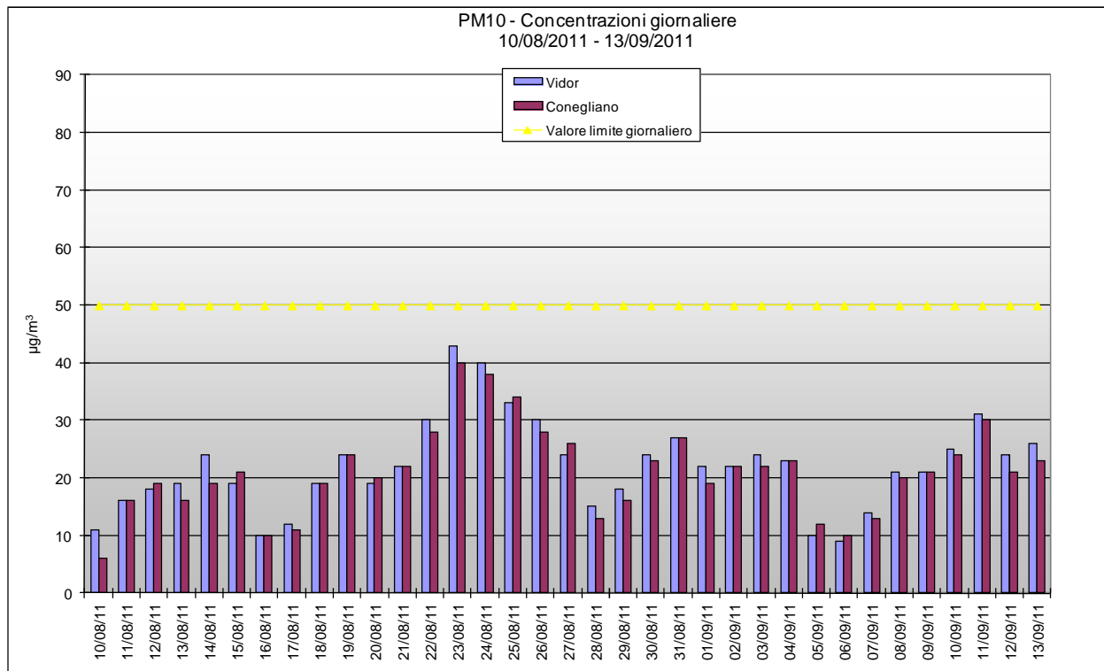
Grafico 1 Valori medi giornalieri di PM10 rilevati presso la stazione fissa di Conegliano ed il campionatore portatile posizionato a Vidor – campagna estiva.
