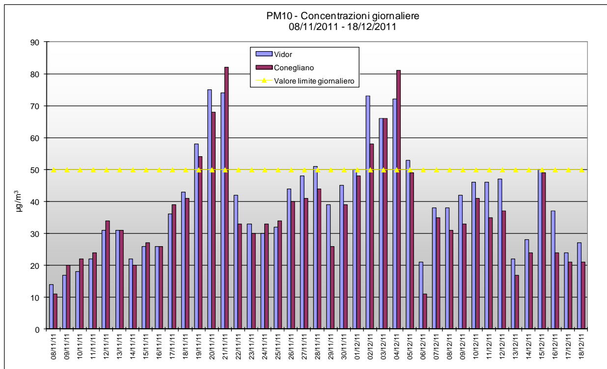
Grafico 2 Valori medi giornalieri di PM10 rilevati presso la stazione fissa di Conegliano ed il campionatore portatile posizionato a Vidor – campagna invernale.
