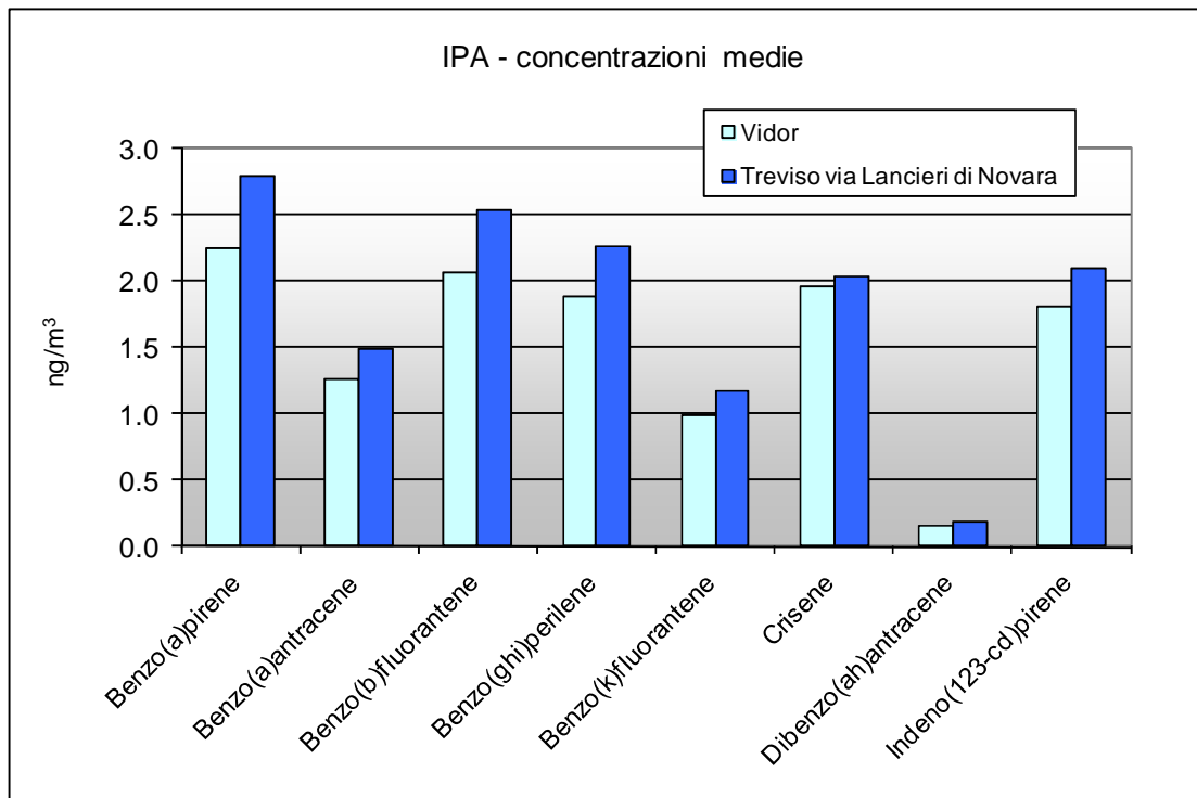
Grafico 4 Confronto tra i valori di IPA determinati su campioni di PM10 prelevati nel sito di monitoraggio e presso la stazione fissa di Treviso durante le campagne.
