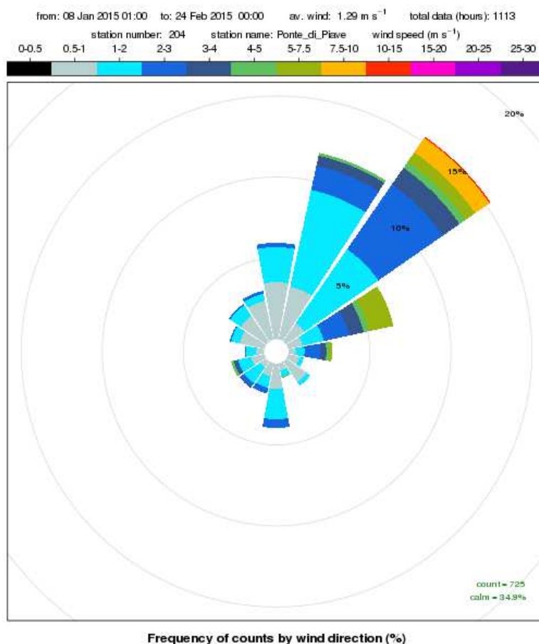
Figura 6. rosa dei venti a scansione oraria registrati presso la stazione meteorologica di Ponte di Piave nel periodo 8 gennaio – 23 febbraio 2015
