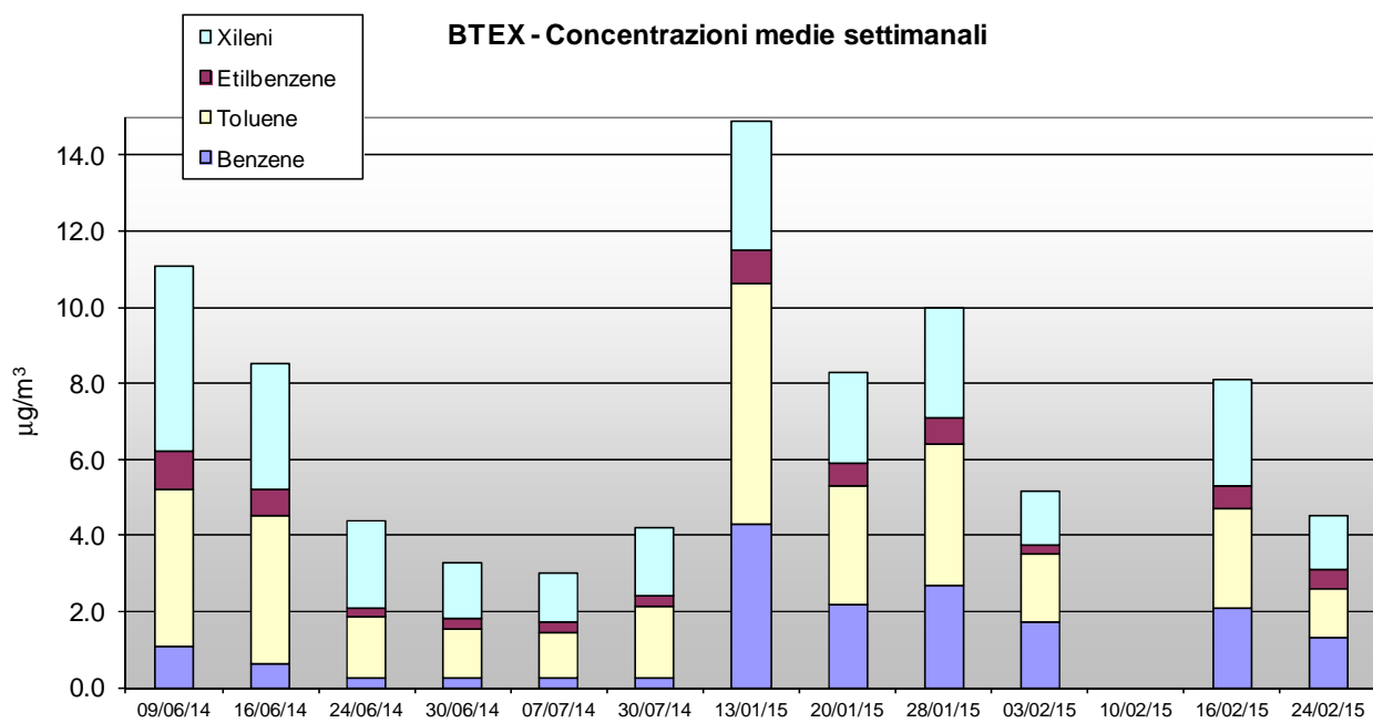
Grafico 2 - Valori settimanali di BTEX (benzene, toluene, etilbenzene e xilene) rilevati a Zenson di Piave.
