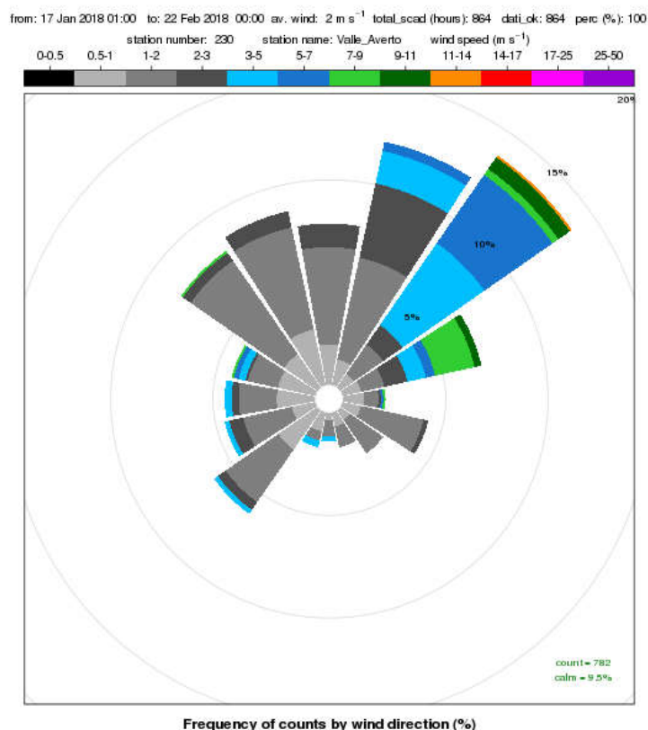
Figura 4. Rosa dei venti registrati presso la stazione meteorologica di Campagna Lupia - Valle Averno nel periodo 17 gennaio - 21 febbraio 2018
