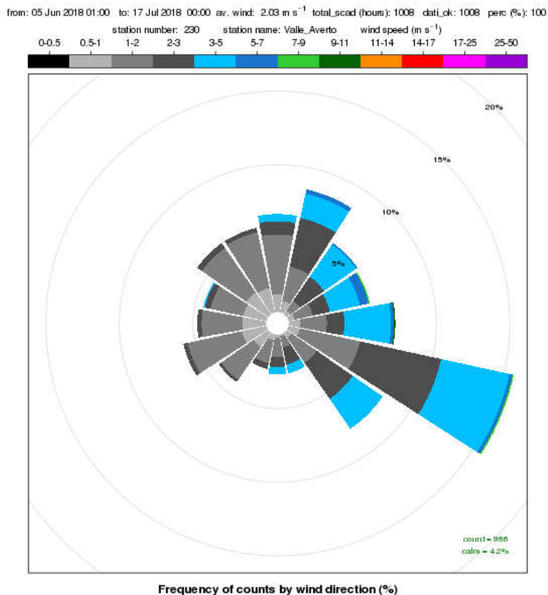
Figura 6. Rosa dei venti registrati presso la stazione meteorologica di Campagna Lupia - Valle Averto nel periodo 5 giugno - 16 luglio 2018
