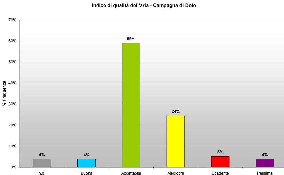
Grafico 1. Calcolo dell'indice sintetico di qualità dell'aria per la campagna di Dolo.
