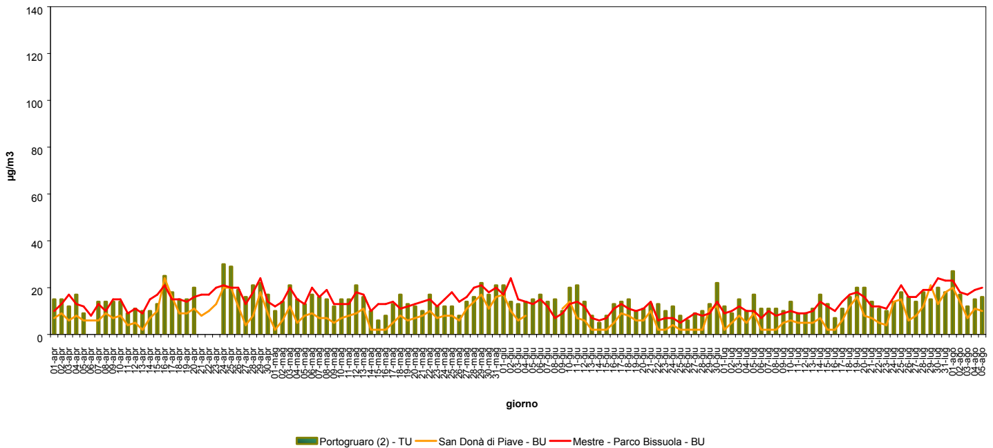
Grafico 4 - Concentrazione giornaliera di PM 2.5 nel Sito 2 (TU) "sem. caldo" (µg/m 3 ).
