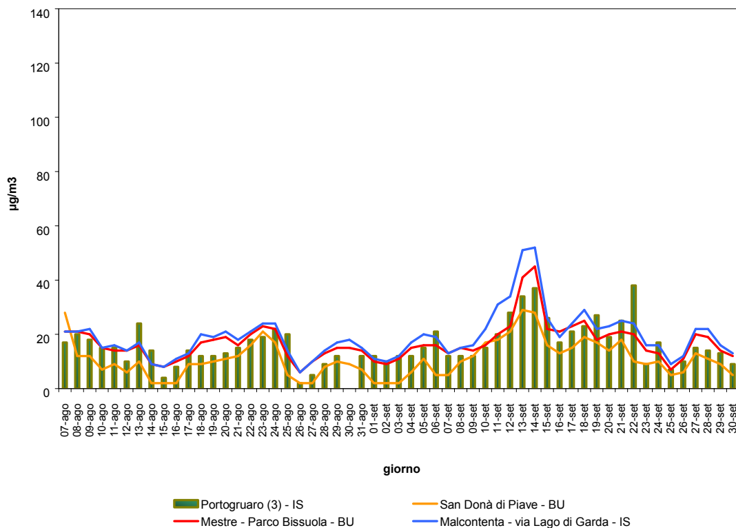
Grafico 5 - Concentrazione giornaliera di PM 2,5 nel Sito 3 (IS) "sem. caldo" (µg/m 3 ).
