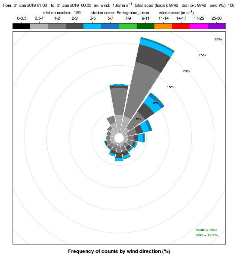
Figura 4. Rosa dei venti registrati presso la stazione meteorologica di Portogruaro nel periodo 1 gennaio – 31 dicembre 2018
