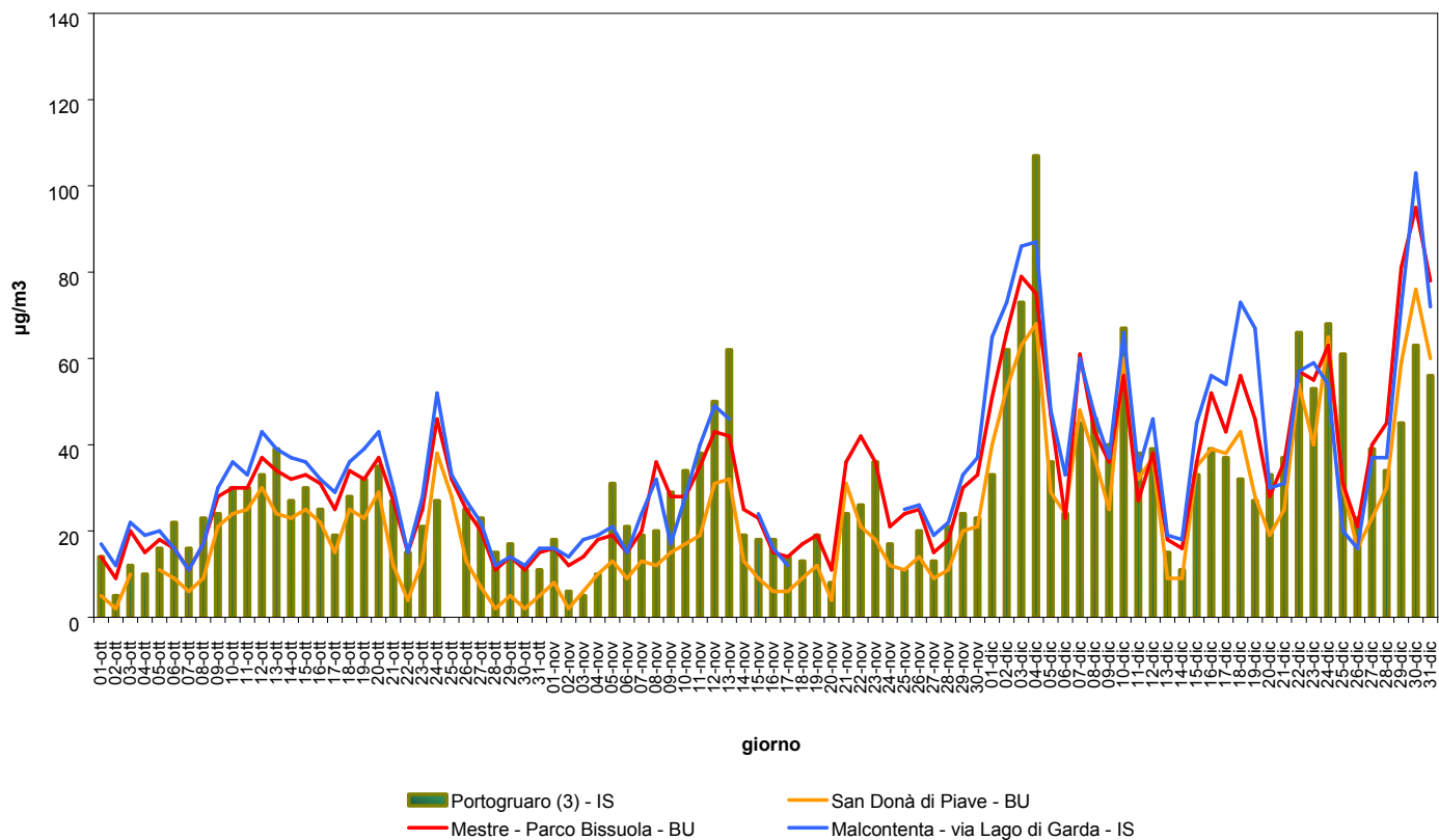
Grafico 6 - Concentrazione giornaliera di PM 2,5 nel Sito 3 (IS) "sem. freddo" (µg/m 3 ).
