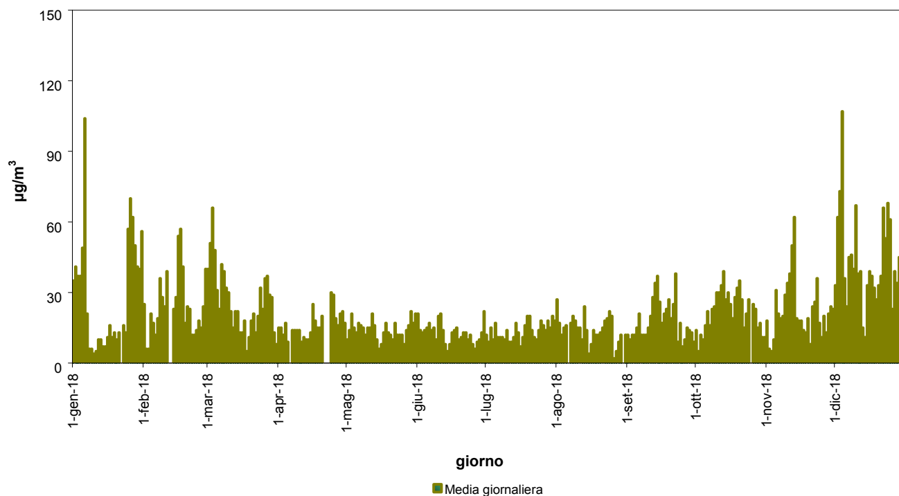
Grafico 1 - Concentrazione giornaliera di PM_{2,5} ( \mu g/m^3 ) rilevata nel 2018 nel Comune di Portogruaro.
