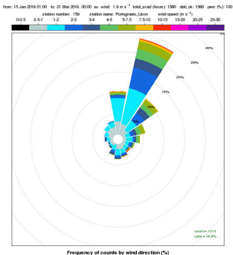
Figura 4. Rosa dei venti registrati presso la stazione meteorologica di Portogruaro Lison nel periodo 15 gennaio - 20 marzo 2016
