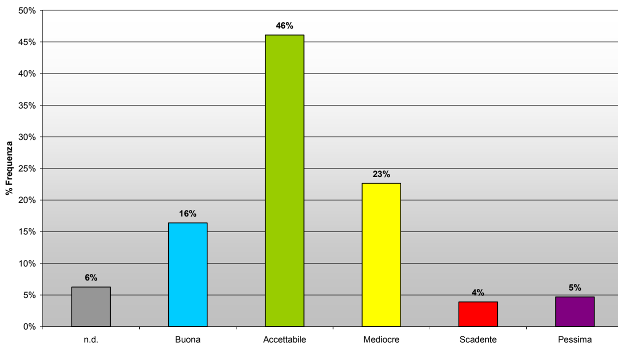
Indice di qualità dell'aria - Campagna di Pramaggiore 2016
