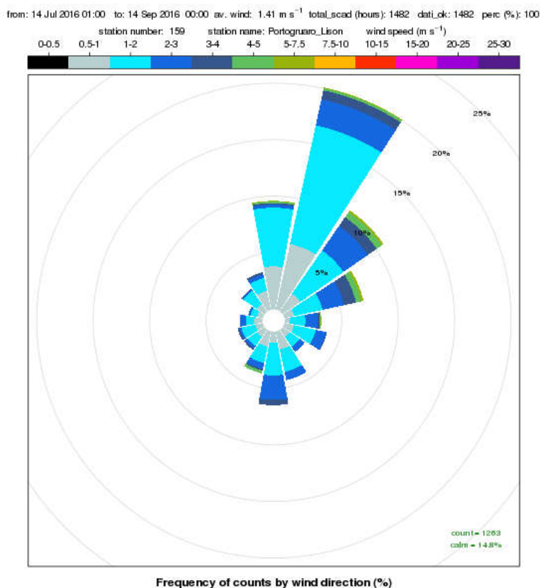
Figura 6. Rosa dei venti registrati presso la stazione meteorologica di Portogruaro Lison nel periodo 14 luglio- 13 settembre 2016
