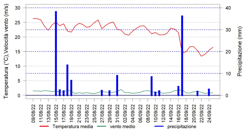
Andamento giornaliero dei parametri meteorologici a Campodarsego Periodo: 09/08/2022 - 25/09/2022
