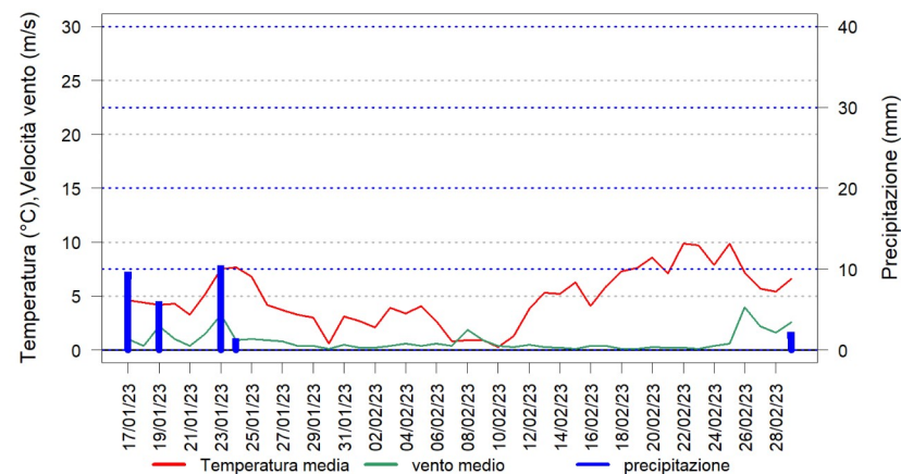
Andamento giornaliero dei parametri meteorologici a Campodarsego Periodo: 17/01/2023 - 01/03/2023
