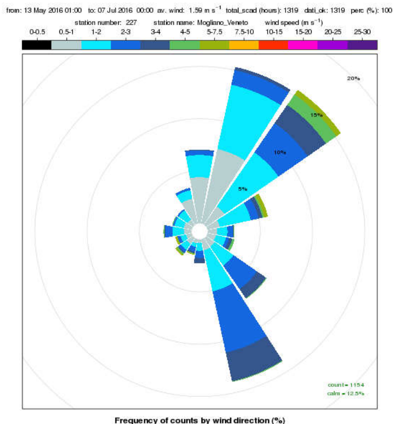
Figura 4. Rosa dei venti a scansione oraria registrati presso la stazione meteorologica di Mogliano Veneto nel periodo 13 maggio - 6 luglio 2016.
