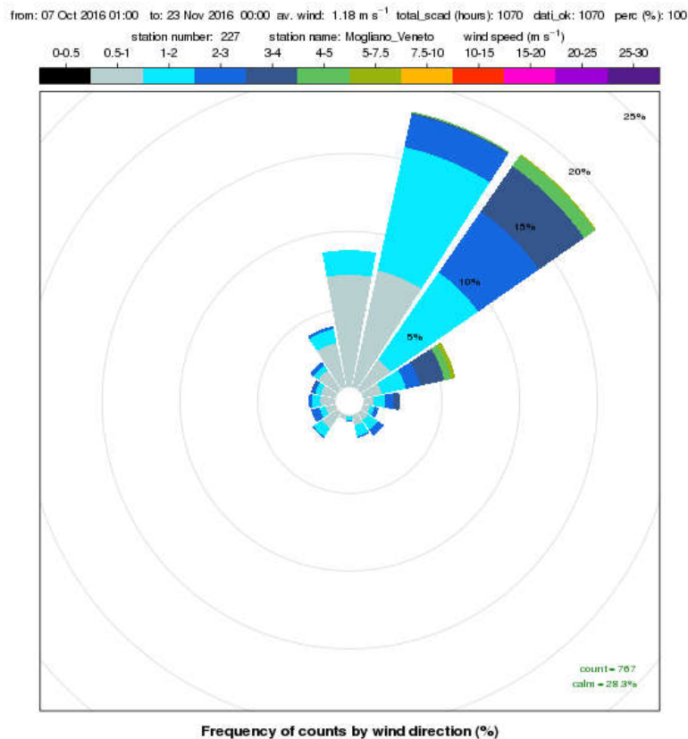
Figura 6. Rosa dei venti a scansione oraria registrati presso la stazione meteorologica di Mogliano Veneto nel periodo 7 ottobre - 23 novembre 2016.
