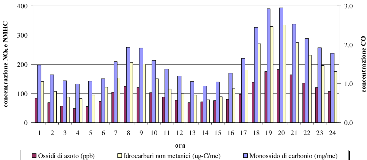
Grafico 7 – Giorno tipo CO – NO x – NMHC.
