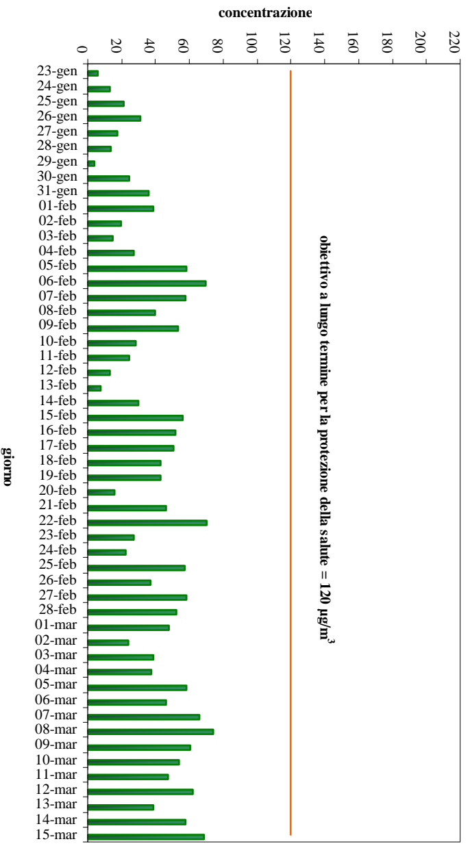
Grafico 7 – Concentrazione Massima Giornaliera della Media Mobile di 8 ore di O 3 (µg/m 3 ).
