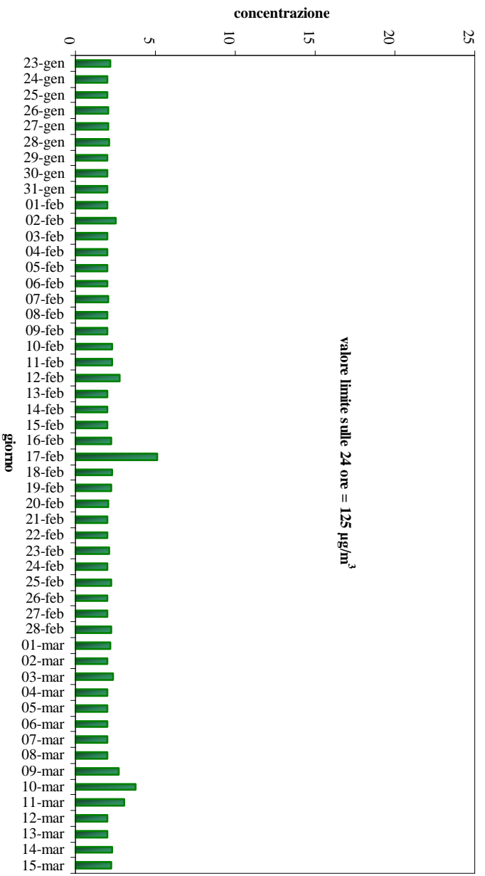
Gráfico 5 – Concentrazione Media Giornaliera di SO 2 (µg/m 3 ).
