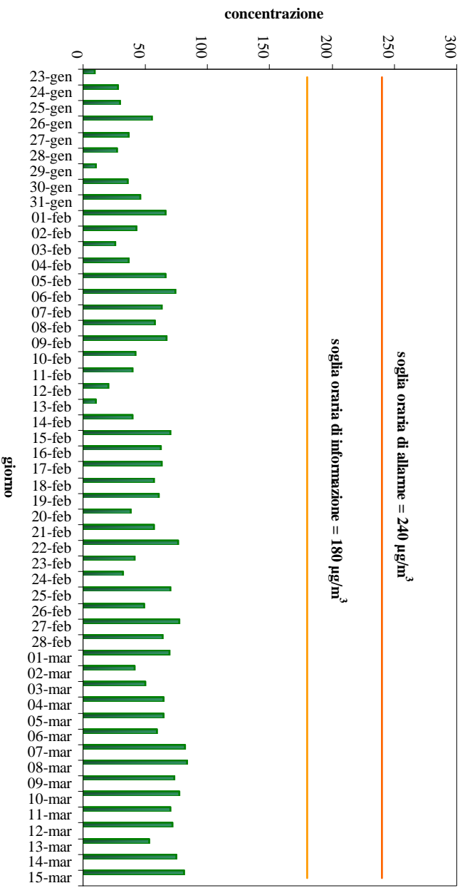
Grafico 6 – Concentrazione Massima Giornaliera della Media Oraria di O 3 (µg/m 3 ).
