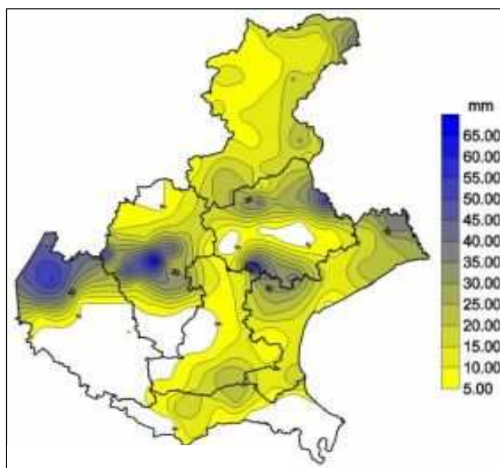
Fig. 3 Precipitazioni del 4 agosto 2002
