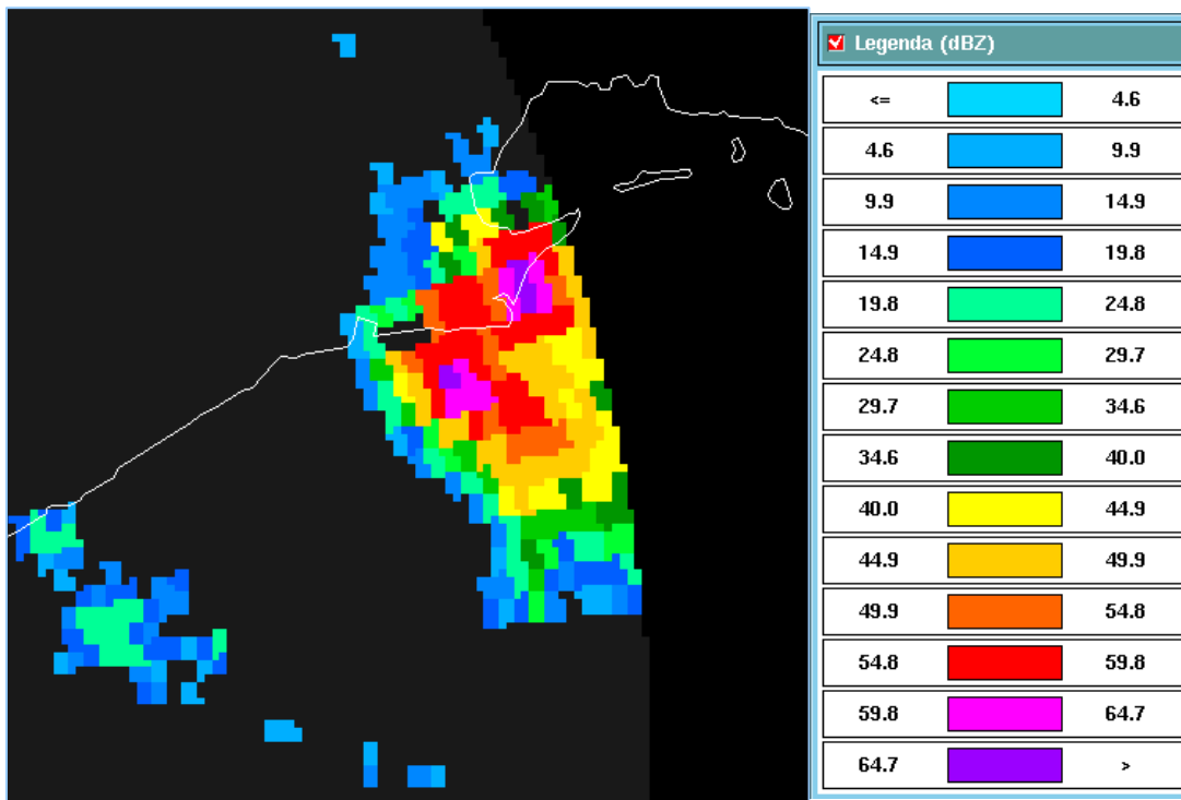
Fig. 4 Immagine radar (Ibmz) e legenda riflettività (palette) delle ore 00.32 UTC del 20 luglio 1997 (Bibione)
