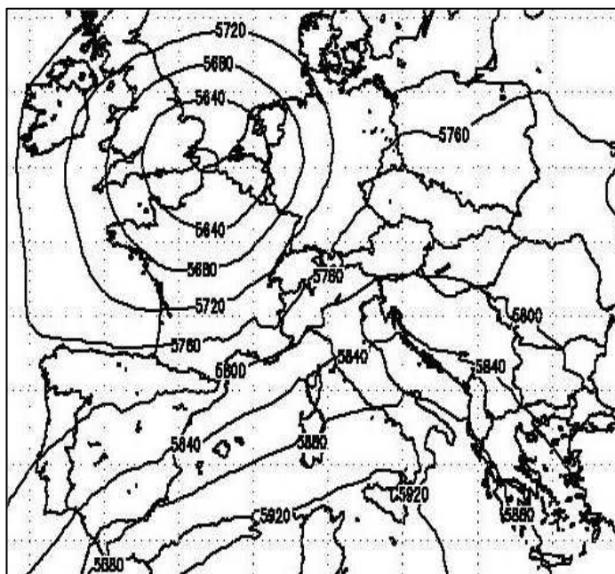
Fig.1 Situazione sinottica relativa al 4 agosto 2002: carta delle altezze geopotenziali a 500 hpa.
