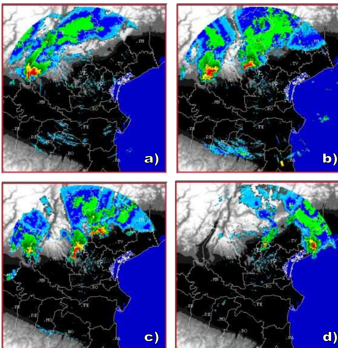
Fig. 2 Immagini radar: fasi delle celle temporalesche/grandinigene
