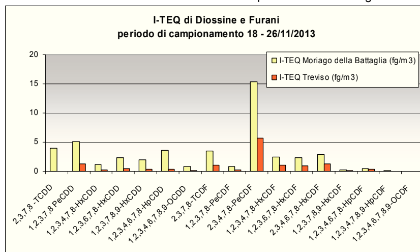
Figura 15 – Concentrazioni medie di diossine e furani espresse come I-TEQ rilevati presso i siti di Moriago della Battaglia e Treviso
