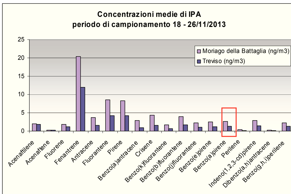
Figura 19 – Concentrazioni medie di IPA rilevati presso i siti di Moriago della Battaglia e Treviso
