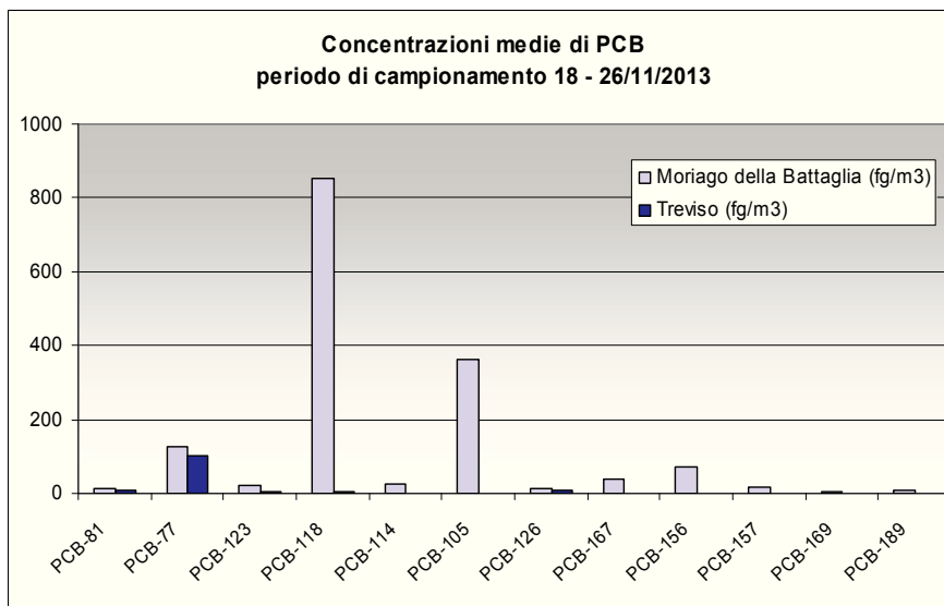
Figura 16 – Concentrazioni medie di PCB-DL rilevati presso i siti di Moriago della Battaglia e Treviso
