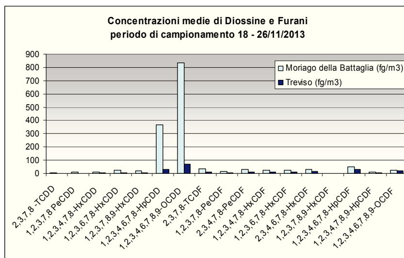
Figura 14 – Concentrazioni medie di diossine e furani rilevati presso i siti di Moriago della Battaglia e Treviso
