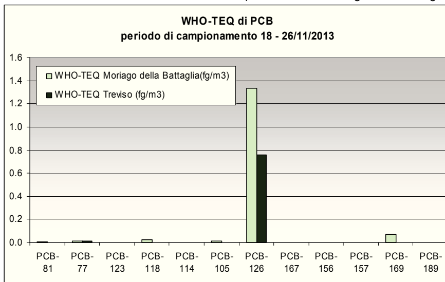
Figura 17 – Concentrazioni medie di PCB espresse come WHO -TEQ rilevati presso i siti di Moriago della Battaglia e Treviso
