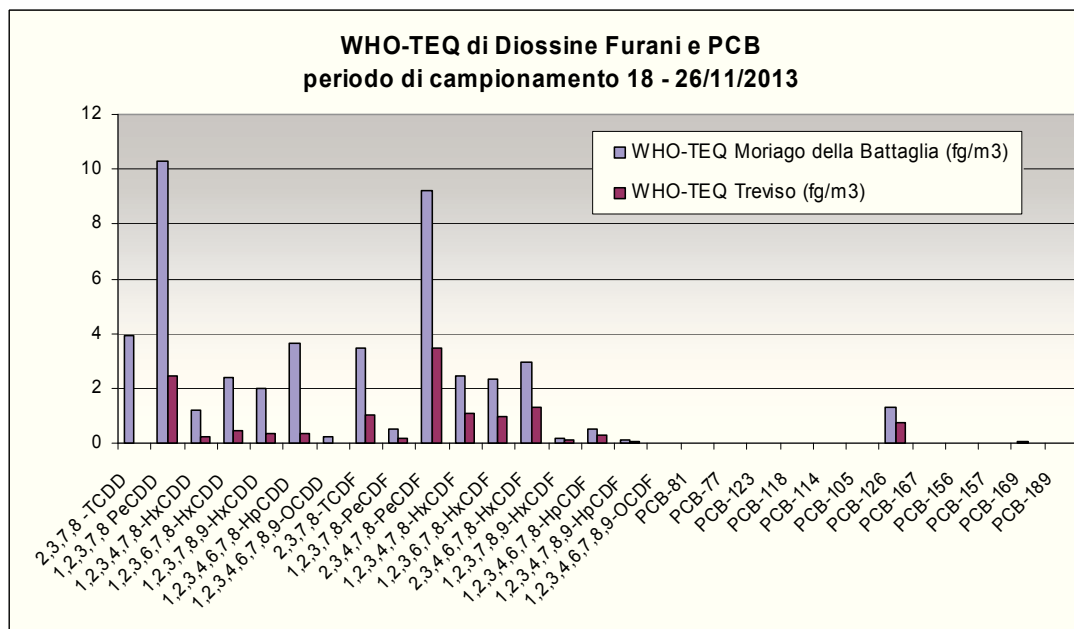
Figura 18 – Concentrazioni medie di Diossine, Furani e PCB espresse come WHO -TEQ rilevati presso i siti di Moriago della Battaglia e Treviso
