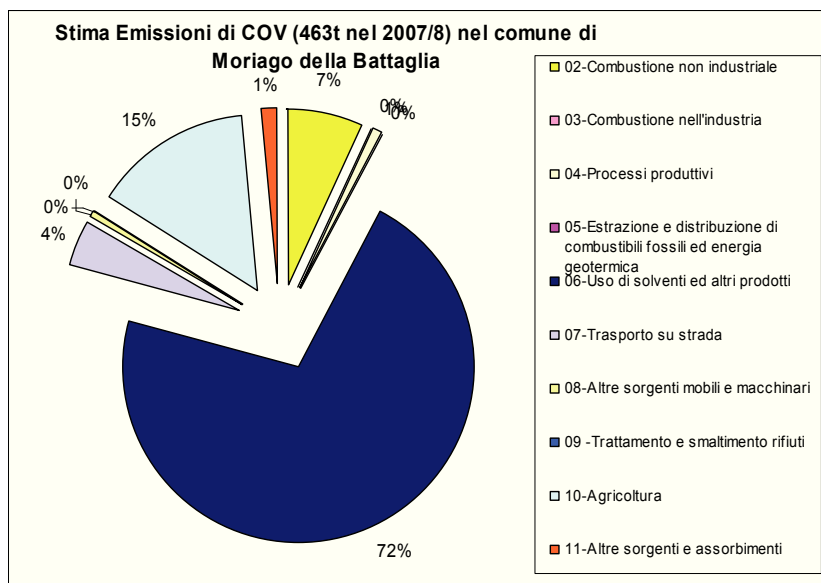
Figura 13 Contributi percentuali dei macrosettori CORINAIR alla stima emissioni di COV nel comune di Moriago della Battaglia – dati INEMAR 2007/8
