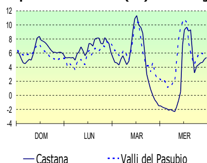
Temperatura aria 2m (°C) ultimi 4 g.
