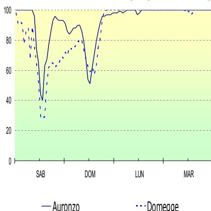
Umidità rel. aria 2m (%) ultimi 4 g.
