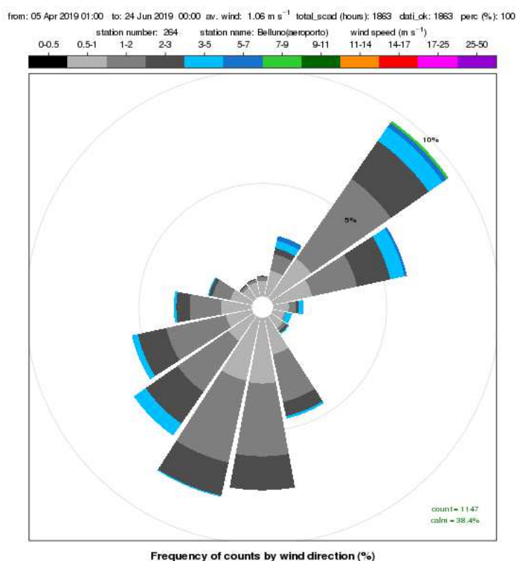
Figura 2: rosa dei venti registrati presso la stazione meteorologica di Belluno - Aeroporto nel periodo 5 aprile – 23 giugno 2019
