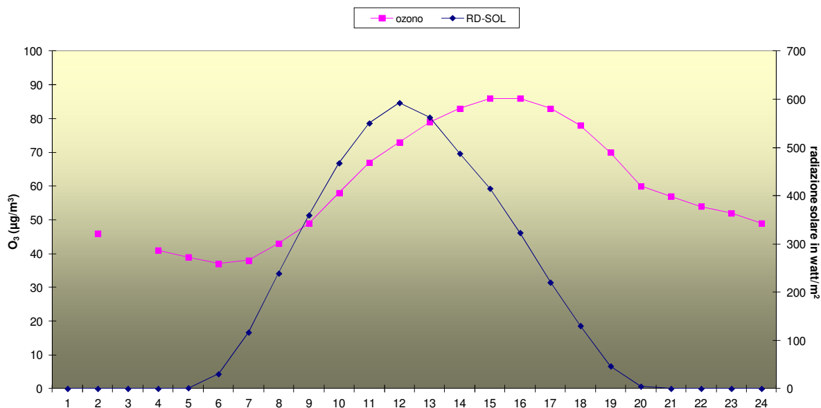
COMUNE DI BELLUNO LOC. CIRVOI: PARAMETRI OZONO (O 3 ) E RADIAZIONE SOLARE GIORNO DAL 5 APRILE AL 23 GIUGNO 2019
