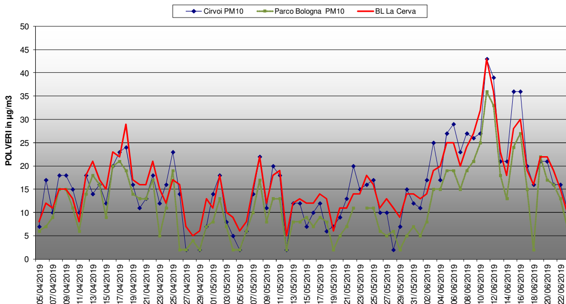
STAZIONI DI Belluno Cirvoi (Mezzo Mobile), Belluno Parco Bologna e Belluno La Cerva: CONFRONTO POLVERI PM10 DAL 5 APRILE AL 23 GIUGNO 2019
