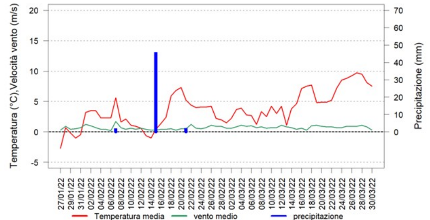
Andamento giornaliero dei parametri meteorologici a Santa Giustina Bellunese Periodo: 27/01/2022 - 30/03/2022
