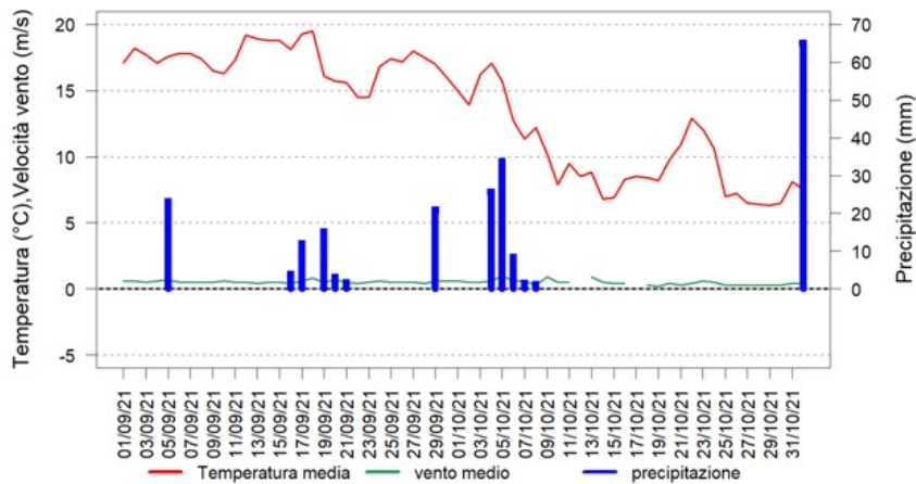
Andamento giornaliero dei parametri meteorologici a Santa Giustina Bellunese Periodo: 01/09/2021 - 01/11/2021
