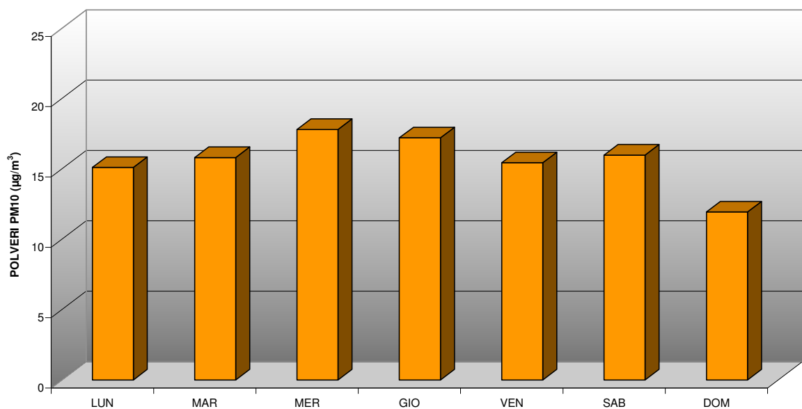
COMUNE DI OSPITALE DI CADORE: PARAMETRO POLVERI PM10 SETTIMANA TIPO DAL 2 OTTOBRE 2014 AL 10 FEBBRAIO 2015
