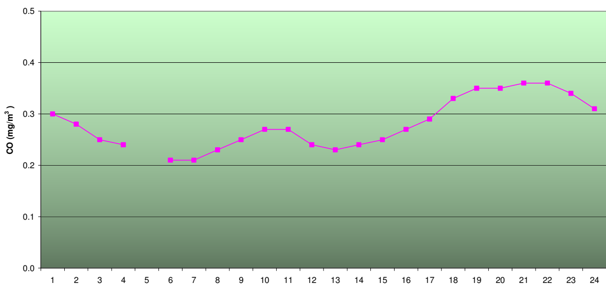
COMUNE DI OSPITALE DI CADORE: PARAMETRO MONOSSIDO DI CARBONIO (CO) GIORNO TIPO DAL 2 OTTOBRE 2014 AL 10 FEBBRAIO 2015
