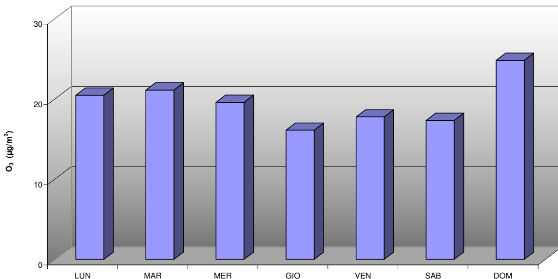
COMUNE DI OSPITALE DI CADORE: PARAMETRO OZONO (O 3 ) SETTIMANA TIPO DAL 2 OTTOBRE 2014 AL 10 FEBBRAIO 2015
