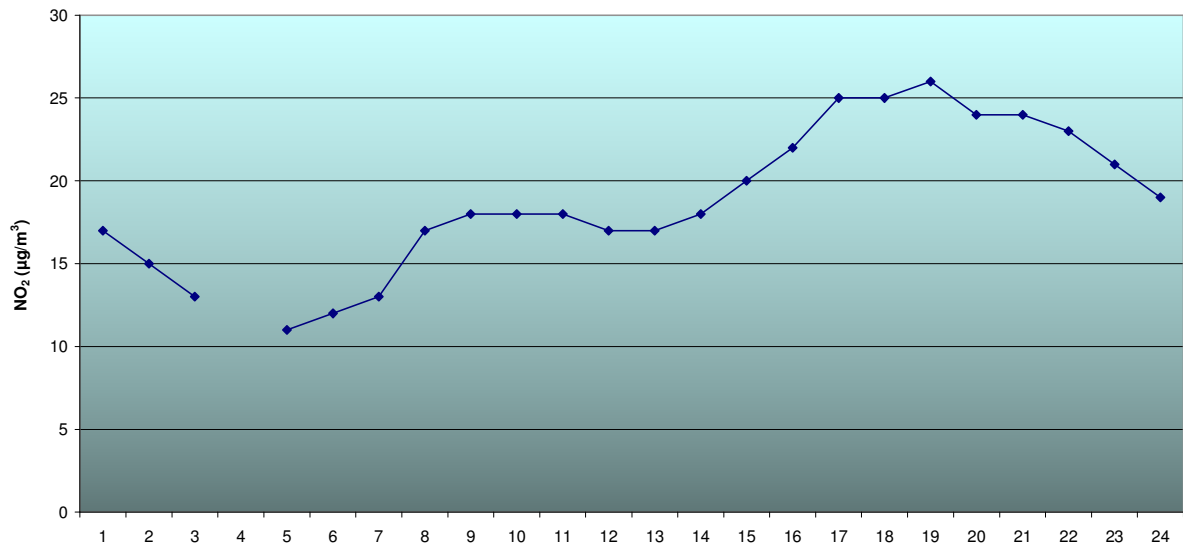
COMUNE DI OSPITALE DI CADORE: PARAMETRO BISSIDO DI AZOTO (NO 2 ) GIORNO TIPO DAL 2 OTTOBRE 2014 AL 10 FEBBRAIO 2015
