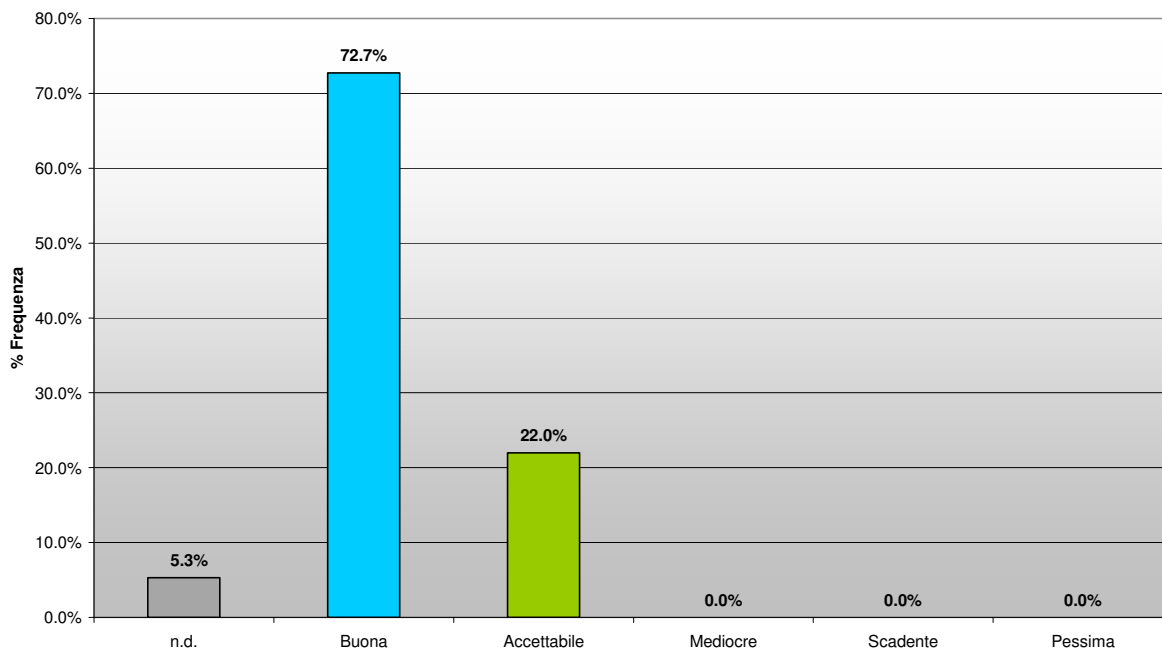
Indice di qualità dell'aria - Campagna di Ospitale di Cadore
