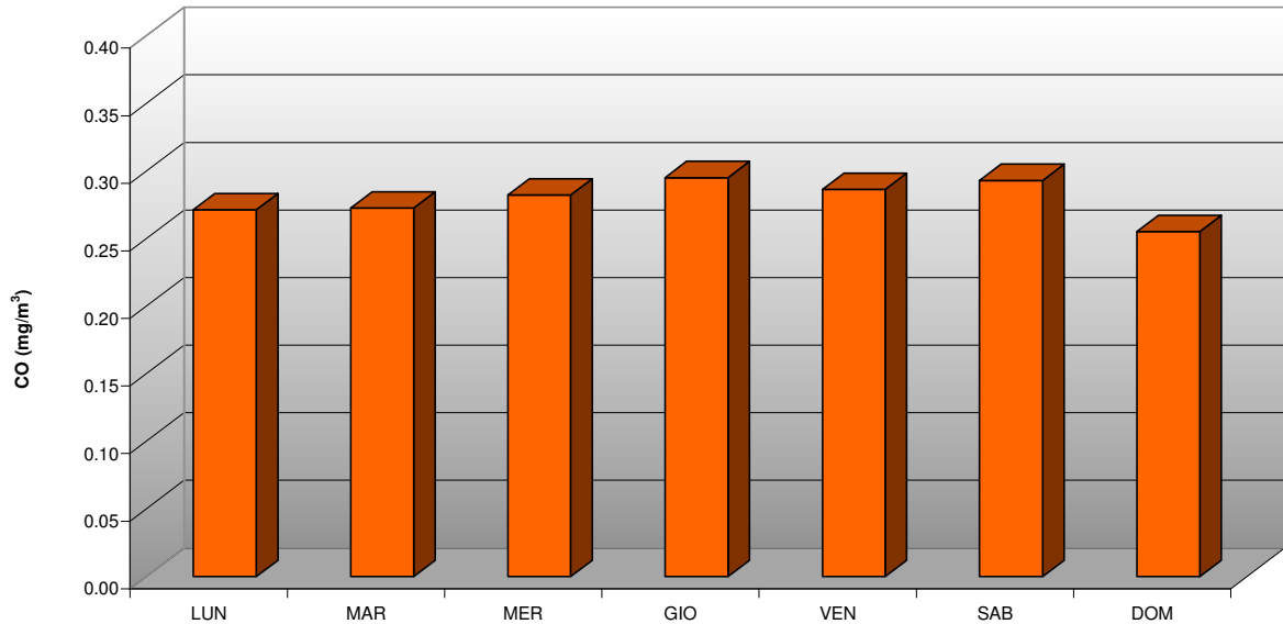
COMUNE DI OSPITALE DI CADORE: PARAMETRO MONOSSIDO DI CARBONIO (CO) SETTIMANA TIPO DAL 2 OTTOBRE 2014 AL 10 FEBBRAIO 2015
