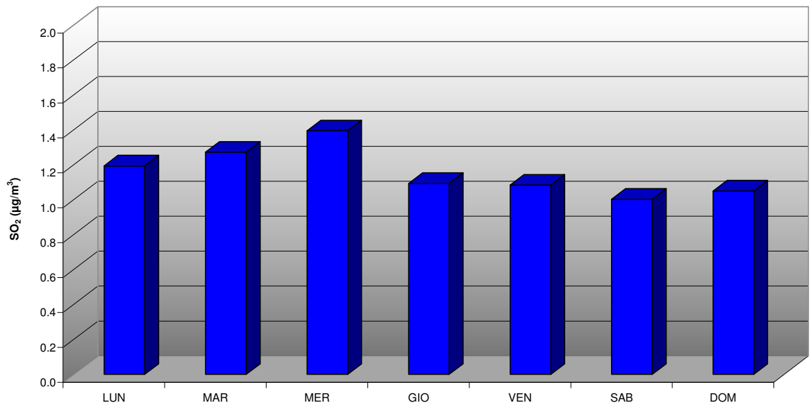
COMUNE DI OSPITALE DI CADORE: PARAMETRO ANIDRIDE SOLFOROSA (SO 2 ) SETTIMANA TIPO DAL 2 OTTOBRE 2014 AL 10 FEBBRAIO 2015
