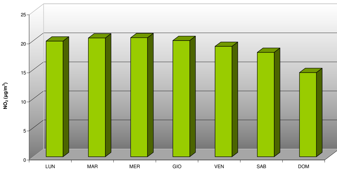
COMUNE DI OSPITALE DI CADORE: PARAMETRO BISSIDO DI AZOTO (NO 2 ) SETTIMANA TIPO DAL 2 OTTOBRE 2014 AL 10 FEBBRAIO 2015
