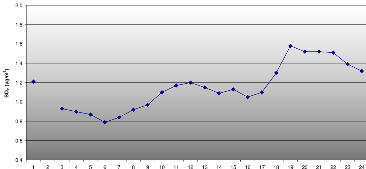
COMUNE DI OSPITALE DI CADORE: PARAMETRO ANIDRIDE SOLFOROSA (SO 2 ) GIORNO TIPO DAL 2 OTTOBRE 2014 AL 10 FEBBRAIO 2015
