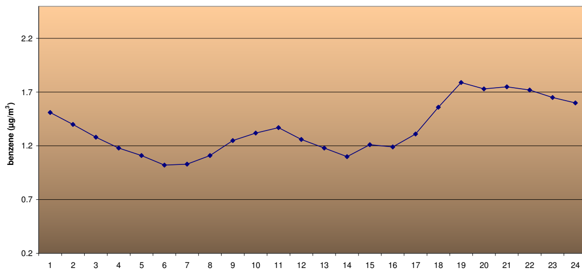
COMUNE DI OSPITALE DI CADORE: PARAMETRO BENZENE (C 6 H 6 ) GIORNO TIPO DAL 2 OTTOBRE 2014 AL 10 FEBBRAIO 2015
