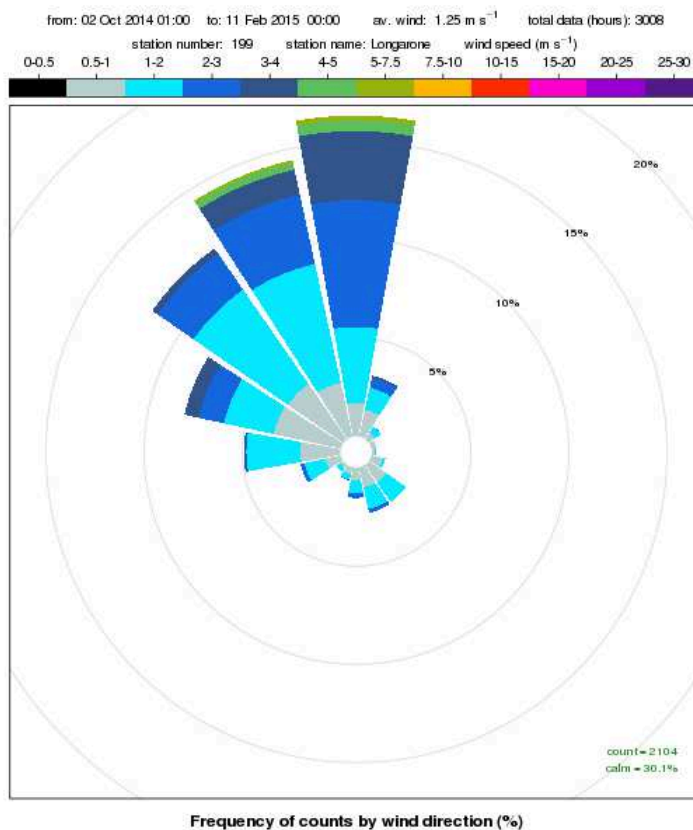
Figura 4: rosa dei venti registrati presso la stazione meteorologica di Longarone nel periodo 2 ottobre 2014 -10 febbraio 2015
