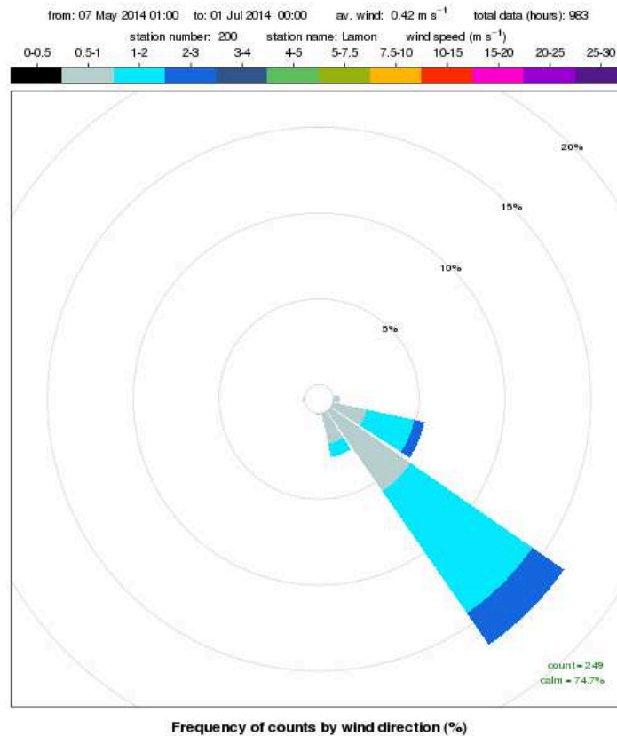
Figura 2: rosa dei venti registrati presso la stazione meteorologica di Lamon nel periodo 7 maggio – 1 luglio 2014
