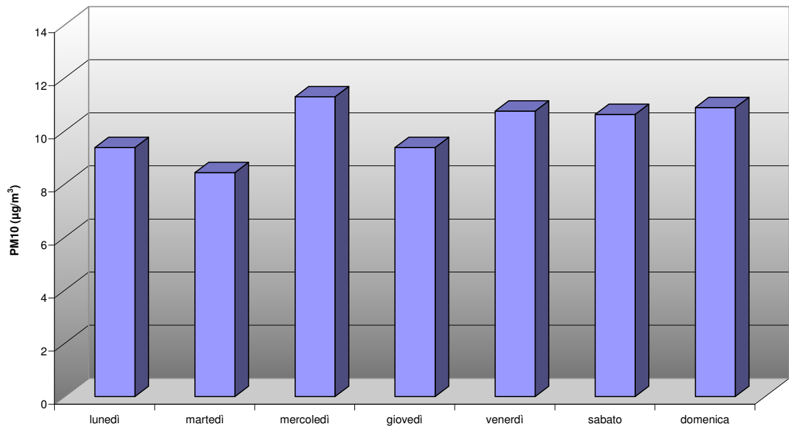
COMUNE DI SORRIVA LOC. SOVRAMONTE: SETTIMANA TIPO POLVERI PM10 DAL 7 MAG AL 1 LUG 2014
