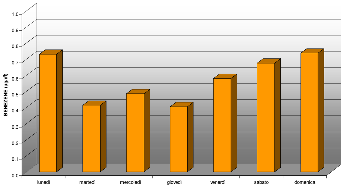
COMUNE DI SOVRAMONTE LOC. SORRIVA: SETTIMANA TIPO BENZENE DAL 7 MAGGIO AL 1 LUGLIO 2014
