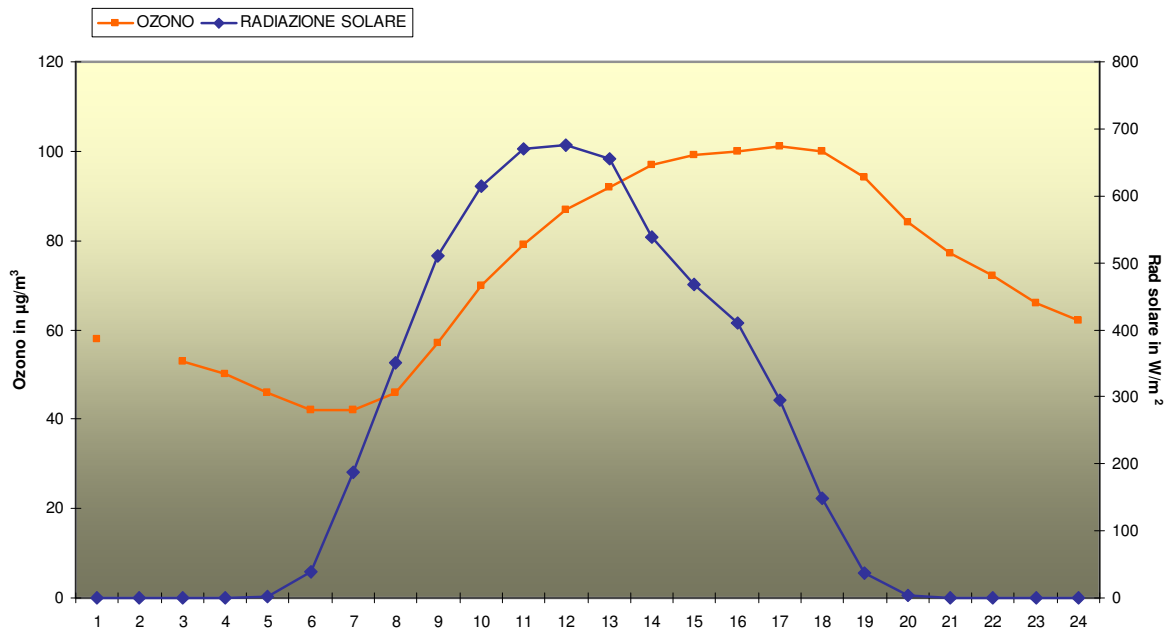
COMUNE DI SOVRAMONTE LOC. SORRIVA: GIORNO TIPO OZONO E RADIAZIONE SOLARE DAL 7 MAGGIO AL 1 LUGLIO 2014
