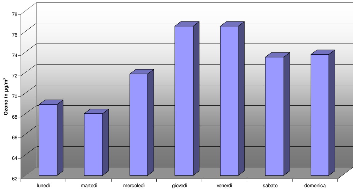
COMUNE DI SOVRAMONTE LOC. SORRIVA: SETTIMANA TIPO OZONO DAL 7 MAG AL 1 LUG 2014
