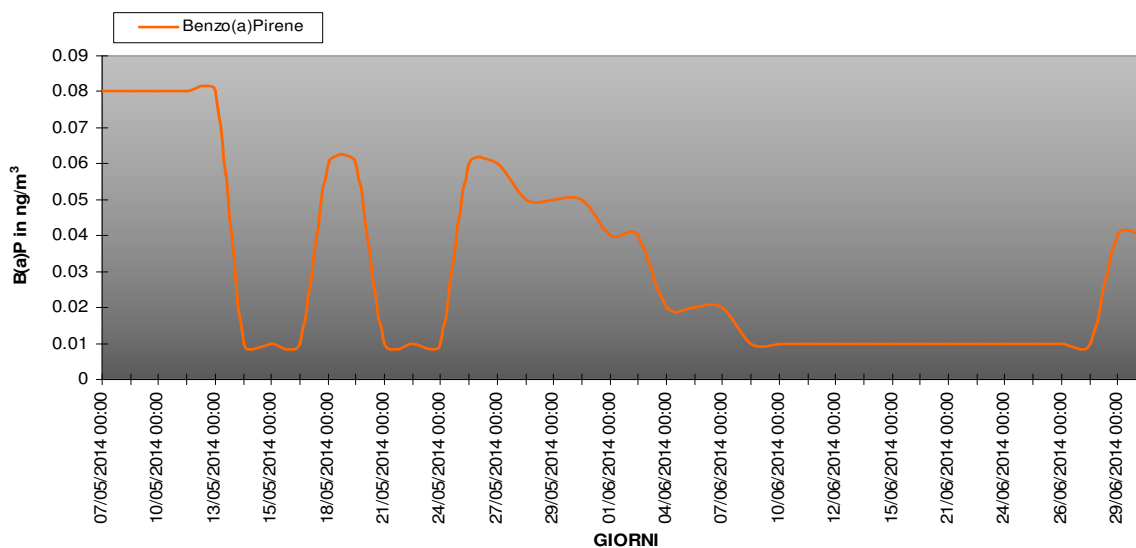
COMUNE DI SOVRAMONTE LOC. SORRIVA : MEDIE GIORNALIERE DI BENZO(a)PIRENE DAL 7 MAG AL 1 LUG 2014
