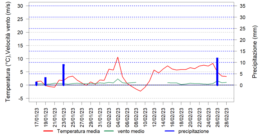
Andamento giornaliero dei parametri meteorologici a Sospirolo Periodo: 17/01/2023 - 28/02/2023
