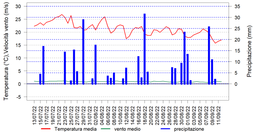
Andamento giornaliero dei parametri meteorologici a Sospirolo Periodo: 13/07/2022 - 12/09/2022
