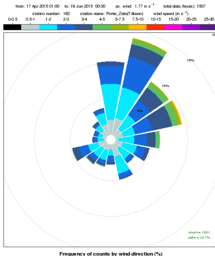
Figura 6: rosa dei venti registrati presso la stazione meteorologica di Tribano nel periodo 17 aprile - 18 giugno 2015
