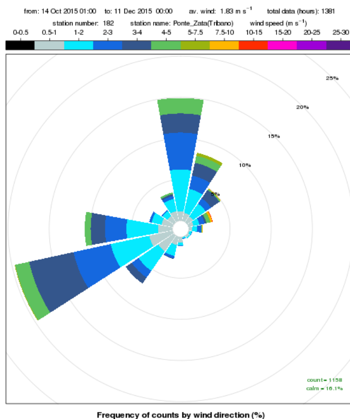
Figura 4: rosa dei venti registrati presso la stazione meteorologica di Tribano nel periodo 14 ottobre - 10 dicembre 2015
