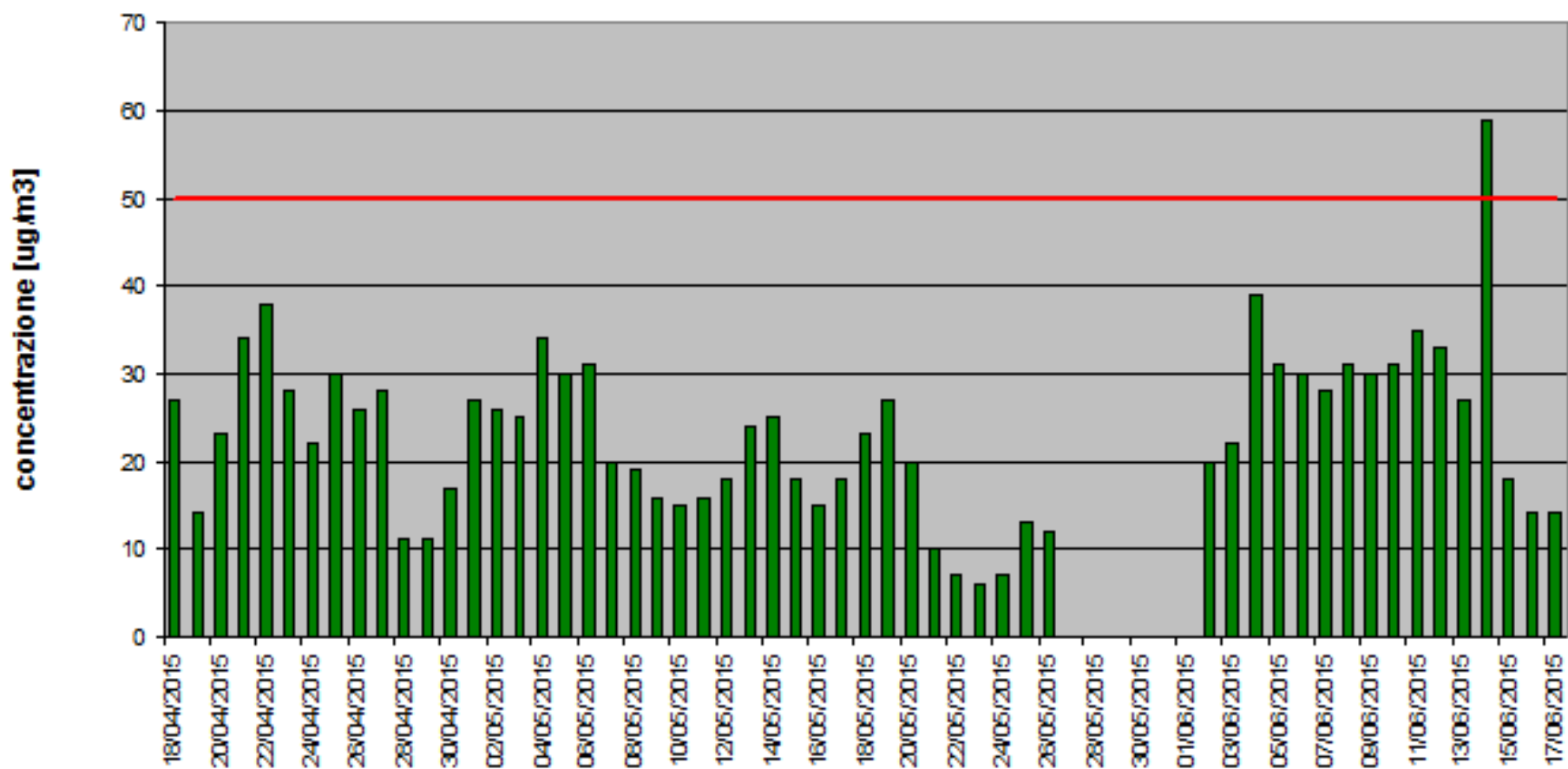
PM10: concentrazione giornaliera [18/04-18/06/2015] vs valore limite
