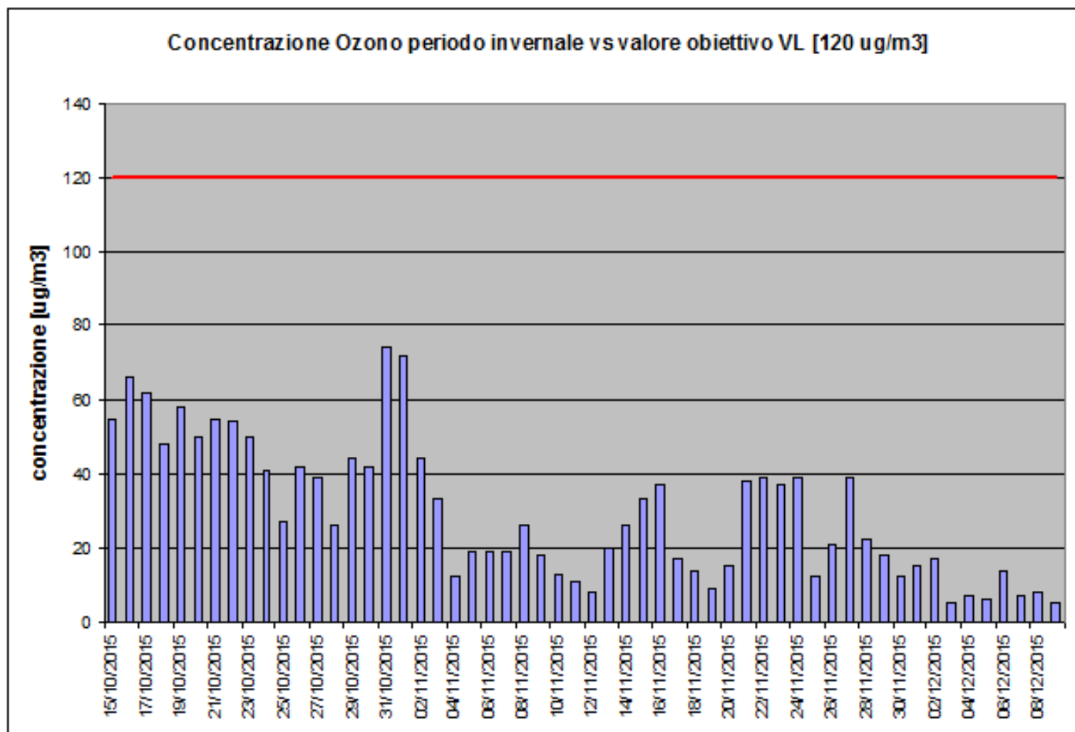
Grafico 1 – Concentrazione Massima Giornaliera della Media Mobile di 8h di O 3 (µg/m 3 ). Semestre “invernale”
