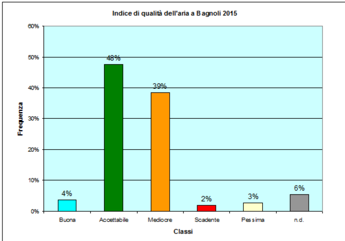
Figura 7. Calcolo dell'indice sintetico di qualità dell'aria per Bagnoli di Sopra
