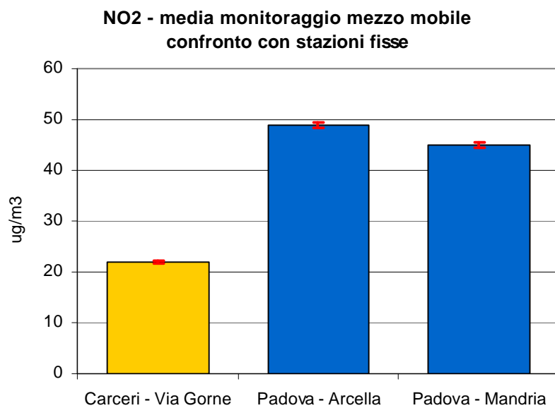
Figura 2.4 Biossido di azoto (NO 2 ): concentrazione media rilevata durante il monitoraggio in Via Gorne nel Comune di Carceri; le barre indicano l'errore standard della media.
