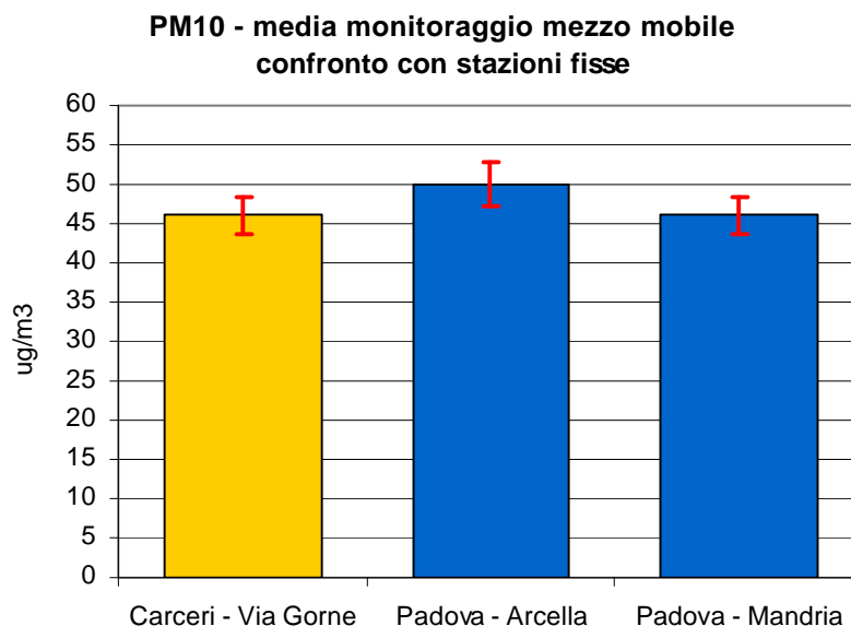
Figura 2.5 Polveri fini (PM 10 ): concentrazione media durante il monitoraggio dal 27/08/09 al 14/10/09 e dal 27/11/09 al 18/01/10 nel Comune di Carceri; le barre indicano l'errore standard della media.
