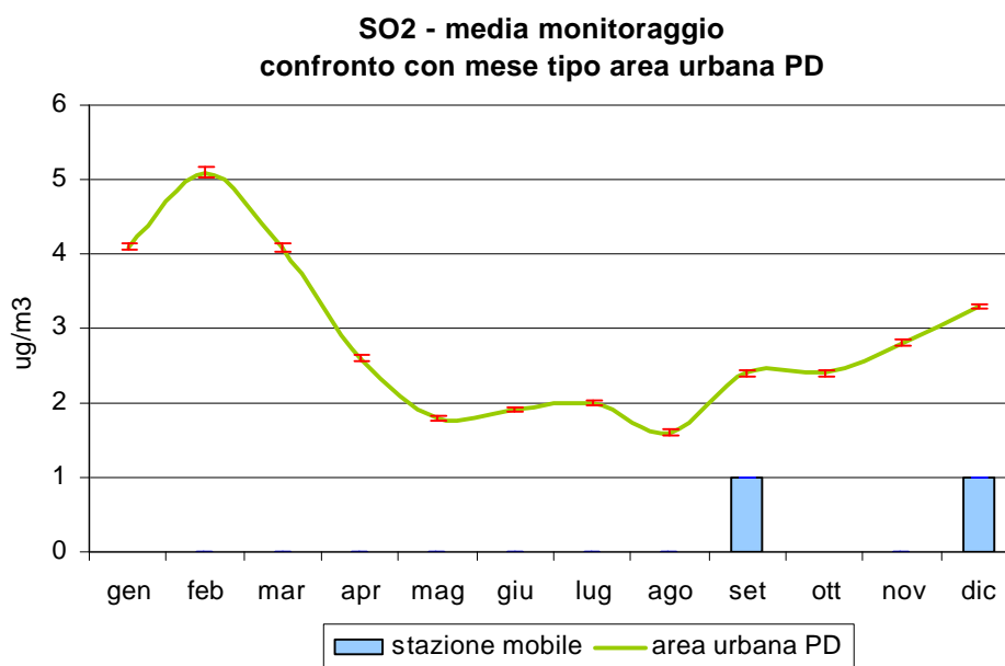
Figura 3.1 Biossido di zolfo (SO 2 ): confronto delle concentrazioni medie rilevate durante il monitoraggio in Via Gorne nel Comune di Carceri, con l’andamento caratteristico del ‘mese tipo’ ricavato dalla serie storica nell’area urbana di Padova; le barre indicano l’errore standard della media.
