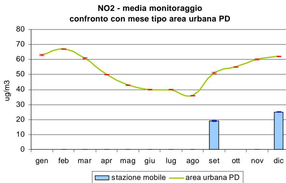
Figura 3.3 Biossido di azoto (NO 2 ): confronto delle concentrazioni medie rilevate durante il monitoraggio in Via Gorne nel Comune di Carceri, con l'andamento caratteristico del 'mese tipo' ricavato dalla serie storica nell'area urbana di Padova; le barre indicano l'errore standard della media.
