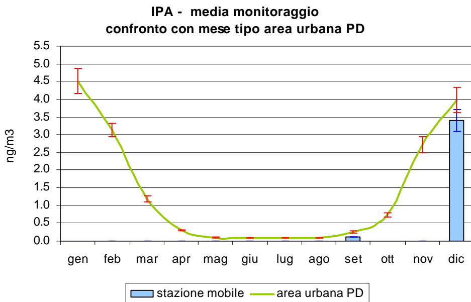
Figura 3.6 Benzo(a)pirene (IPA): confronto delle concentrazioni medie rilevate durante il monitoraggio in Via Gorne nel Comune di Carceri, con l'andamento caratteristico del 'mese tipo' ricavato dalla serie storica nell'area urbana di Padova; le barre indicano l'errore standard della media.
