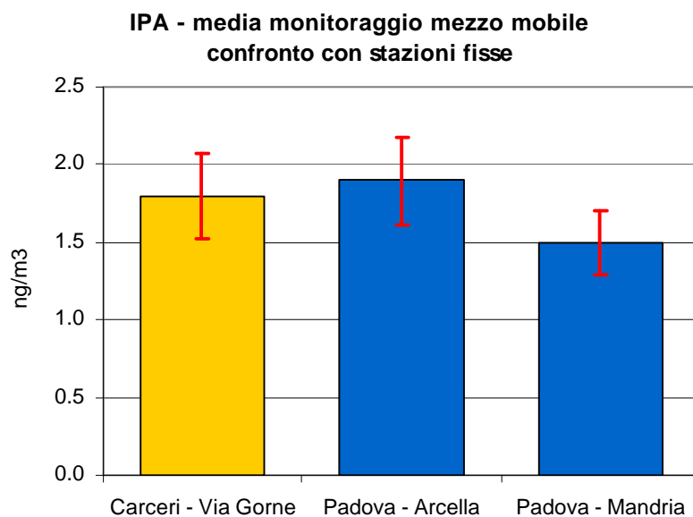
Figura 2.6 Benzo(a)pirene (IPA): concentrazione media rilevata durante il monitoraggio dal 27/08/09 al 14/10/09 e dal 27/11/09 al 18/01/10 in Via Gorne nel Comune di Carceri; le barre indicano l'errore standard della media.
