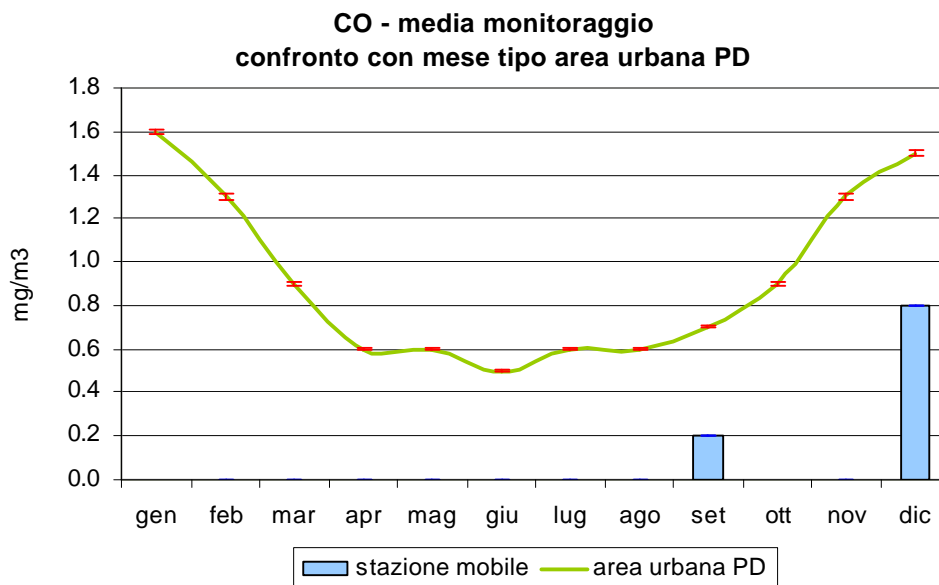
Figura 3.2 Monossido di carbonio (CO): confronto delle concentrazioni medie rilevate durante il monitoraggio in Via Gorne nel Comune di Carceri, con l'andamento caratteristico del 'mese tipo' ricavato dalla serie storica nell'area urbana di Padova; le barre indicano l'errore standard della media.
