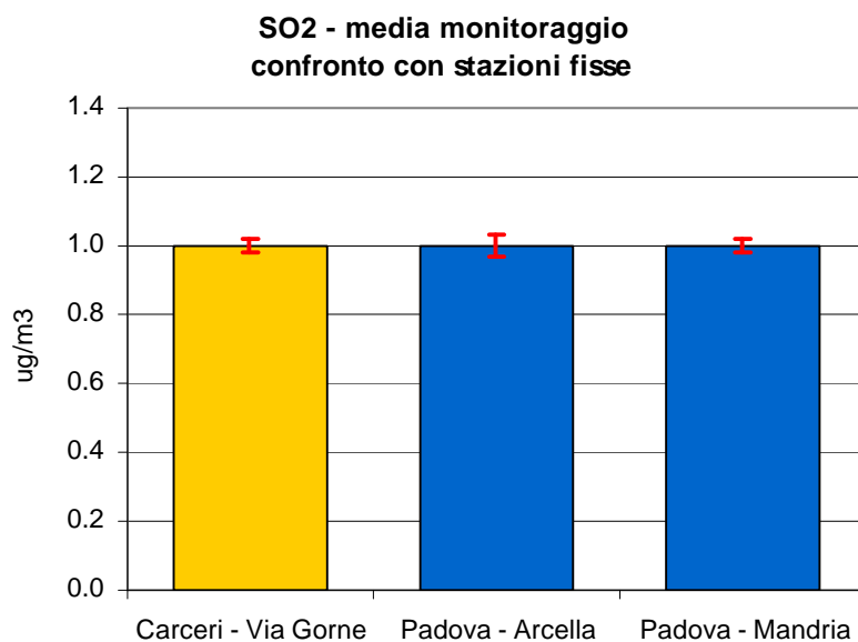
Figura 2.1 Biossido di zolfo (SO 2 ): concentrazione media rilevata durante il monitoraggio dal 27/08/09 al 14/10/09 e dal 27/11/09 al 18/01/10 in Via Gorne nel Comune di Carceri; le barre indicano l'errore standard della media.
