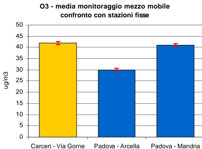
Figura 2.3 Ozono ( O_3 ): concentrazione media rilevata durante il monitoraggio in Via Gorne nel Comune di Carceri; le barre indicano l'errore standard della media.
