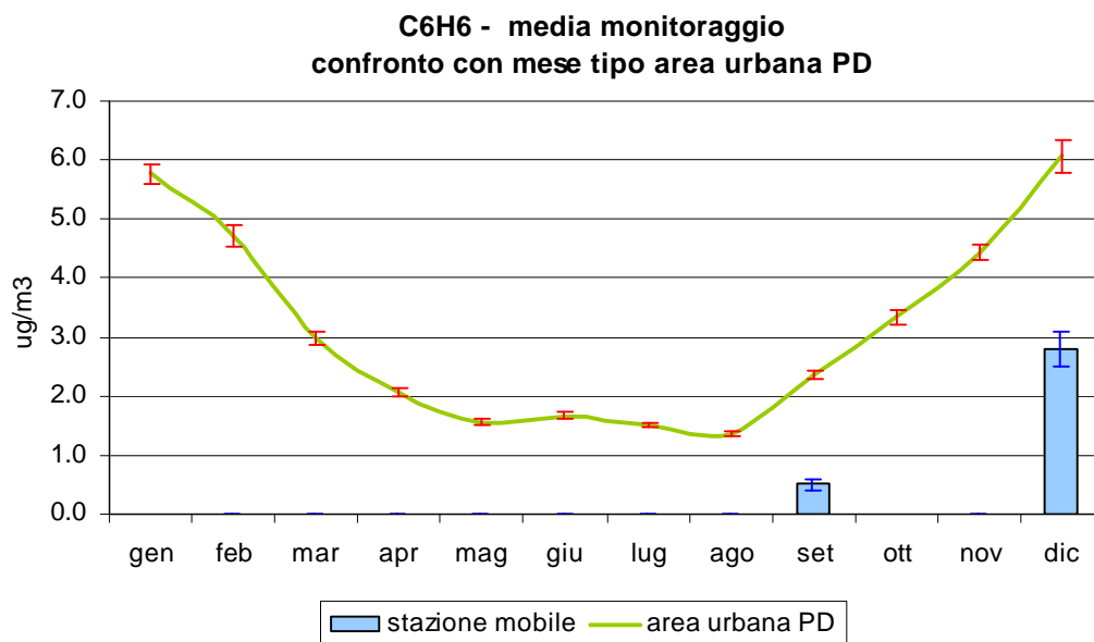
Figura 3.7 Benzene ( C_6H_6 ): confronto delle concentrazioni medie rilevate durante il monitoraggio in Via Gorne nel Comune di Carceri, con l'andamento caratteristico del 'mese tipo' ricavato dalla serie storica nell'area urbana di Padova; le barre indicano l'errore standard della media.
