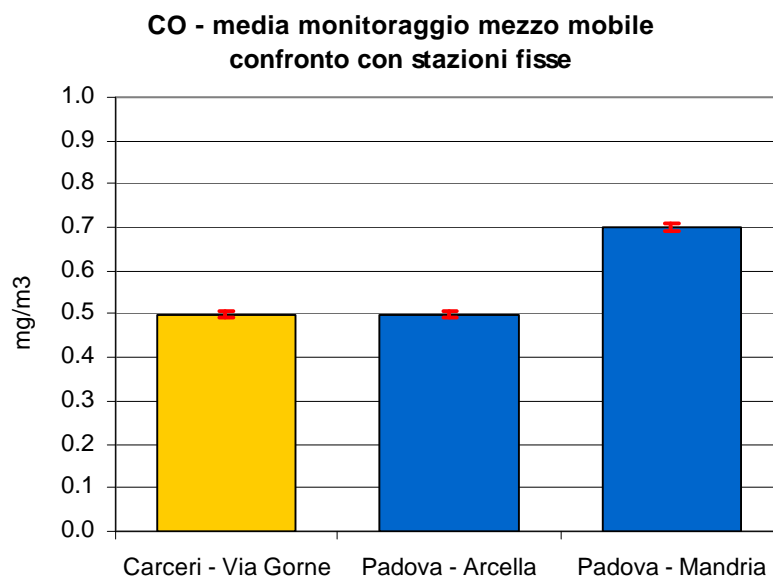
Figura 2.2 Monossido di carbonio (CO): concentrazione media rilevata durante il monitoraggio in Via Gorne nel Comune di Carceri; le barre indicano l'errore standard della media.
