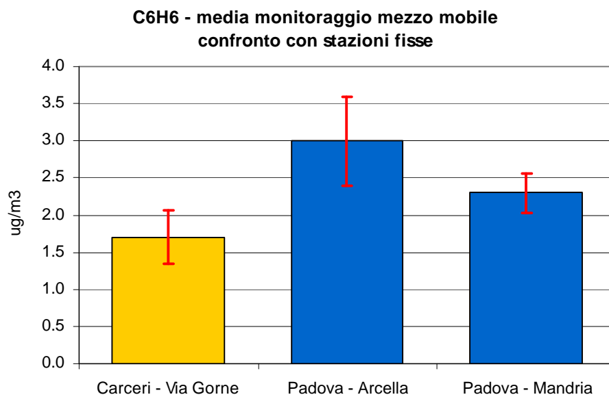
Figura 2.7 Benzene (C 6 H 6 ): concentrazione media rilevata durante il monitoraggio in Via Gorne nel Comune di Carceri; le barre indicano l'errore standard della media.
