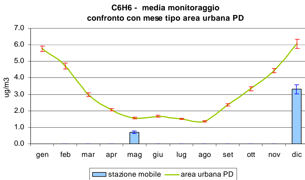
Figura 3.7 Benzene (C 6 H 6 ): confronto delle concentrazioni medie rilevate durante il monitoraggio in Viale dello Sport nel Comune di Cittadella, con l'andamento caratteristico del 'mese tipo' ricavato dalla serie storica nell'area urbana di Padova; le barre indicano l'errore standard della media.
