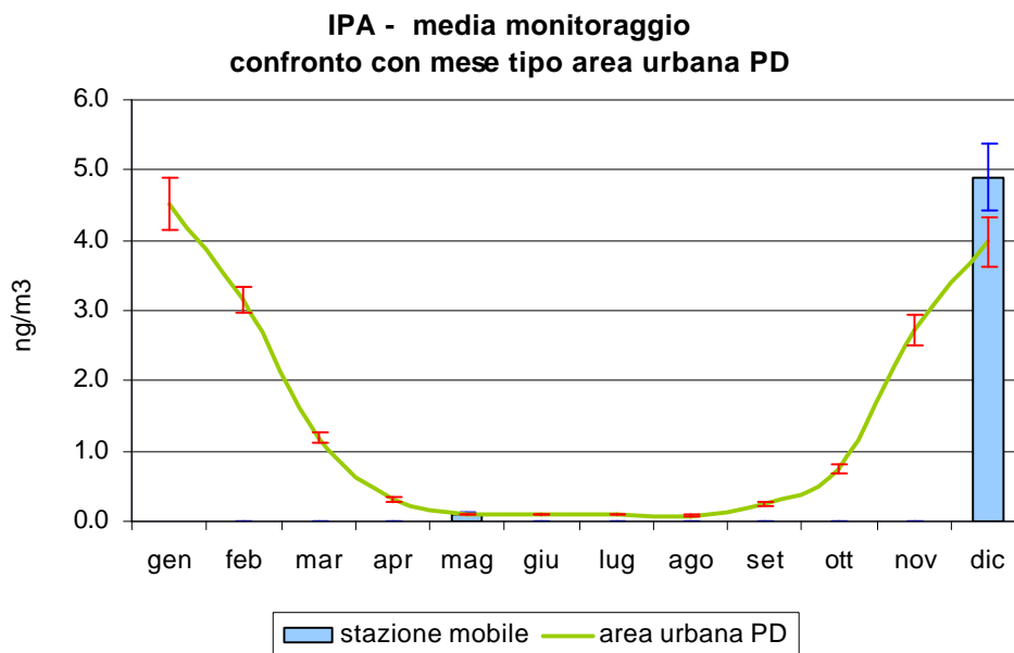
Figura 3.6 Benzo(a)pirene (IPA): confronto delle concentrazioni medie rilevate durante il monitoraggio in Viale dello Sport nel Comune di Cittadella, con l'andamento caratteristico del 'mese tipo' ricavato dalla serie storica nell'area urbana di Padova; le barre indicano l'errore standard della media.
