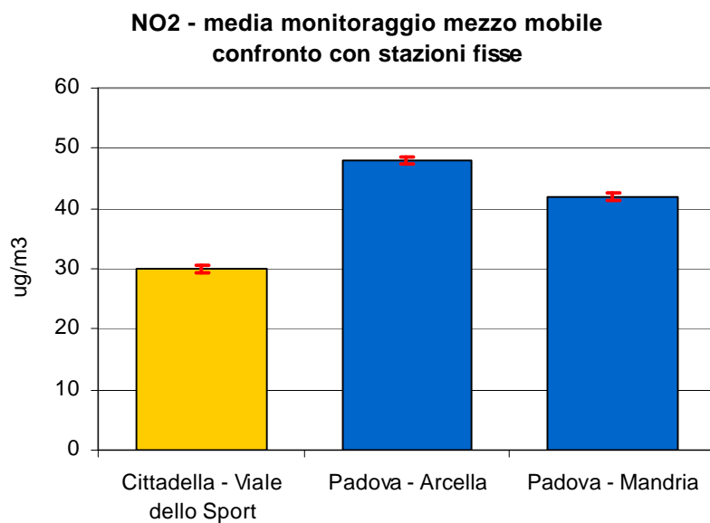
Figura 2.4 Biossido di azoto (NO 2 ): concentrazione media rilevata durante il monitoraggio in Viale dello Sport nel Comune di Cittadella; le barre indicano l'errore standard della media.
