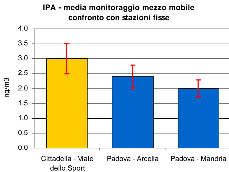
Figura 2.6 Benzo(a)pirene (IPA): concentrazione media rilevata durante il monitoraggio dal 22/04/09 al 18/05/09 e dal 25/11/09 al 04/01/10 in Viale dello Sport nel Comune di Cittadella; le barre indicano l'errore standard della media.
