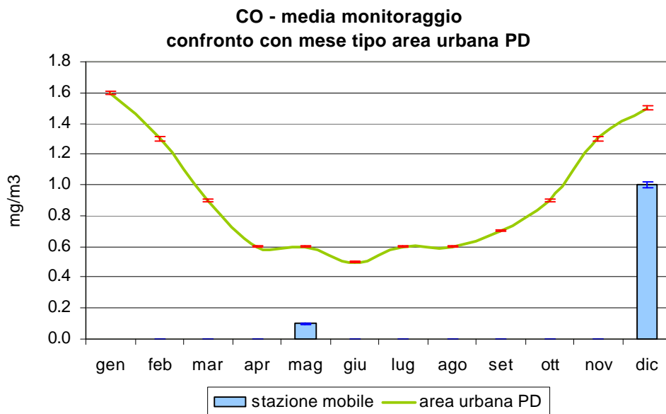
Figura 3.2 Monossido di carbonio (CO): confronto delle concentrazioni medie rilevate durante il monitoraggio in Viale dello Sport nel Comune di Cittadella, con l'andamento caratteristico del 'mese tipo' ricavato dalla serie storica nell'area urbana di Padova; le barre indicano l'errore standard della media.
