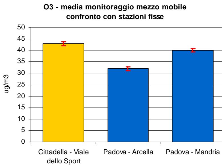
Figura 2.3 Ozono ( O_3 ): concentrazione media rilevata durante il monitoraggio in Viale dello Sport nel Comune di Cittadella; le barre indicano l'errore standard della media.
