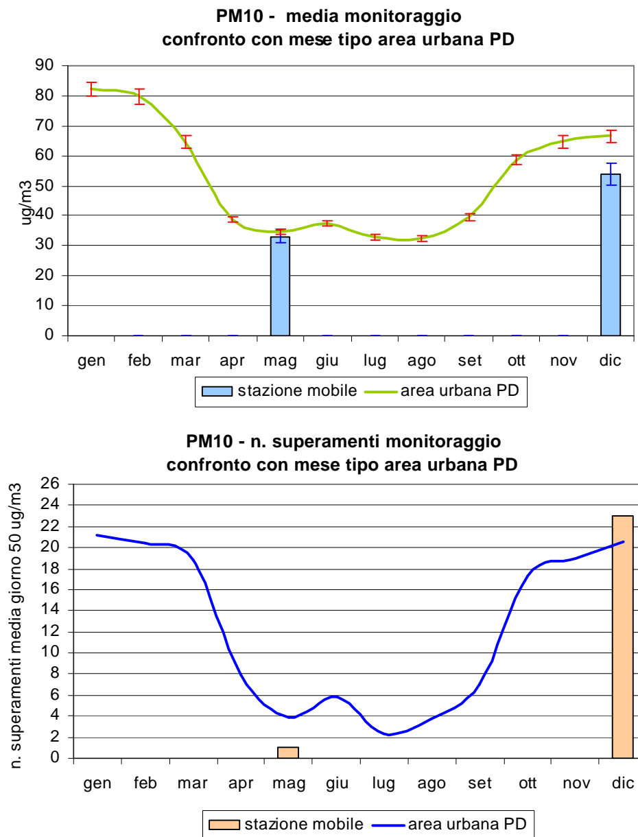
Figura 3.5 Polveri fini ( PM_{10} ): confronto delle concentrazioni medie e del numero di superamenti del valore limite di protezione della salute ( 50 \mu\text{g}/\text{m}^3 ) rilevati durante il monitoraggio in Viale dello Sport nel Comune di Cittadella, con l'andamento caratteristico del 'mese tipo' ricavato dalla serie storica nell'area urbana di Padova; per i valori di concentrazione mensile le barre indicano l'errore standard della media.
