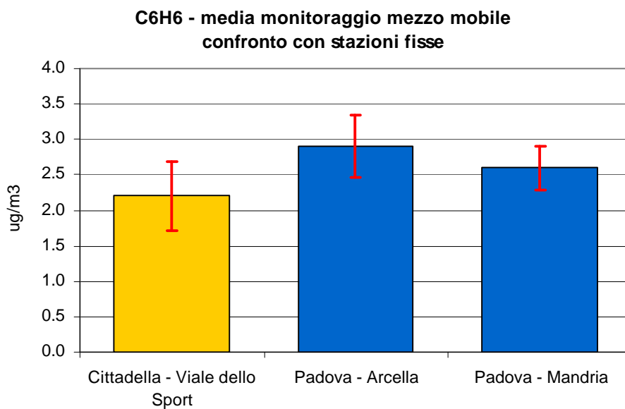
Figura 2.7 Benzene (C 6 H 6 ): concentrazione media rilevata durante il monitoraggio in Viale dello Sport nel Comune di Cittadella; le barre indicano l'errore standard della media.
