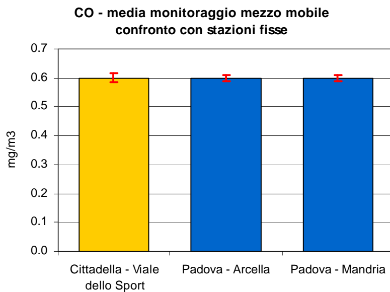
Figura 2.2 Monossido di carbonio (CO): concentrazione media rilevata durante il monitoraggio in Viale dello Sport nel Comune di Cittadella; le barre indicano l'errore standard della media.
