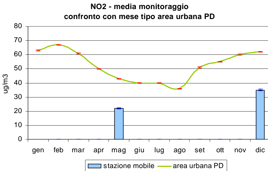
Figura 3.3 Biossido di azoto (NO 2 ): confronto delle concentrazioni medie rilevate durante il monitoraggio in Viale dello Sport nel Comune di Cittadella, con l'andamento caratteristico del 'mese tipo' ricavato dalla serie storica nell'area urbana di Padova; le barre indicano l'errore standard della media.
