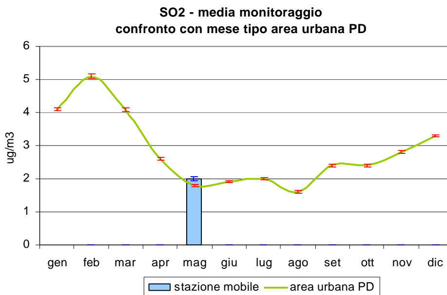
Figura 3.1 Biossido di zolfo (SO 2 ): confronto delle concentrazioni medie rilevate durante il monitoraggio in Viale dello Sport nel Comune di Cittadella, con l'andamento caratteristico del 'mese tipo' ricavato dalla serie storica nell'area urbana di Padova; le barre indicano l'errore standard della media.
