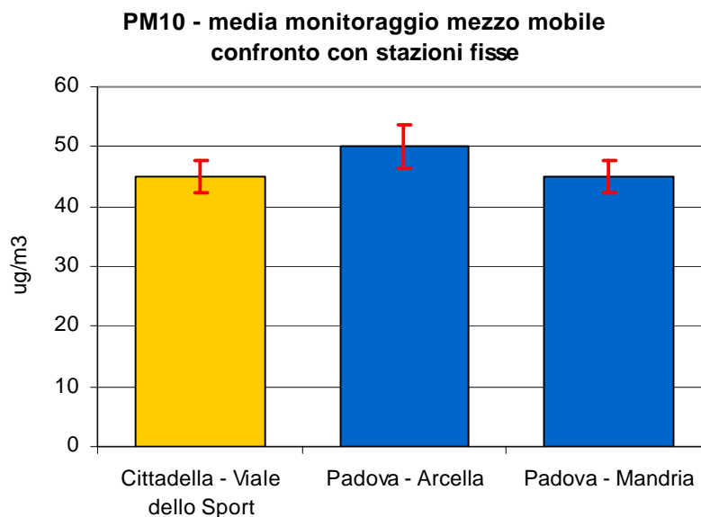
Figura 2.5 Polveri fini (PM 10 ): concentrazione media durante il monitoraggio dal 22/04/09 al 18/05/09 e dal 25/11/09 al 04/01/10 nel Comune di Cittadella; le barre indicano l'errore standard della media.
