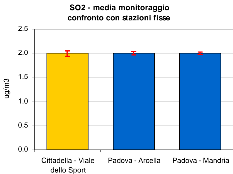
Figura 2.1 Biossido di zolfo (SO 2 ): concentrazione media rilevata durante il monitoraggio dal 22/04/09 al 18/05/09 in Viale dello Sport nel Comune di Cittadella; le barre indicano l'errore standard della media.
