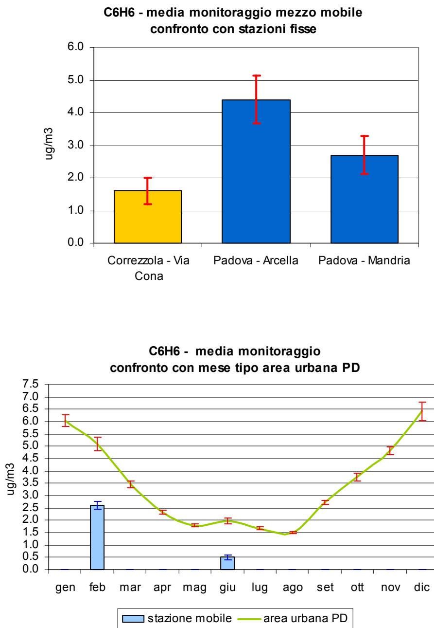
Figura 2.7 Benzene (C 6 H 6 ): concentrazione media rilevata durante il monitoraggio dal 30/01/08 al 27/02/08 e dal 01/05/08 al 04/06/08 in Via Cona nel Comune di Correzzola; confronto con i periodi corrispondenti presso le stazioni fisse di Arcella e Mandria nel Comune di Padova e con l'andamento caratteristico del 'mese tipo' ricavato dalla serie storica nell'area urbana di Padova; le barre indicano l'errore standard della media.
