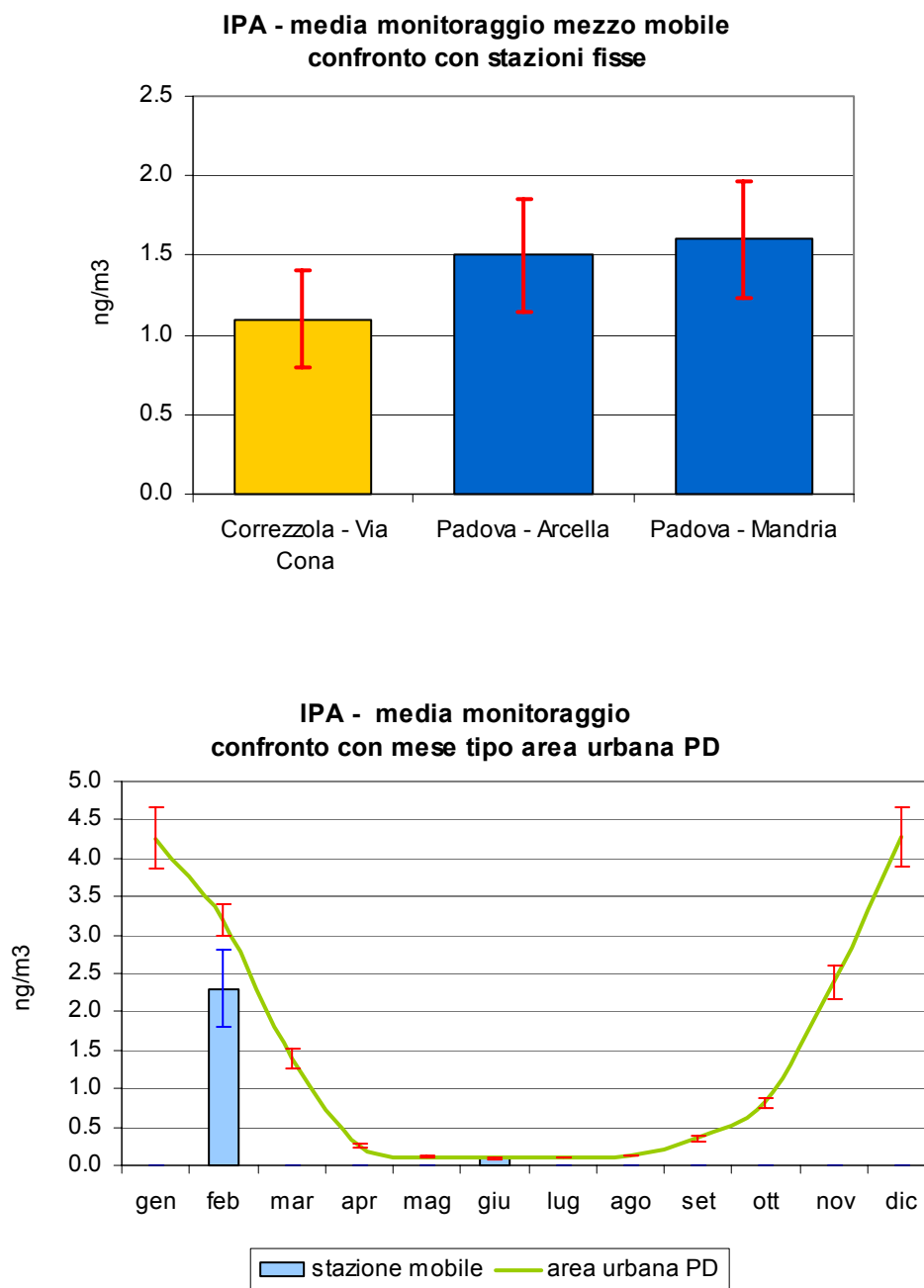
Figura 2.6 Benzo(a)pirene (IPA): concentrazione media rilevata durante il monitoraggio dal 30/01/08 al 27/02/08 e dal 01/05/08 al 04/06/08 in Via Cona nel Comune di Correzzola; confronto con i periodi corrispondenti presso le stazioni fisse di Arcella e Mandria nel Comune di Padova e con l'andamento caratteristico del 'mese tipo' ricavato dalla serie storica nell'area urbana di Padova; le barre indicano l'errore standard della media.
