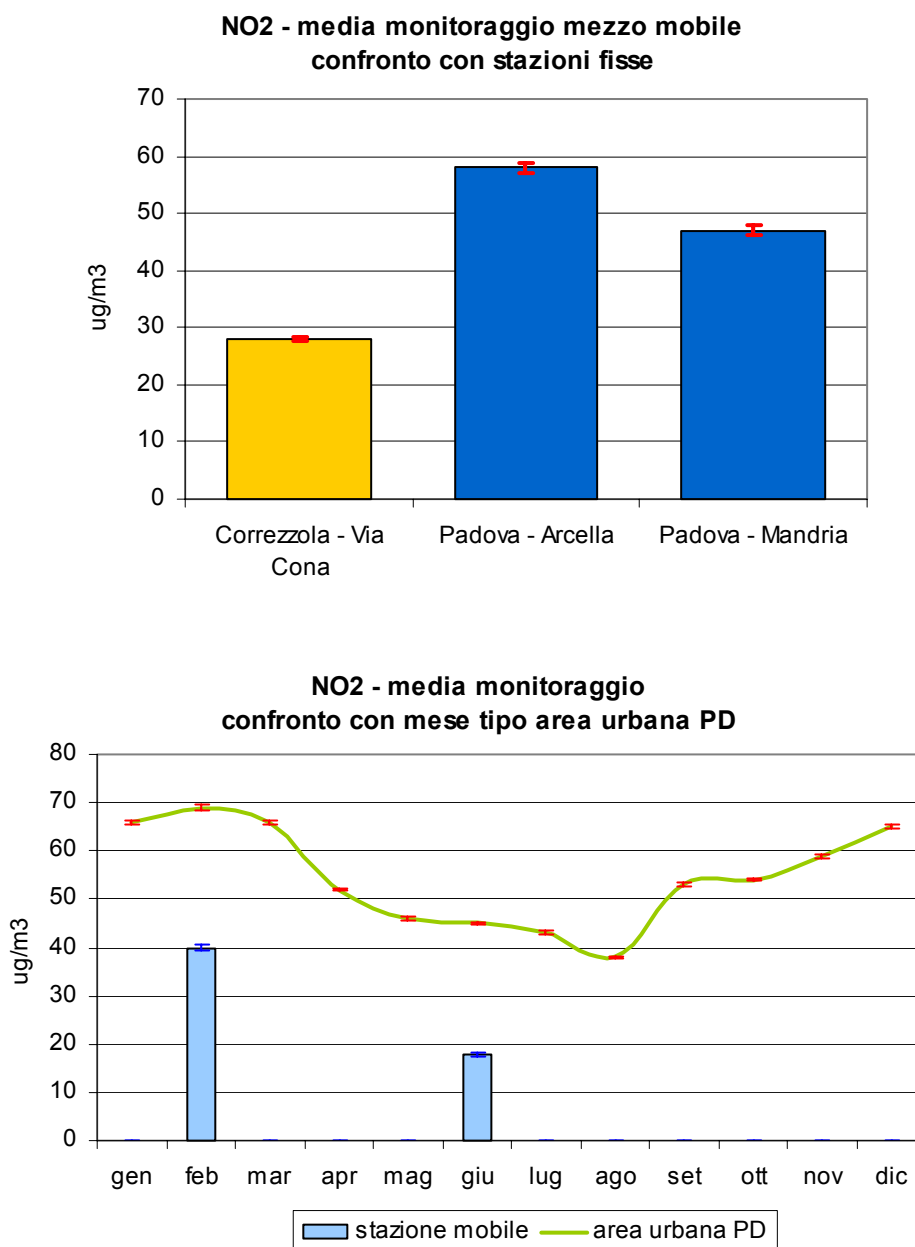
Figura 2.4 Biossido di azoto ( \text{NO}_2 ): concentrazione media rilevata durante il monitoraggio dal 30/01/08 al 27/02/08 e dal 01/05/08 al 04/06/08 in Via Cona nel Comune di Correzzola; confronto con i periodi corrispondenti presso le stazioni fisse di Arcella e Mandria nel Comune di Padova e con l'andamento caratteristico del 'mese tipo' ricavato dalla serie storica nell'area urbana di Padova; le barre indicano l'errore standard della media.
