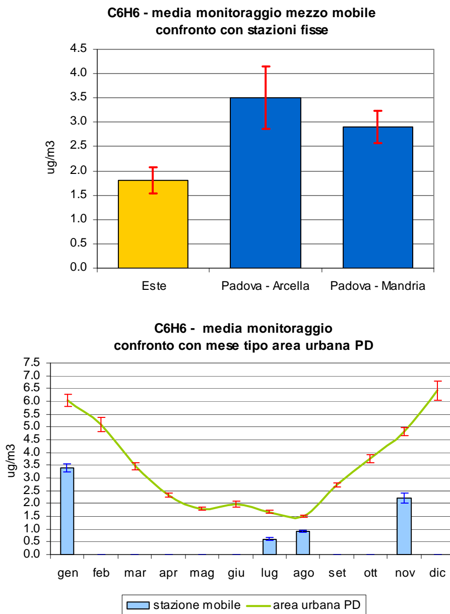
Figura 2.7 Benzene (C 6 H 6 ): concentrazione media rilevata durante il monitoraggio nel Comune di Este; confronto con i periodi corrispondenti presso le stazioni fisse di Arcella e Mandria nel Comune di Padova e con l'andamento caratteristico del 'mese tipo' ricavato dalla serie storica nell'area urbana di Padova; le barre indicano l'errore standard della media.
