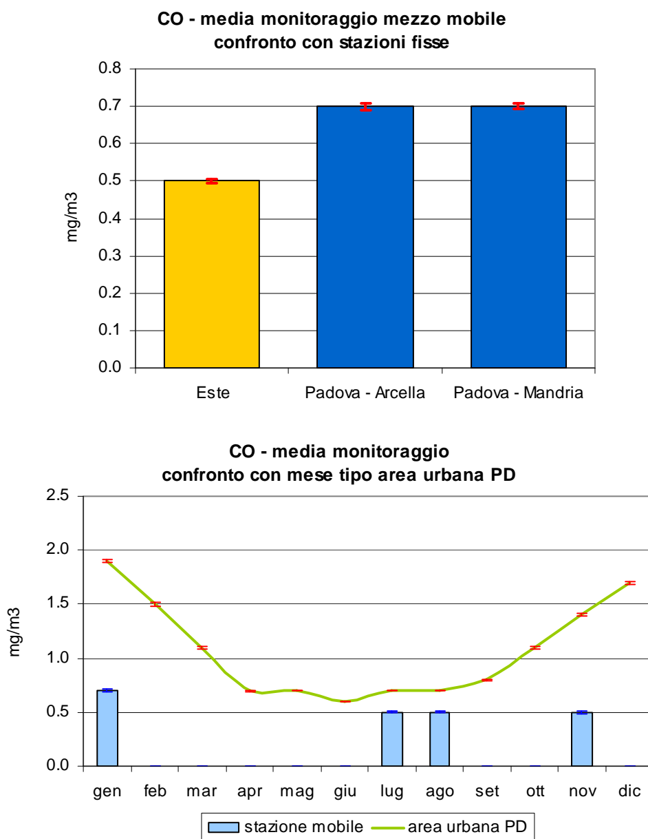
Figura 2.2 Monossido di carbonio (CO): concentrazione media rilevata durante il monitoraggio nel Comune di Este; confronto con i periodi corrispondenti presso le stazioni fisse di Arcella e di Mandria nel Comune di Padova e con l'andamento caratteristico del 'mese tipo' ricavato dalla serie storica nell'area urbana di Padova; le barre indicano l'errore standard della media.
