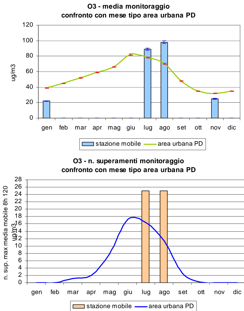
Figura 2.3 Ozono (O 3 ): concentrazione media e numero di superamenti rilevati durante il monitoraggio nel Comune di Este; confronto con i periodi corrispondenti presso le stazioni fisse di Arcella e di Mandria nel Comune di Padova e con l'andamento caratteristico del 'mese tipo' ricavato dalla serie storica nell'area urbana di Padova; per i valori di concentrazione mensile le barre indicano l'errore standard della media.
