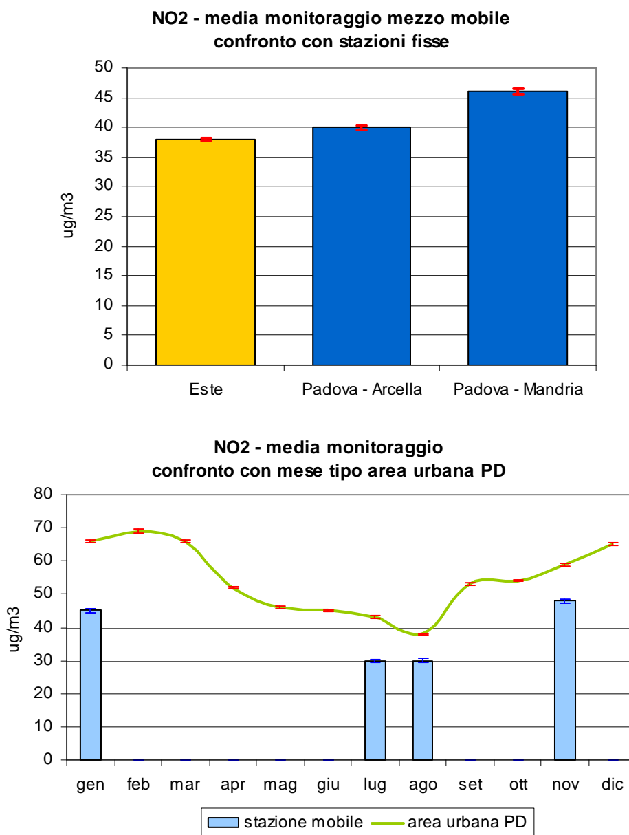
Figura 2.4 Biossido di azoto ( \text{NO}_2 ): concentrazione media rilevata durante il monitoraggio nel Comune di Este; confronto con i periodi corrispondenti presso le stazioni fisse di Arcella e Mandria nel Comune di Padova e con l'andamento caratteristico del 'mese tipo' ricavato dalla serie storica nell'area urbana di Padova; le barre indicano l'errore standard della media.
