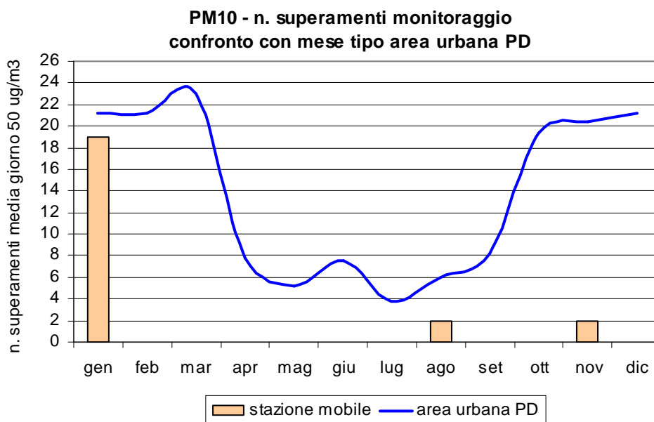
Figura 2.5 Polveri fini (PM 10 ): concentrazione media e numero di superamenti rilevati durante il monitoraggio nel Comune di Este; confronto con i periodi corrispondenti presso le stazioni fisse di Arcella e Mandria nel Comune di Padova e con l'andamento caratteristico del 'mese tipo' ricavato dalla serie storica nell'area urbana di Padova; per i valori di concentrazione mensile le barre indicano l'errore standard della media.
