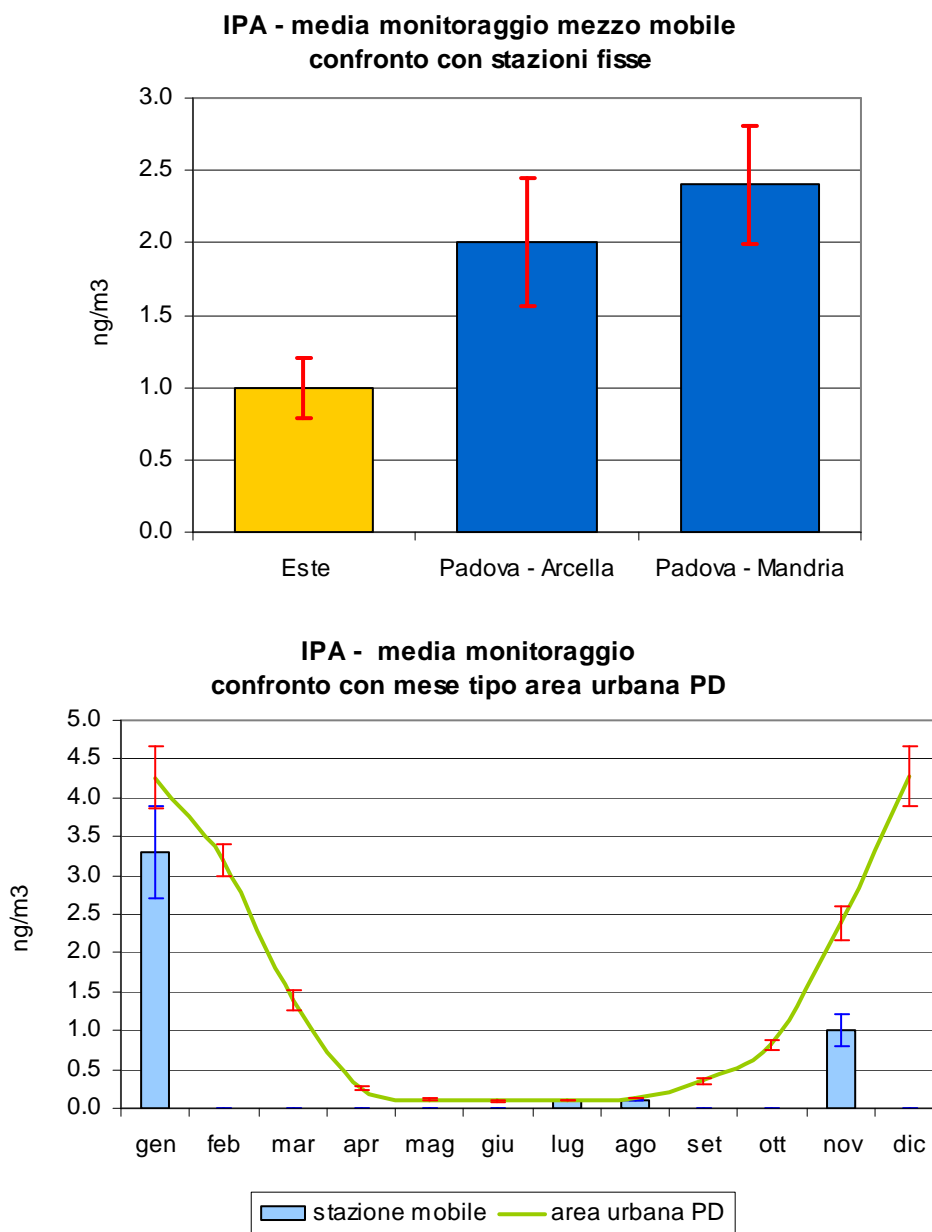
Figura 2.6 Benzo(a)pirene (IPA): concentrazione media rilevata durante il monitoraggio nel Comune di Este; confronto con i periodi corrispondenti presso le stazioni fisse di Arcella e Mandria nel Comune di Padova e con l'andamento caratteristico del 'mese tipo' ricavato dalla serie storica nell'area urbana di Padova; le barre indicano l'errore standard della media.
