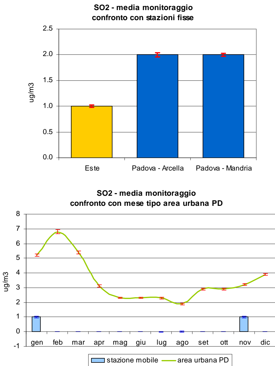
Figura 2.1 Biossido di zolfo ( \text{SO}_2 ): concentrazione media rilevata durante il monitoraggio nel Comune di Este; confronto con i periodi corrispondenti presso le stazioni fisse di Arcella e Mandria nel Comune di Padova e con l'andamento caratteristico del 'mese tipo' ricavato dalla serie storica nell'area urbana di Padova; le barre indicano l'errore standard della media.
