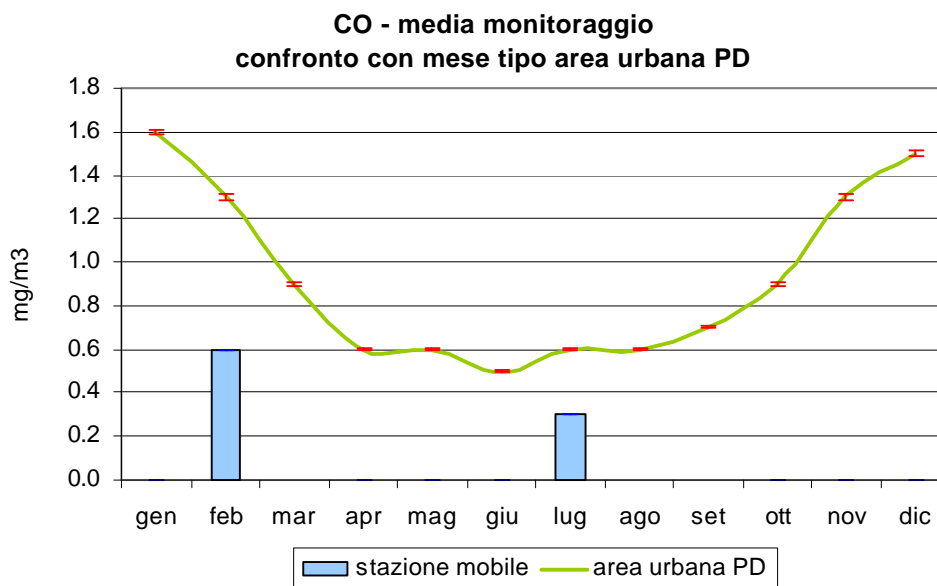
Figura 3.1 Monossido di carbonio (CO): confronto delle concentrazioni medie rilevate durante il monitoraggio in Via G. Marconi nel Comune di Megliadino San Fidenzio, con l’andamento caratteristico del ‘mese tipo’ ricavato dalla serie storica nell’area urbana di Padova; le barre indicano l’errore standard della media.
