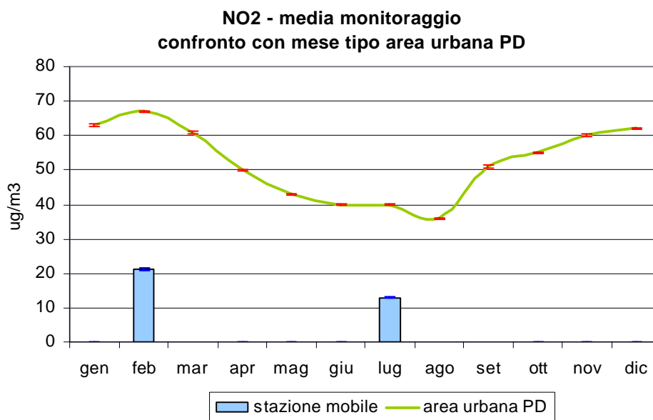
Figura 3.3 Biossido di azoto ( NO_2 ): confronto delle concentrazioni medie rilevate durante il monitoraggio in Via G. Marconi nel Comune di Megliadino San Fidenzio, con l'andamento caratteristico del 'mese tipo' ricavato dalla serie storica nell'area urbana di Padova; le barre indicano l'errore standard della media.
