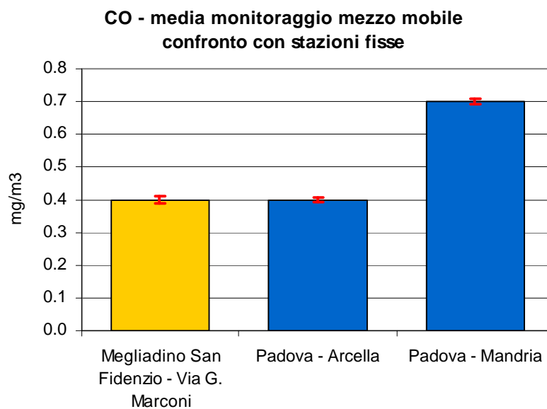
Figura 2.1 Monossido di carbonio (CO): concentrazione media rilevata durante il monitoraggio dal 11/02/09 al 17/03/09 e dal 13/06/09 al 02/09/09 in Via G. Marconi nel Comune di Megliadino San Fidenzio, e confronto con i periodi corrispondenti presso le stazioni fisse di Arcella e Mandria; le barre indicano l'errore standard della media.
