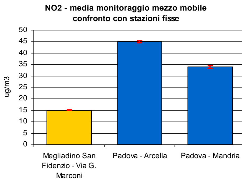
Figura 2.3 Biossido di azoto (NO 2 ): concentrazione media rilevata durante il monitoraggio dal 11/02/09 al 17/03/09 e dal 13/06/09 al 02/09/09 in Via G. Marconi nel Comune di Megliadino San Fidenzio, e confronto con i periodi corrispondenti presso le stazioni fisse di Arcella e Mandria; le barre indicano l'errore standard della media.
