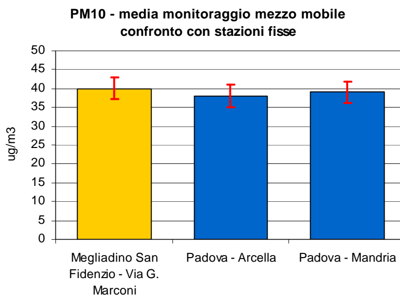
Figura 2.4 Polveri fini ( PM_{10} ): concentrazione media durante il monitoraggio dal 11/02/09 al 17/03/09 e dal 13/06/09 al 02/09/09 nel Comune di Megliadino San Fidenzio e confronto con i periodi corrispondenti presso le stazioni fisse di Arcella e Mandria; le barre indicano l'errore standard della media.
